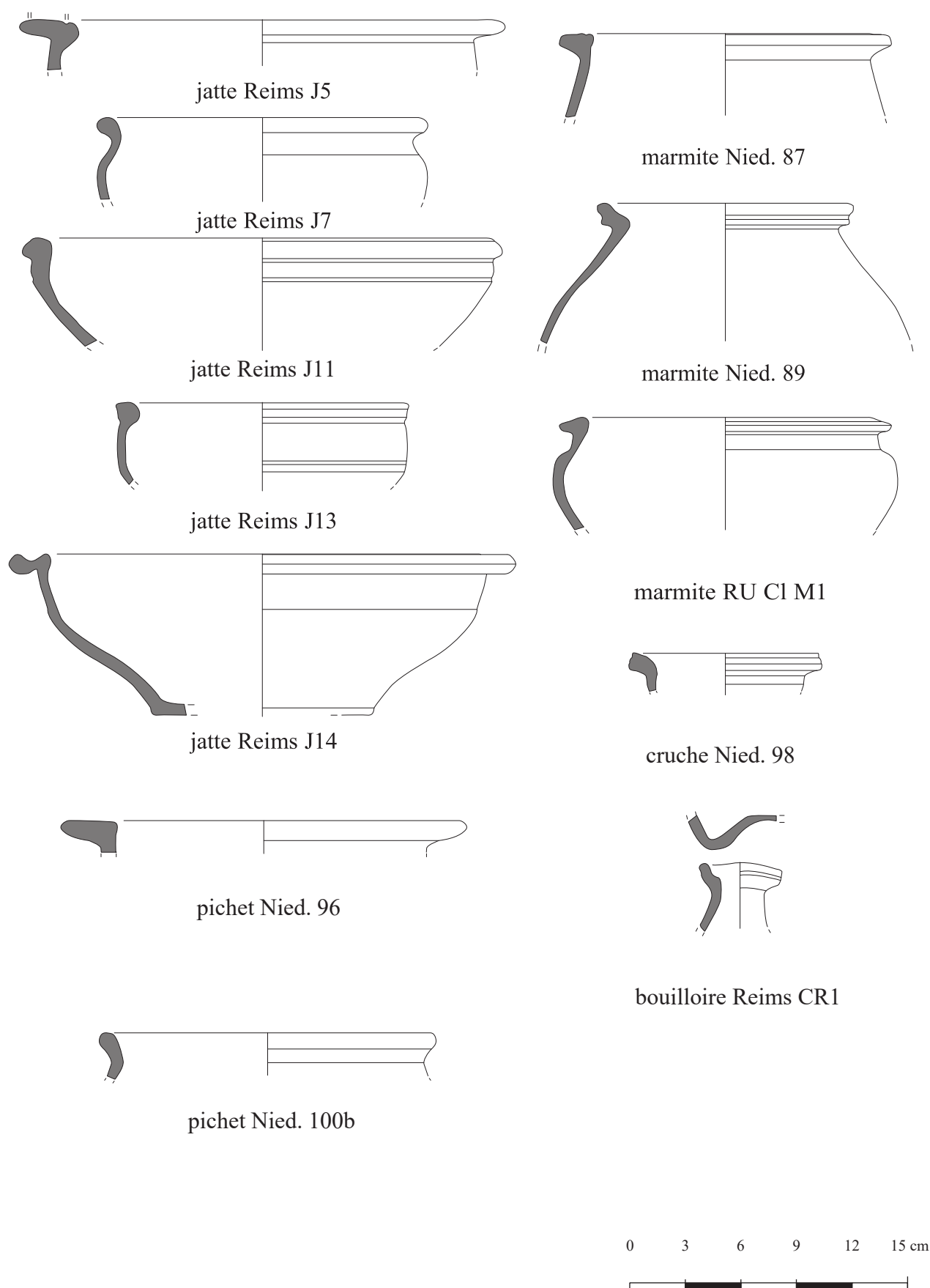
Fig. 152 Planche typologique des jattes, marmites, cruche, pichets et bouilloire en céramique rugueuse.
