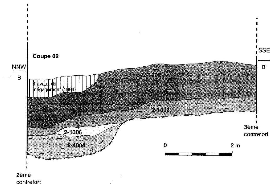
Fig. 59 Relevé de la coupe 02 (Milutinovic Feller 1997 p. 20 fig. 12).
