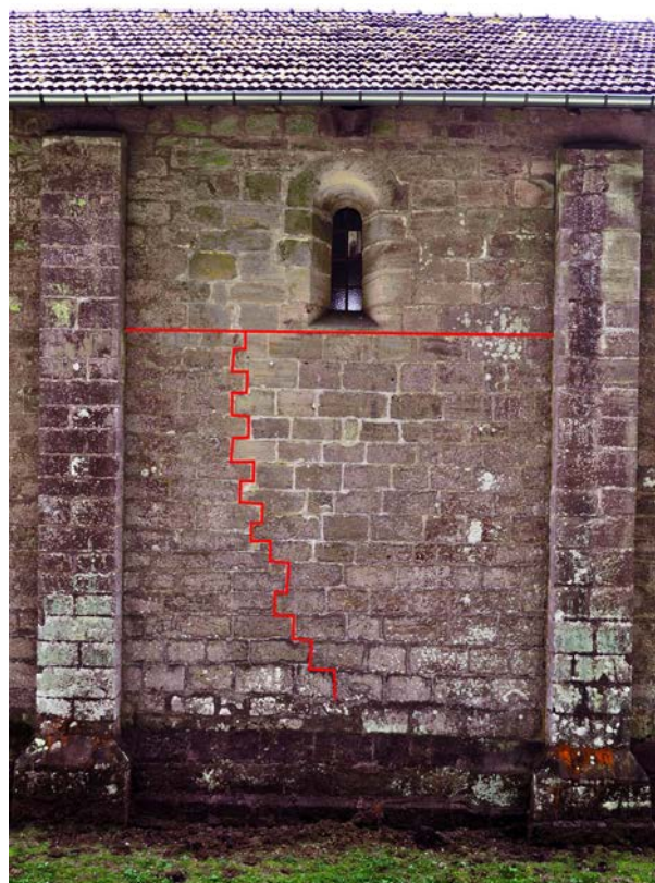
Fig. 42 – Couture sur la troisième travée nord de l'abbatiale de Droiteval, 88 (cliché Cédric Moulis).
