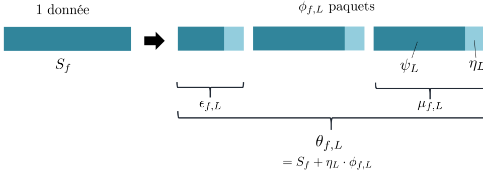
FIGURE 2.5 – Modèle de fragmentation
