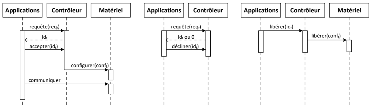
FIGURE 2.17 – Diagrammes de séquence des interfaces contrôleur/applications et contrôleur/matériel
