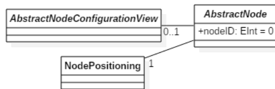
FIGURE 5.18 – Modèle UML des fonctionnalités optionnelles spécifiques aux nœuds
