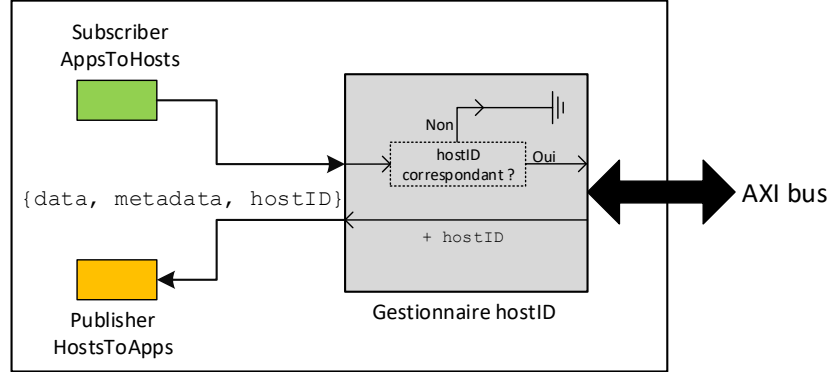
FIGURE 5.9 – Acteur EricaHostPart
