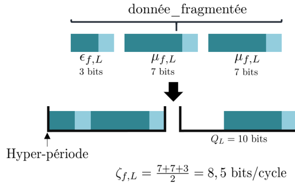
FIGURE 2.10 – Illustration du calcul de la bande passante offerte maximale
