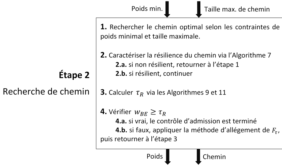
FIGURE 3.11 – Extension de l'étape de recherche de chemin lors du contrôle d'admission
