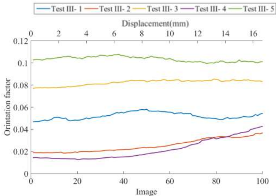
Fig 5 Facteurs d'orientation des tests de laboratoire
