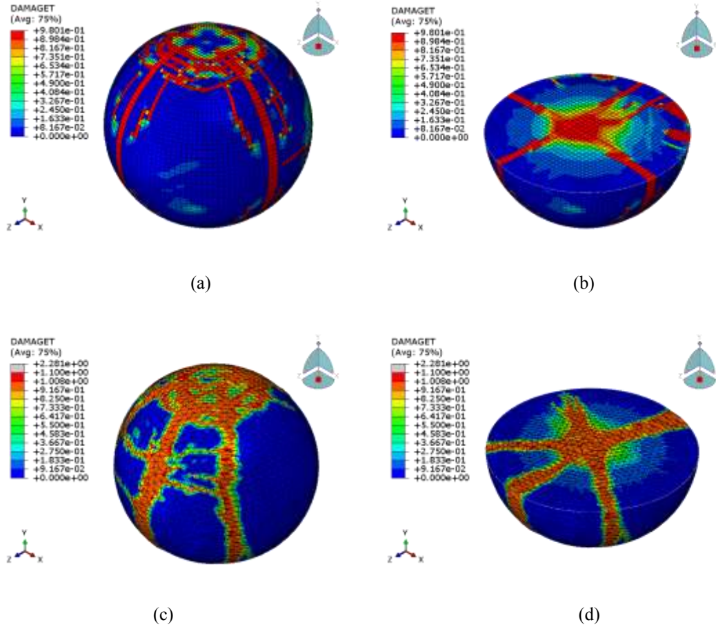
(a)(b) État d'échec de Model 1-1. (c)(d) État d'échec de Model 1-2
