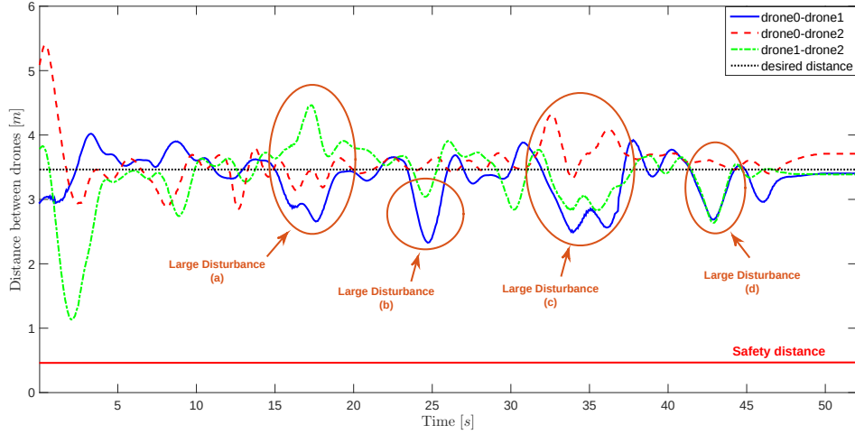
FIGURE 4.19 – Distances entre agents en temps réel en présence d'importantes perturbations. cible mobile.
