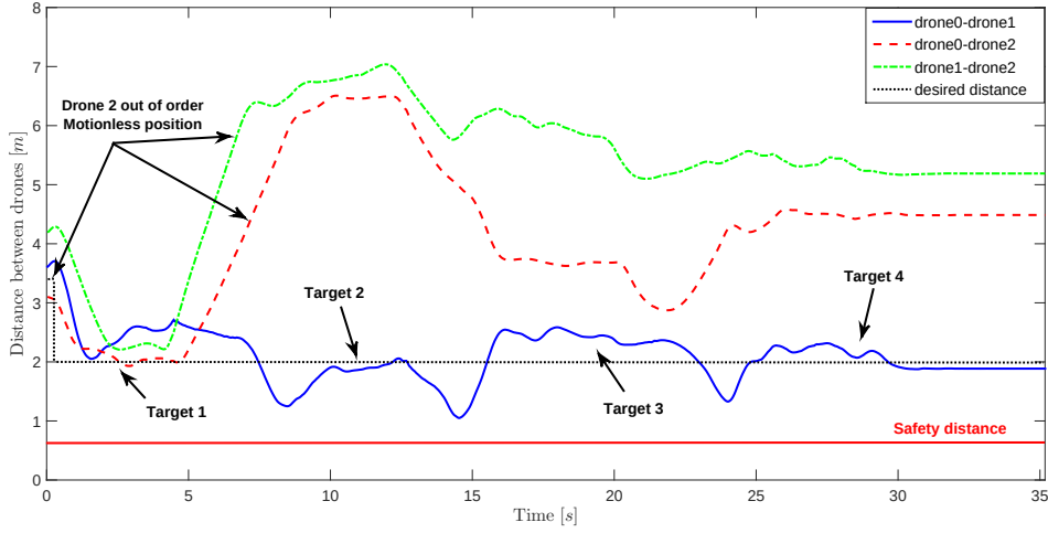
FIGURE 4.24 – Distances entre les UAVs dans le cas d'une défaillance d'un agent.
