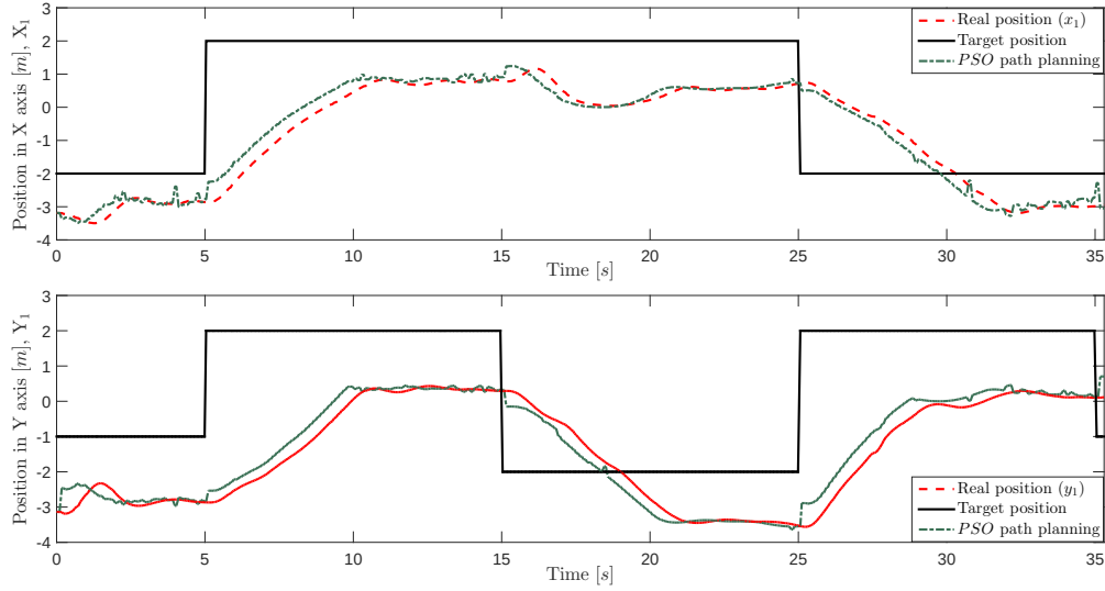
FIGURE 3.17 – Trajectoire calculée et réelle du premier quadrirotor sur les axes x et y
