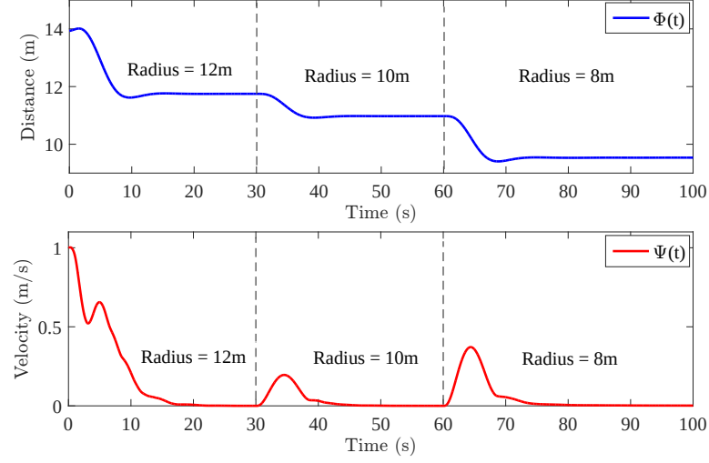
FIGURE 2.17 – La distance moyenne et les différences de vitesse entre les UAVs
