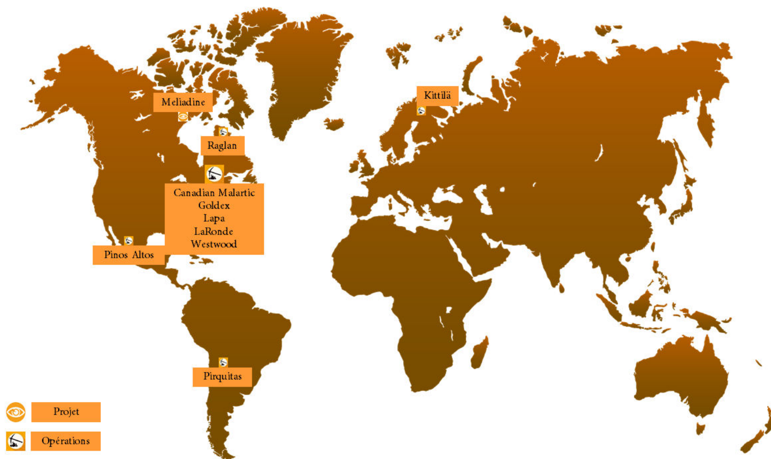
Figure 4.1 Localisation des dix minerais étudiés dans la thèse
