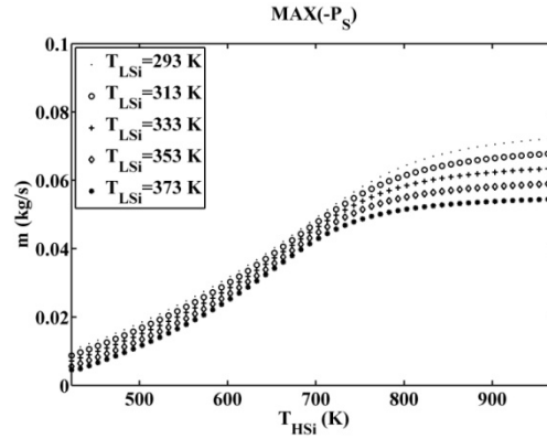
Figure 48 : Débit massique du fluide cyclé dans le cas de la maximisation de la puissance du système en fonction la température du fluide chaud en entrée de système pour différentes valeurs de la température du fluide froid
