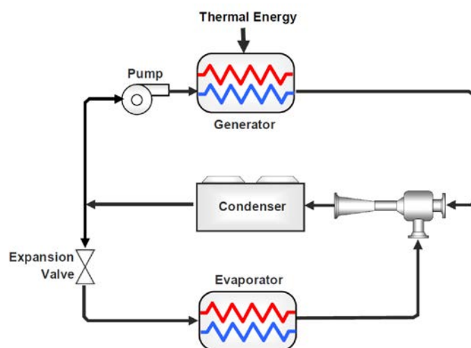
Figure 28 : Schéma d'un éjecteur [77]
