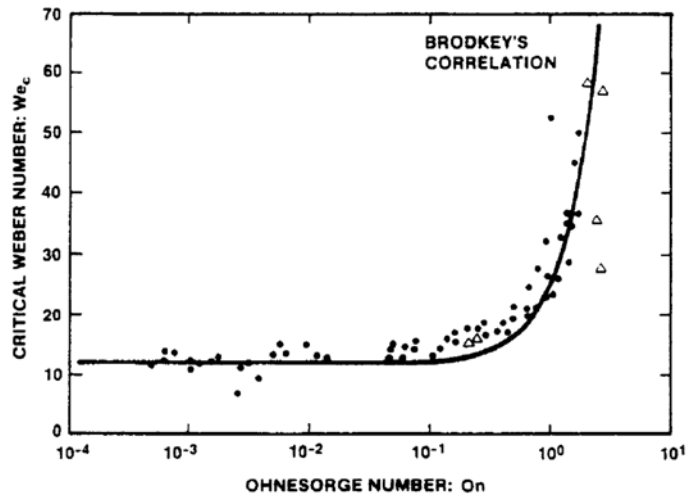
Figure 80 : Nombre de Weber critique: • données expérimentales pour un gaz et un liquide ([133], [131], [132], [134] et [135]); Δ données expérimentales pour deux liquides [136].
