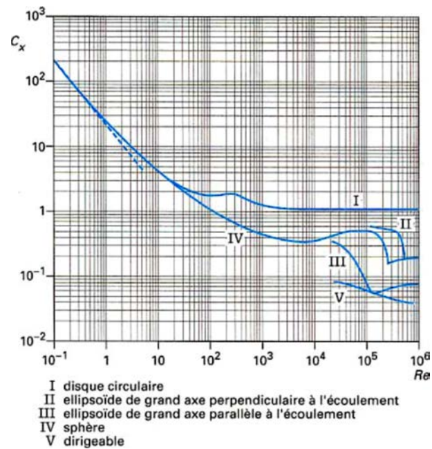
Figure 87 : Coefficient de trainée pour différents obstacles en fonction du nombre de Reynolds [145]
