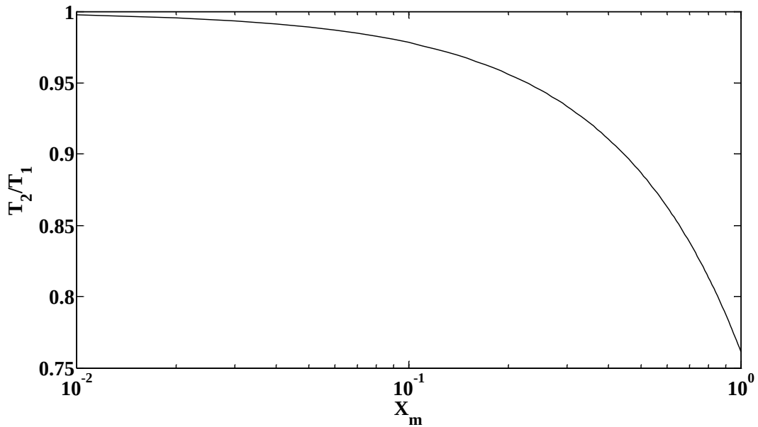
Figure 75 : Evolution du rapport de température entre le début et la fin de la détente en fonction du titre dynamique massique en eau ( P_1/P_2 = 13 )
