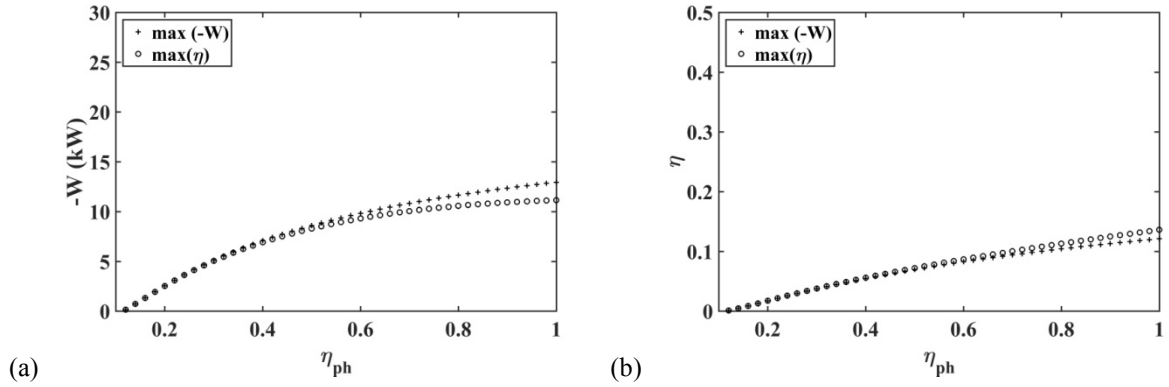
Figure 134 : (a) Puissance produite et (b) rendement; en fonction du rendement de la pompe à huile dans le cas de la maximisation de la puissance et de la maximisation du rendement
