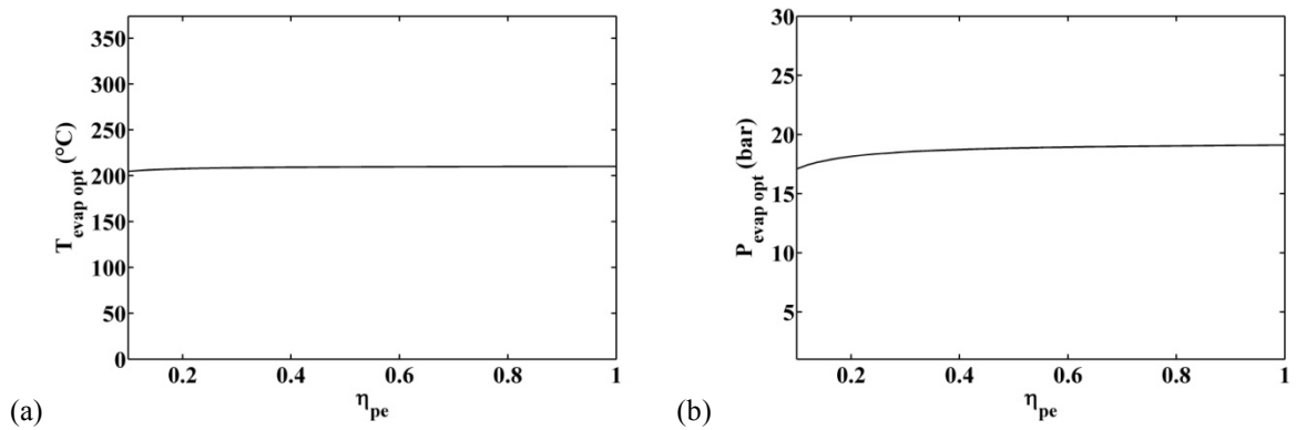
Figure 158 : (a) Température optimale de vaporisation de l'eau et (b) pression optimale de vaporisation de l'eau; en fonction du rendement de la pompe à eau dans le cas de la maximisation de la puissance avec surchauffe de la vapeur
