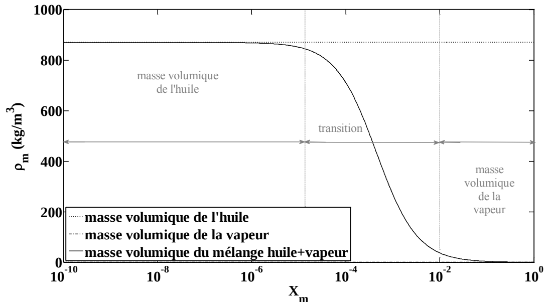
Figure 73 : Masse volumique du mélange huile/vapeur en fonction du titre massique en vapeur X_m ( p = 1 bar, T = 300 °C)
