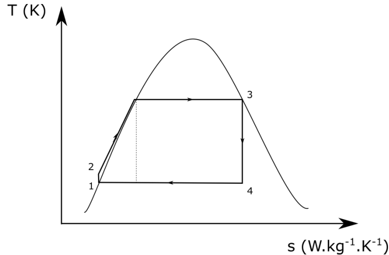
Figure 16 : Cycle de Rankine dans le diagramme entropique
