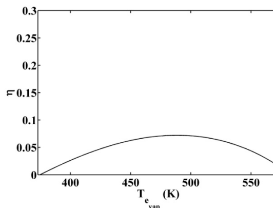
Figure 113 : Rendement au sens du premier principe en fonction de la température de vaporisation de l'eau
