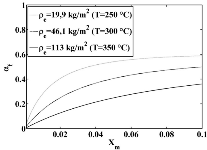
Figure 83 : Taux de vide, dans le cas d'un écoulement dispersé d'huile et de vapeur d'eau, sans dissipations, en fonction du titre dynamique massique en eau, et pour différentes valeurs de la masse volumique de la vapeur d'eau
