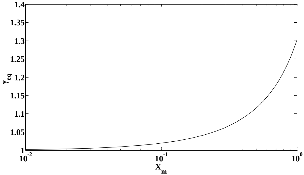
Figure 74 : Evolution du coefficient de détente isentropique en fonction du titre dynamique massique en eau ( T = 300 °C).
