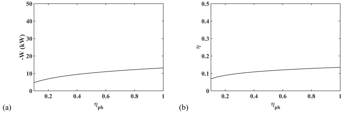
Figure 157 : (a) Puissance produite et (b) rendement; en fonction du rendement de la pompe à huile dans le cas de la maximisation de la puissance avec surchauffe de la vapeur
