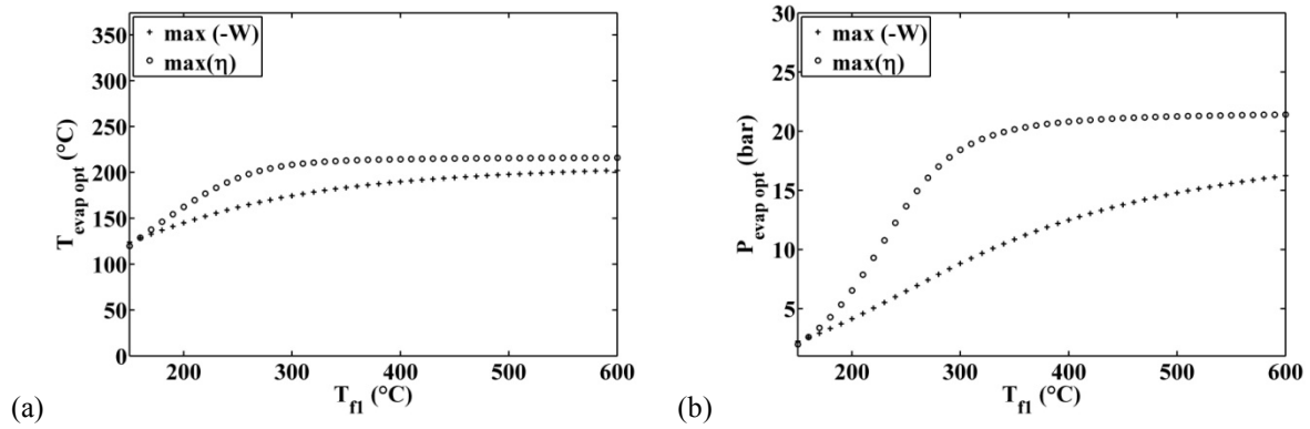
Figure 124 : (a) Température optimale de vaporisation de l'eau et (b) pression optimale de vaporisation de l'eau ; en fonction de la température de la fumée disponible dans le cas de la maximisation de la puissance et de la maximisation du rendement
