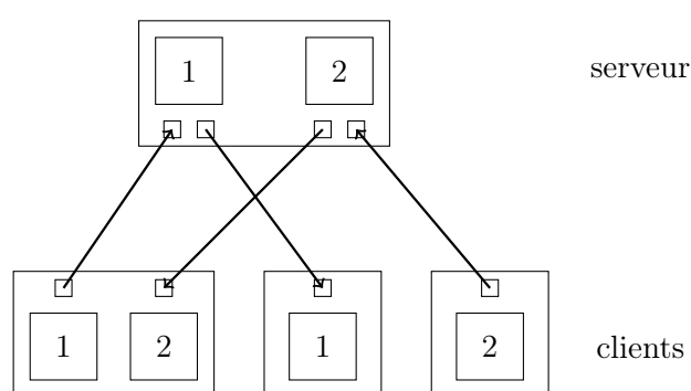
FIGURE 5.19 – Exemple de liens websockets clients-serveur
