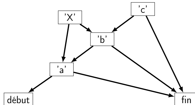
FIGURE 3.12 – Exemple de document WOOT
