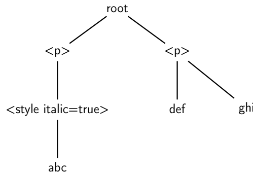
FIGURE 4.1 – Exemple de modèle de document
