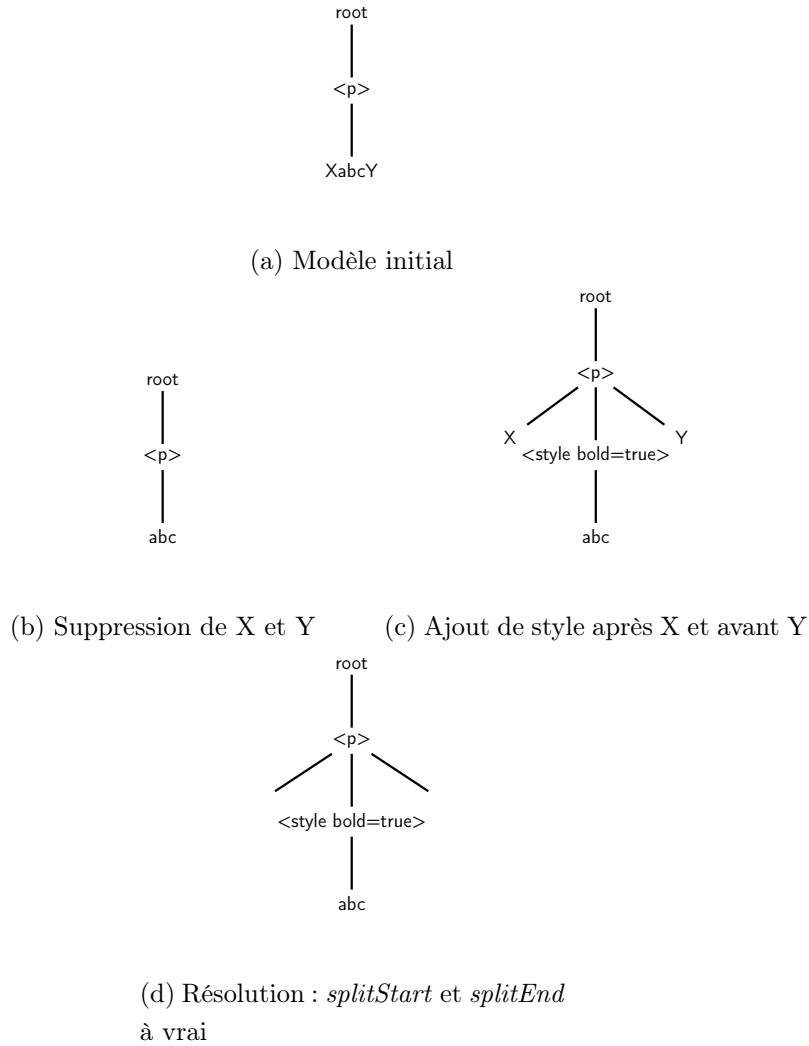
FIGURE 4.6 – Suppression et style en bordure de feuille
