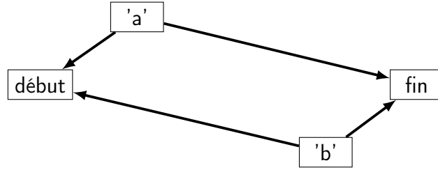
FIGURE 3.13 – Insertions concurrentes simples avec WOOT
