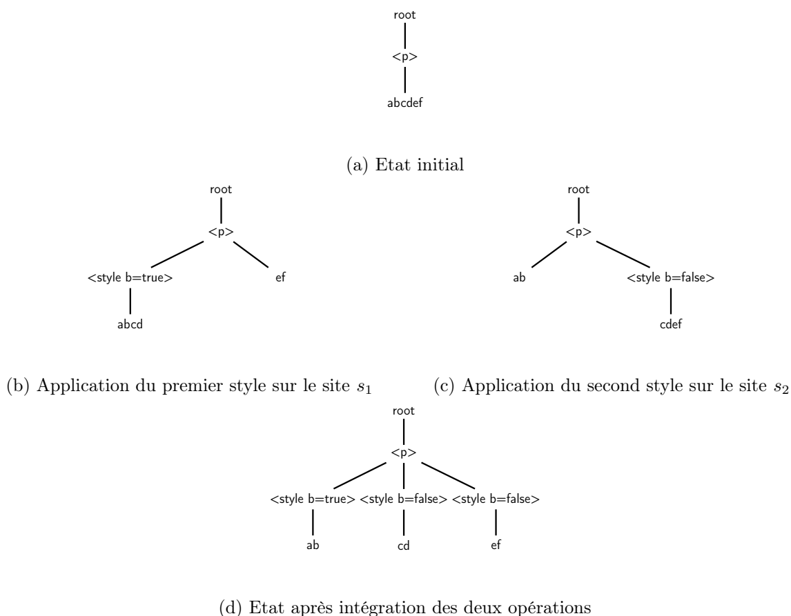
FIGURE 4.8 – Intégration de deux opérations Style concurrentes
