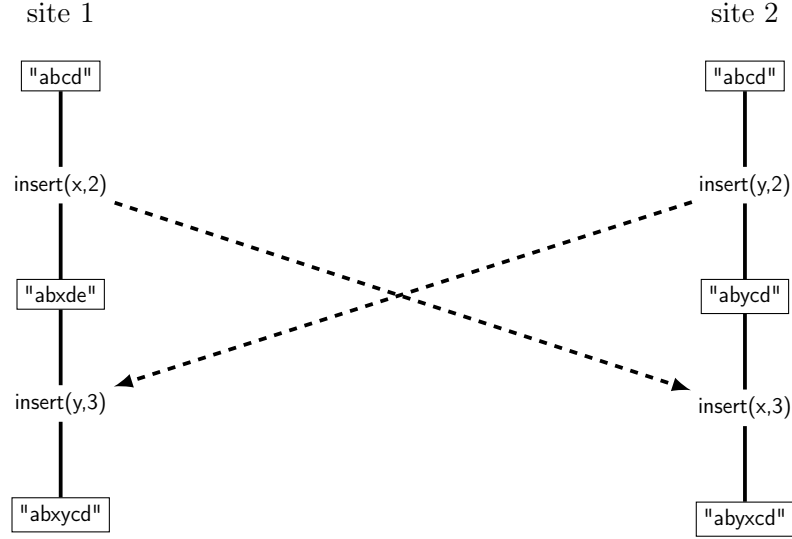
FIGURE 3.3 – Divergence avec respect des intentions
