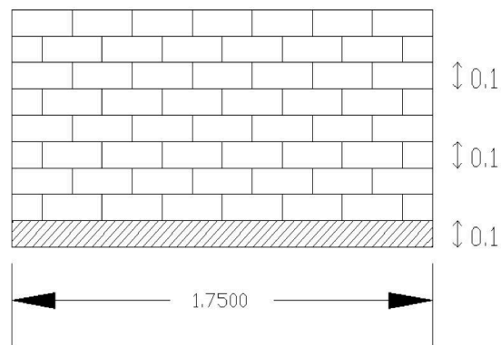
Figure 101 : Géométrie des murs en maçonnerie testés dans l'essai de flexion et illustration de la manutention du mur.
