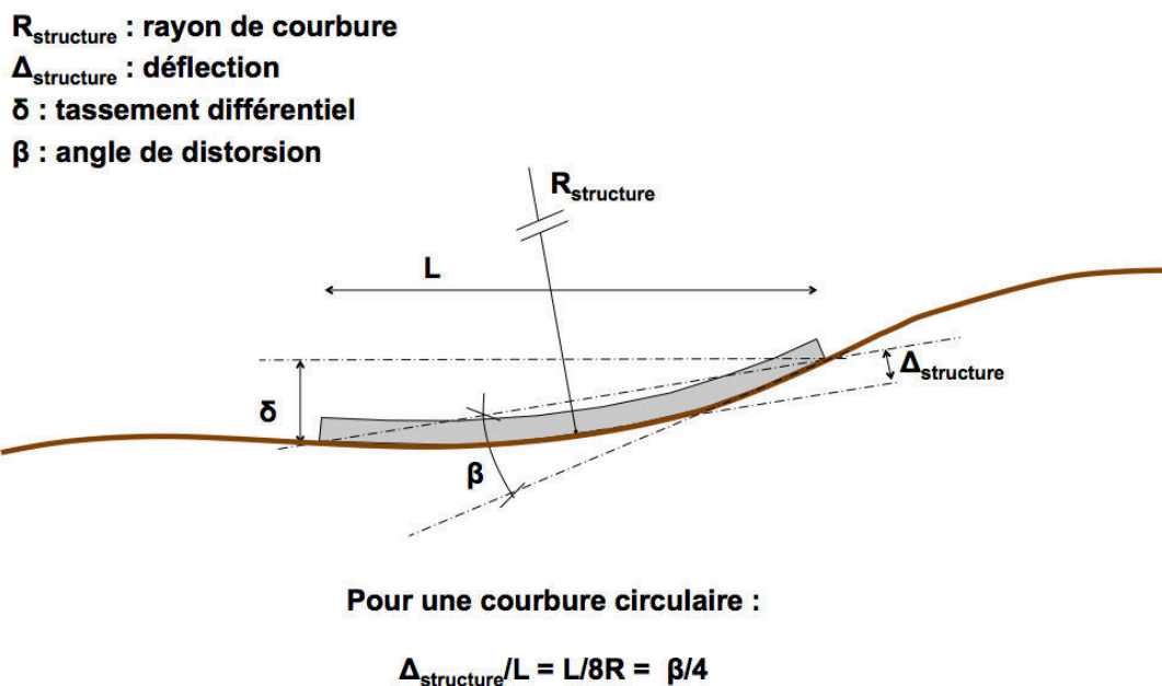
Figure 12 : Définition de quelques mouvements auxquels des seuils sont affectés
