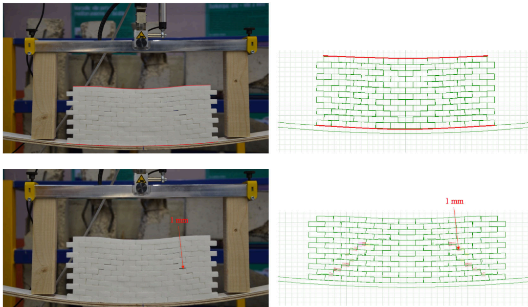
Figure 125 : Comparaison des modèles expérimental et numérique
