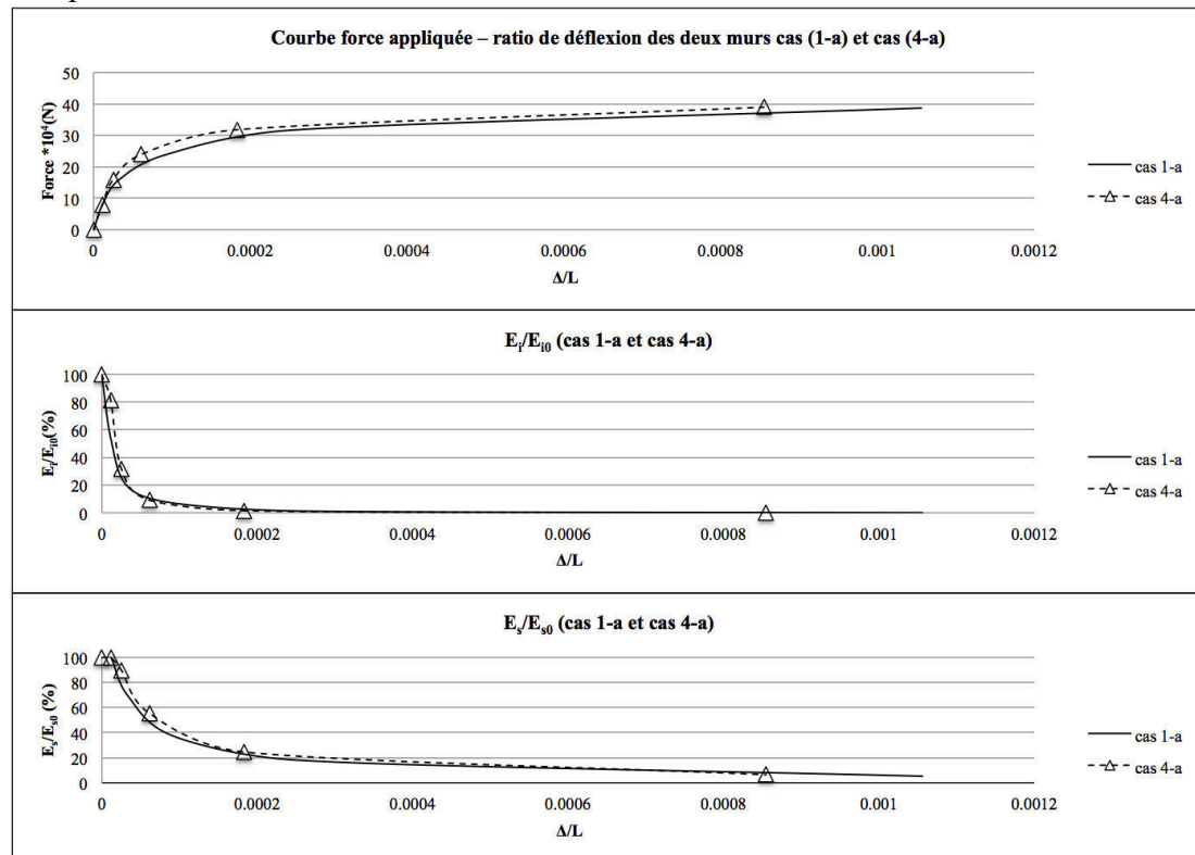
Figure 81 : Comparaison du comportement des deux murs (1-a) et (4-a)
