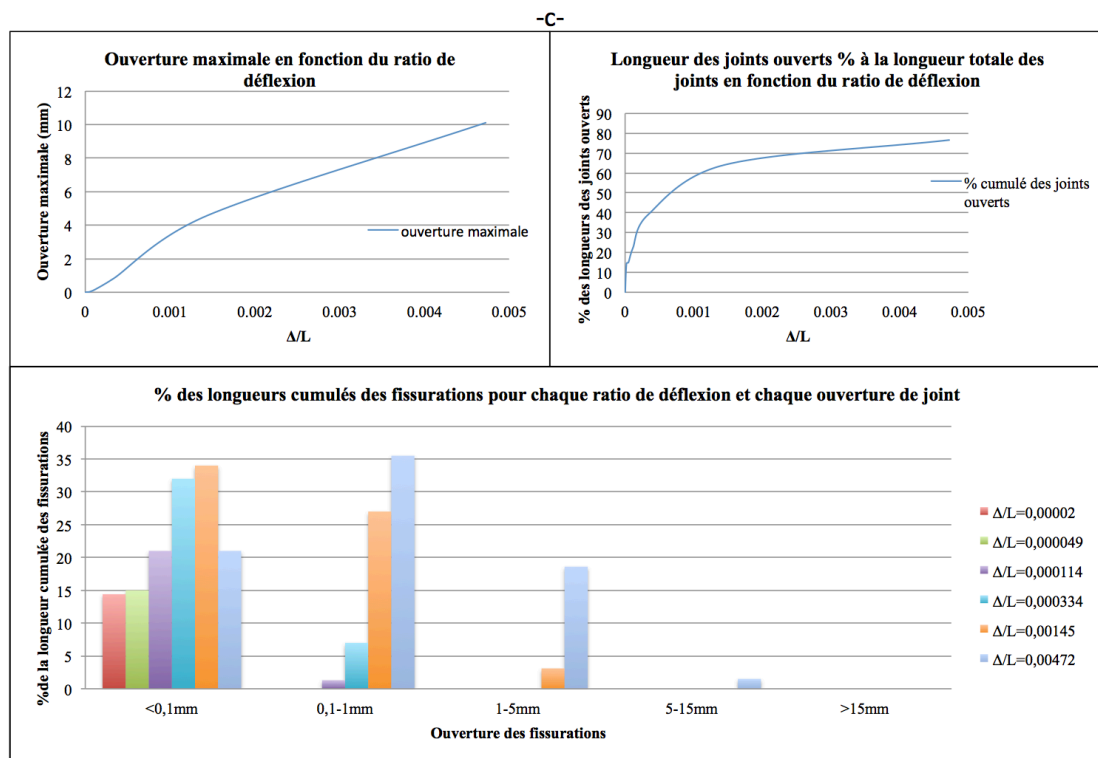
Figure 75 : Cas (2ii-a) – évolution de la rigidité et des ouvertures des joints en fonction de la déflexion subit.
