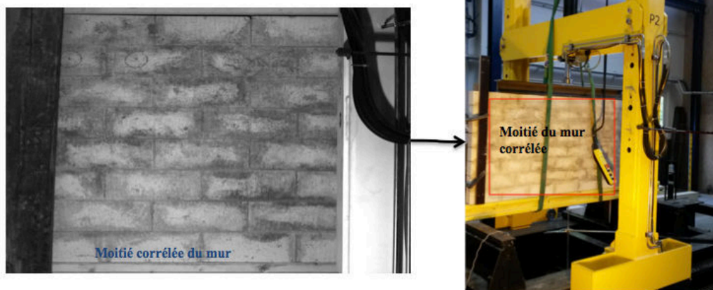
Figure 102 : Illustration de la zone photographiée pour la corrélation d'image.
