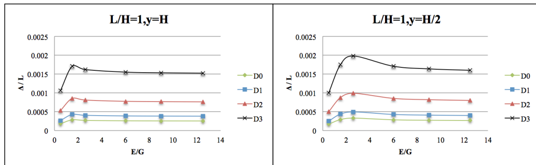
Figure 39 : Effet du ratio E/G sur les seuils du ratio de déflexion pour L/H=1 , effet de la position de l'axe neutre en fonction de E/G pour L/H=1
