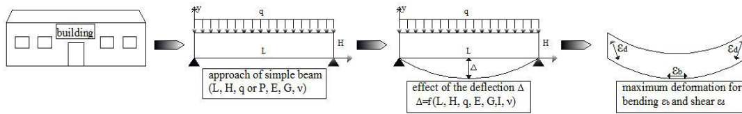
Figure 36 : Méthode analytique utilisée pour évaluer l'effet des propriétés des bâtiments sur les valeurs seuils du ratio de déflexion
