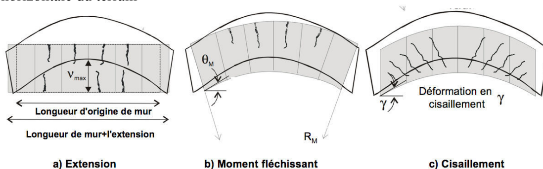
Figure 17 : Trois modes de déformation selon la méthode de superposition de Boone
