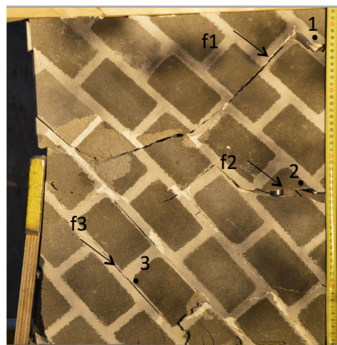
Figure 87 : Fissurations observées à la fin de l'essai (f1, f2 et f3)
