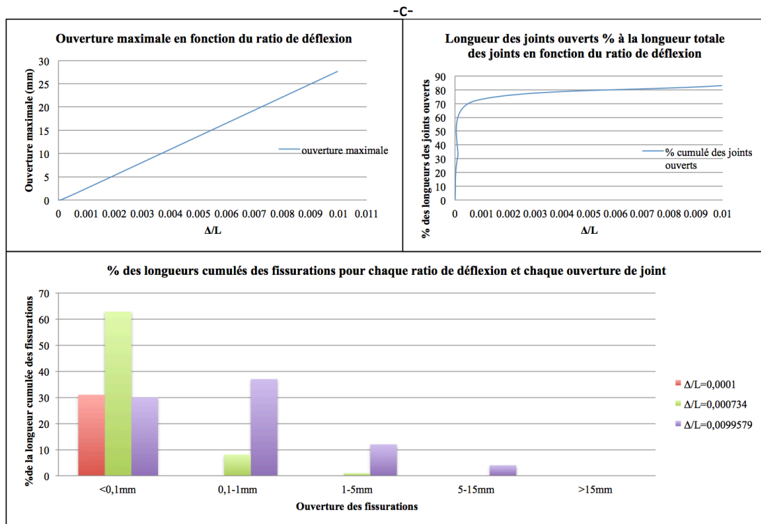
Figure 73 : Cas (1-b) – évolution de la rigidité et des ouvertures des joints en fonction de la déflexion subie.
