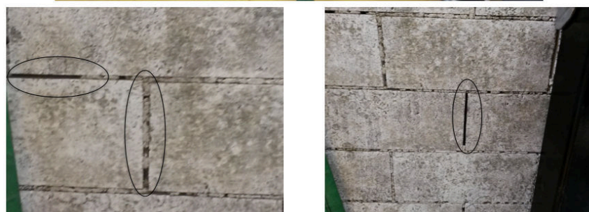
Figure 108 : Défaut de construction : quelques joints ne sont pas remplis complètement de mortier
