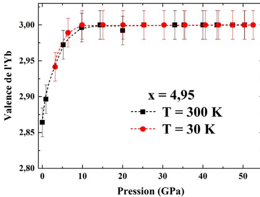
Figure IV.7 : Variation de la valence de l'ytterbium à 300 K et 30 K, sous l'effet de la pression externe, pour x = 4,95 .
