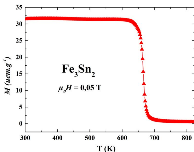
Figure VI.10 : Courbe thermomagnétique ( \mu_0 H = 0,05 \text{ T} ) de \text{Fe}_3\text{Sn}_2 .
