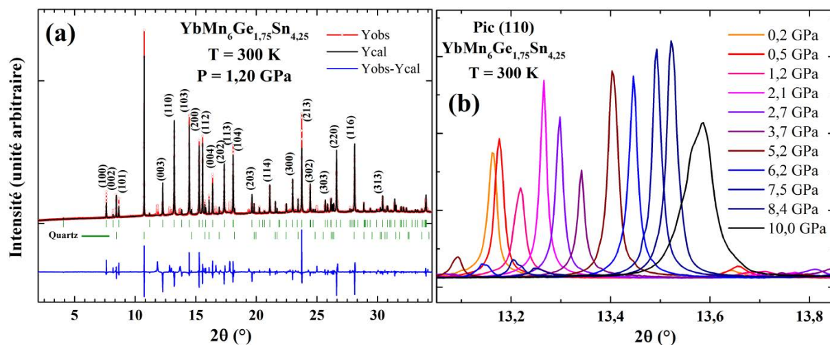
Figure IV.1 : Diffractogrammes de rayons X du composé x = 4,25 à 300 K. (a) Diffractogramme complet pour P \sim 1,20 GPa. (b) Région angulaire restreinte proche du pic (110) pour différentes pressions.
