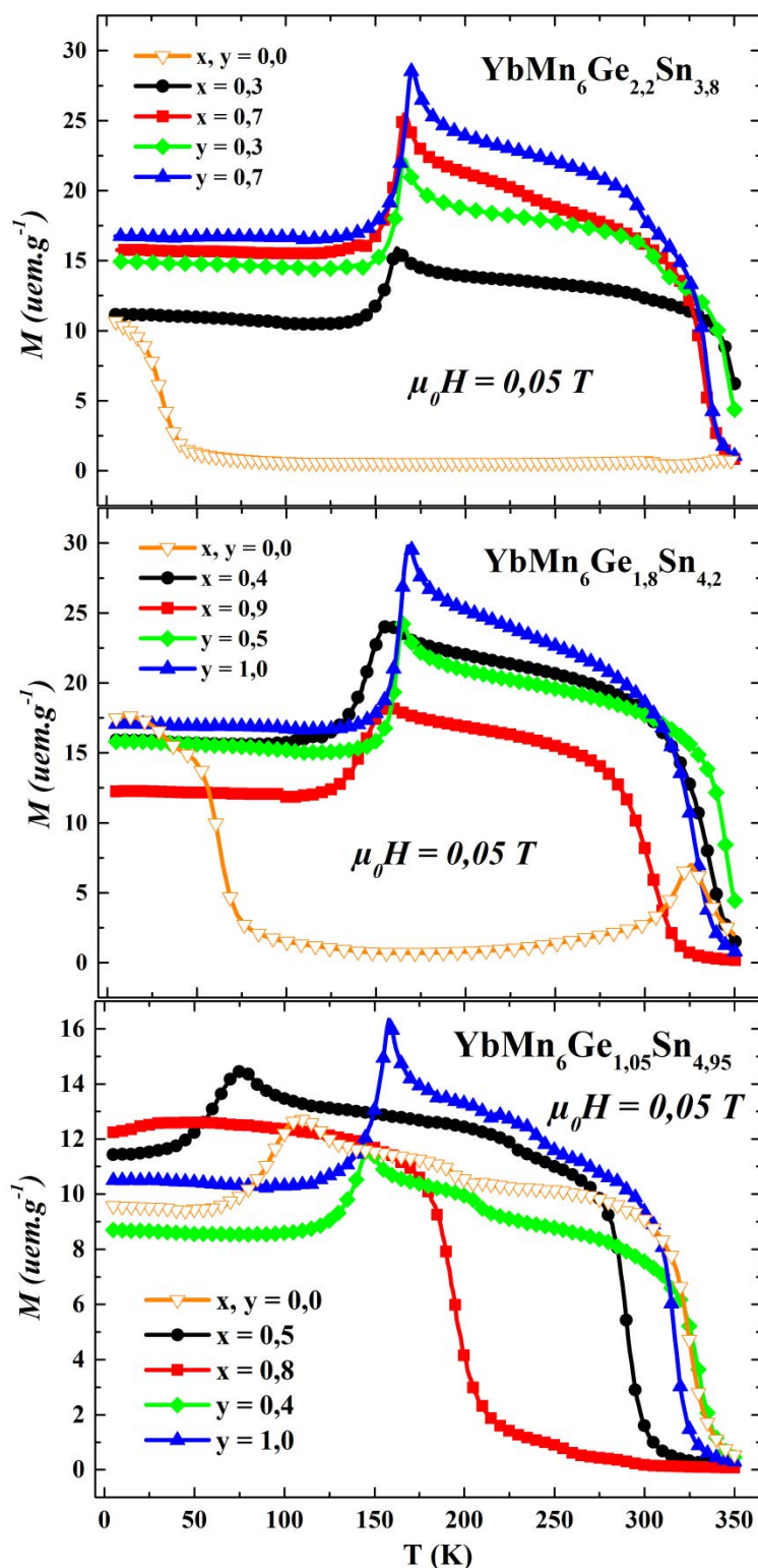
Figure V.4 : Courbes thermomagnétiques ( \mu_0 H = 0,05 T) des composés \text{YbMn}_6\text{Ge}_{2,2-x}\text{Sn}_{3,8}\text{Ga}_x et \text{YbMn}_6\text{Ge}_{2,2}\text{Sn}_{3,8-y}\text{Ga}_y ; \text{YbMn}_6\text{Ge}_{1,8-x}\text{Sn}_{4,2}\text{Ga}_x et \text{YbMn}_6\text{Ge}_{1,8}\text{Sn}_{4,2-y}\text{Ga}_y ; \text{YbMn}_6\text{Ge}_{1,05-x}\text{Sn}_{4,95}\text{Ga}_x et \text{YbMn}_6\text{Ge}_{1,05}\text{Sn}_{4,95-y}\text{Ga}_y . Les données concernant les composés non substitués \text{YbMn}_6\text{Ge}_{2,2}\text{Sn}_{3,8} et \text{YbMn}_6\text{Ge}_{1,8}\text{Sn}_{4,2} sont issues de [9].
