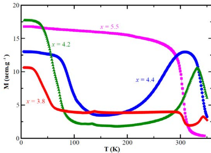
Figure II.10 : Courbes thermomagnétiques pour différents comportements de la série \text{YbMn}_6\text{Ge}_{6-x}\text{Sn}_x ( x = 3,8 ; 4,2 ; 4,4 et 5,5 ) [34].
