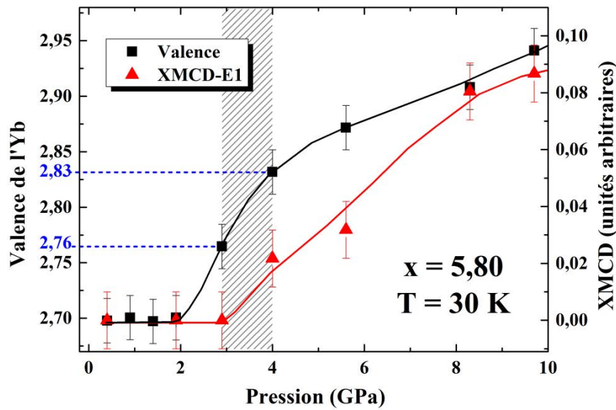
Figure IV.13 : Valence de l'ytterbium (symboles noirs, échelle de gauche) et intensité de la contribution E1 du signal XMCD (symboles rouges, échelle de droite) en fonction de la pression pour x = 5,80 ( T = 30 K).
