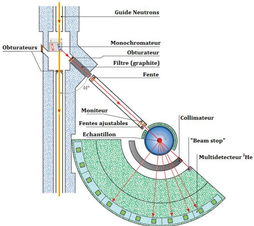
Figure I.5 : Schéma descriptif du diffractomètre D1b à l'ILL [13].
