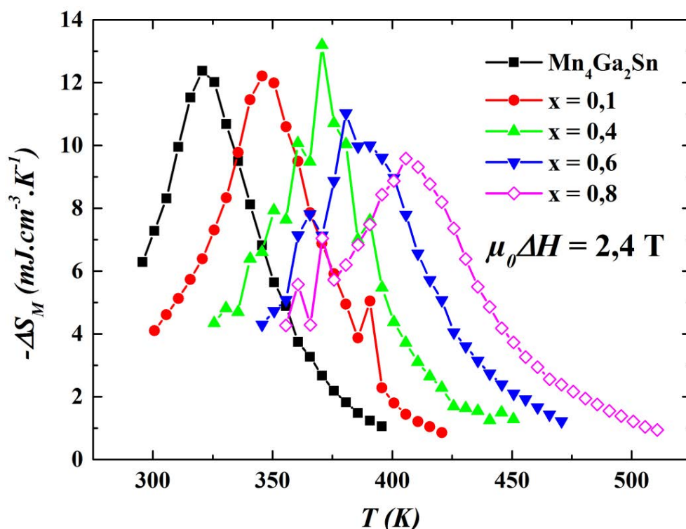
Figure VI.9 : Evolution thermique de la variation d'entropie magnétique des composés \text{Mn}_{4-x}\text{Fe}_x\text{Ga}_2\text{Sn} .
