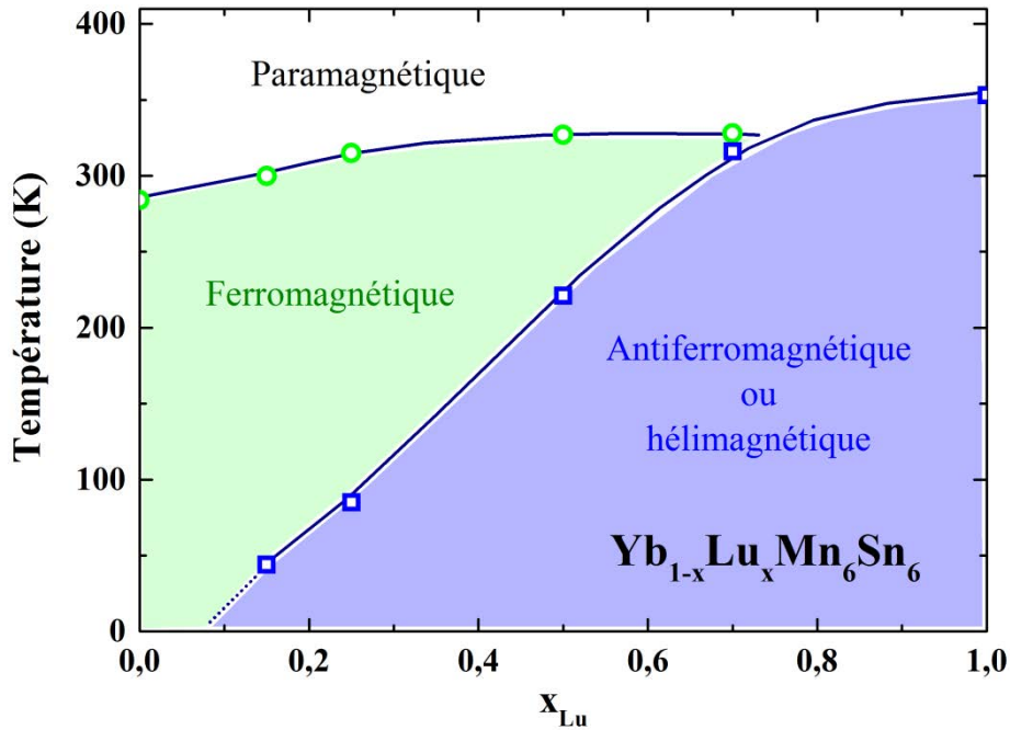
Figure V.16 : Diagramme de phase magnétique ( x, T ) de la série \text{Yb}_{1-x}\text{Lu}_x\text{Mn}_6\text{Sn}_6 . Les carrés bleus repèrent les températures de transition antiferromagnétique ou hélimagnétique ( T_{AF} ou T_N ) alors que les cercles verts repèrent les températures de mise en ordre ferromagnétique ( T_C ) du sous-réseau de Mn.
