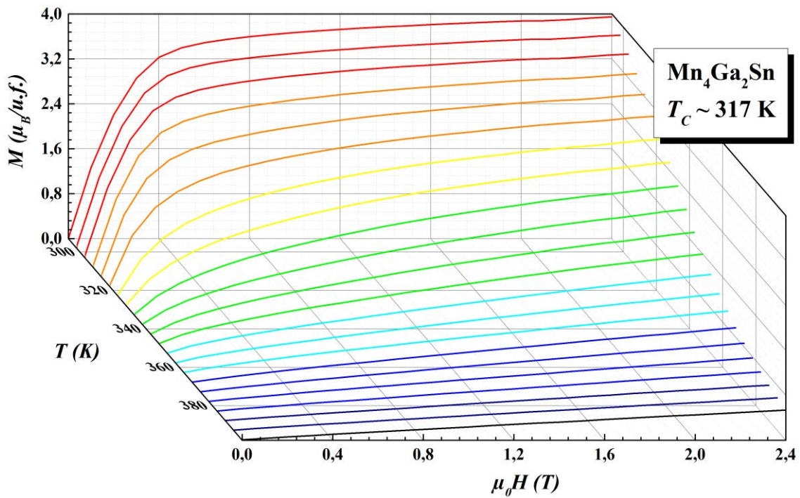
Figure VI.8 : Courbes d'aimantation isotherme de Mn_4Ga_2Sn entre 290 et 400 K.
