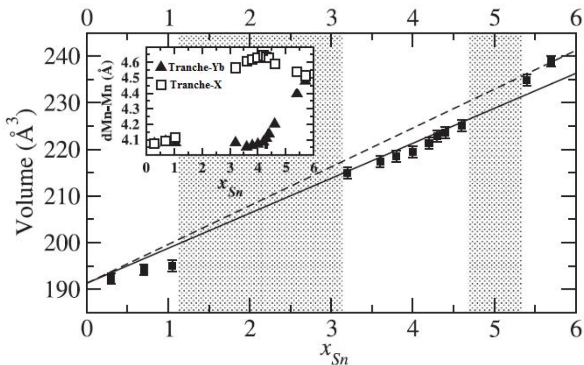
Figure II.5 : Evolution du volume de la maille des composés \text{YbMn}_6\text{Ge}_{6-x}\text{Sn}_x en fonction de la teneur en étain. Les zones grisées repèrent les lacunes de miscibilité. L'insert montre l'évolution de la distance Mn-Mn interplanaire au travers des tranches Yb et X [34].
