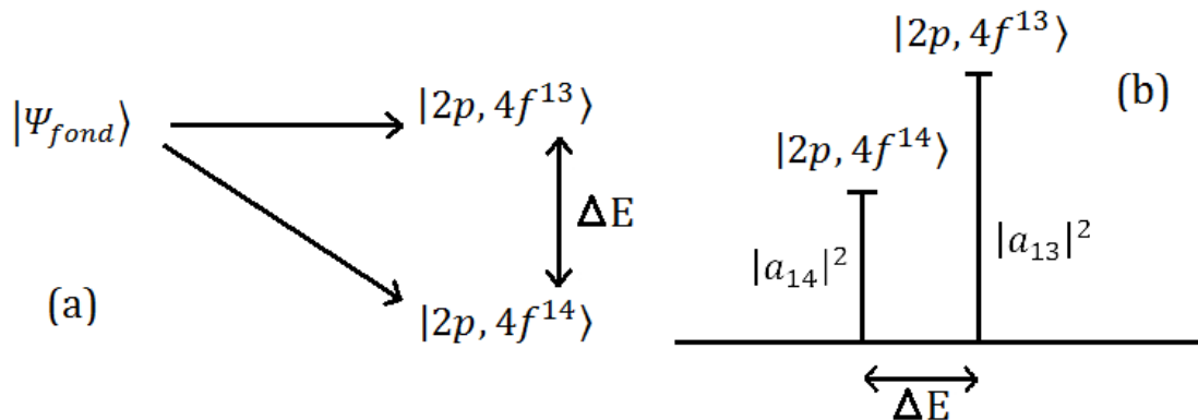
Figure I.10 : Représentation schématisée de l'état fondamental et des états finaux du seuil L_3 de l'ytterbium (a) ainsi que du spectre d'absorption X (b).
