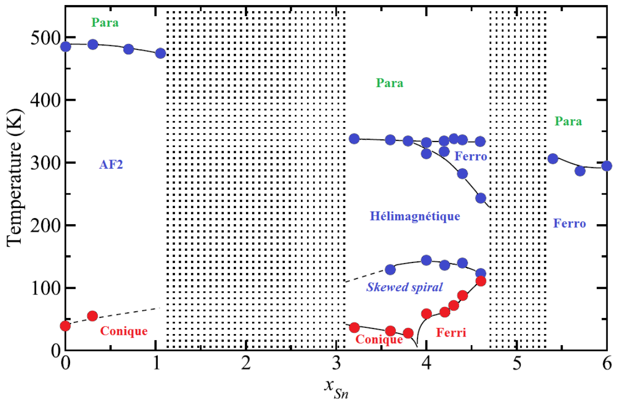
Figure II.9 : Diagramme de phase magnétique ( x , T ) de la série \text{YbMn}_6\text{Ge}_{6-x}\text{Sn}_x , en bleu les températures des transitions magnétiques du sous-réseau de Mn, en rouge celles du sous-réseau d'Yb [34].
