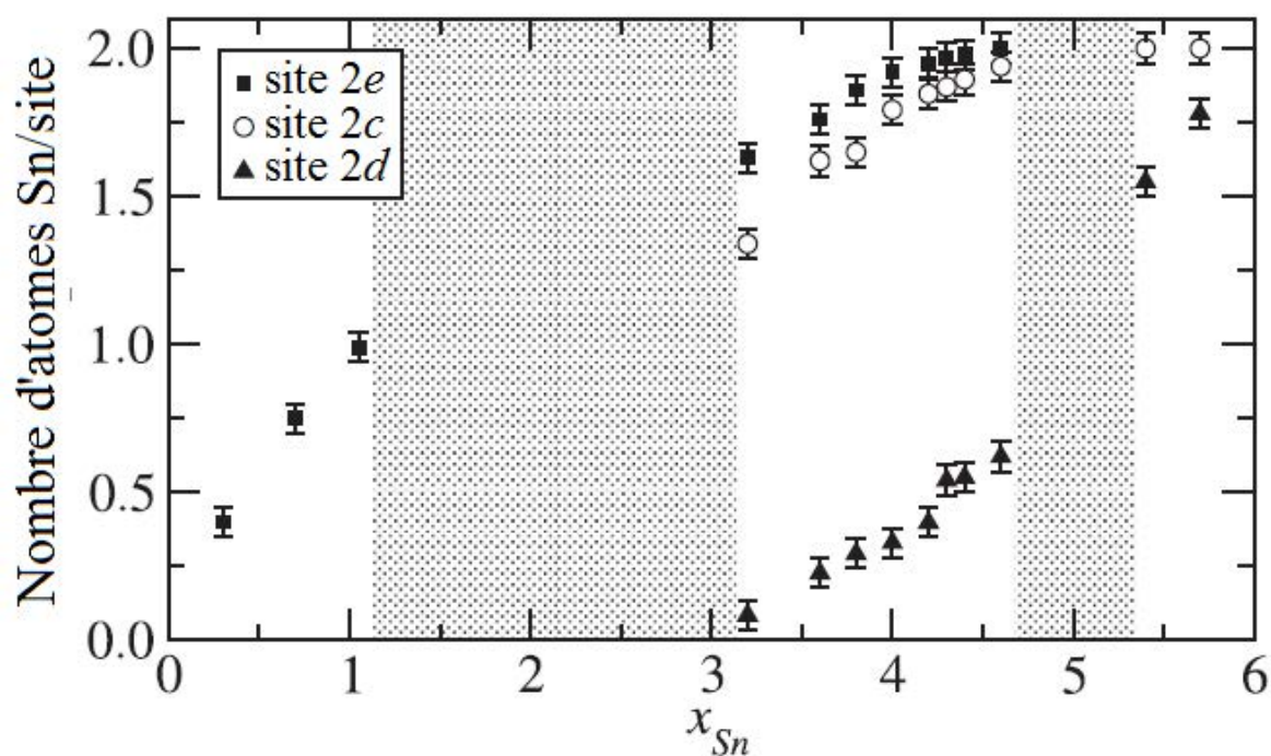
Figure II.6 : Evolution de l'occupation des trois sites de métalloïde par les atomes d'étain, dans composés \text{YbMn}_6\text{Ge}_{6-x}\text{Sn}_x , en fonction de la teneur en étain [34].
