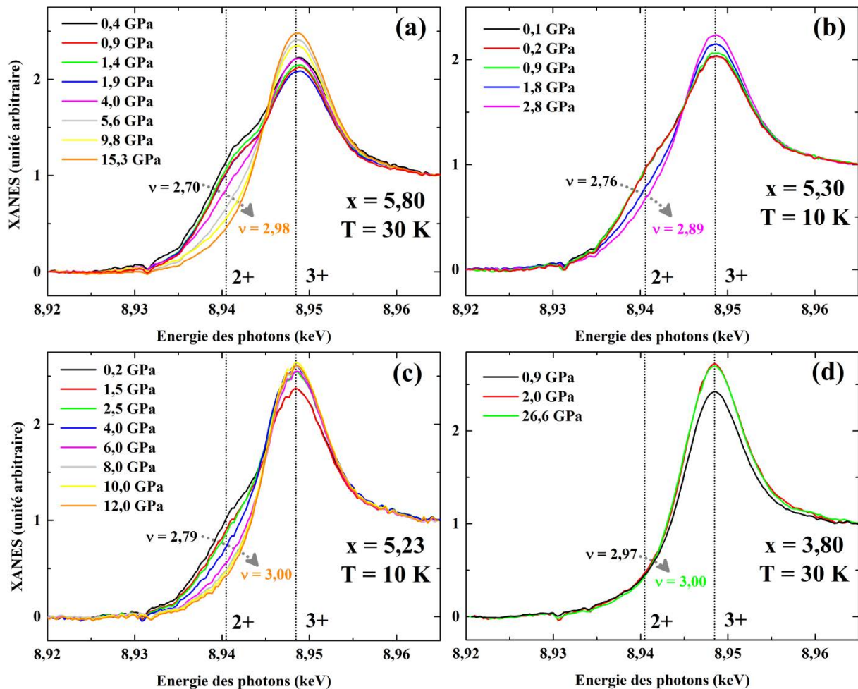
Figure IV.5 : Spectres XANES enregistés au seuil L_3 de l'ytterbium, à basse température (10 K ou 30 K) et sous pression, pour les composés riches en Sn dans la série \text{YbMn}_6\text{Ge}_{6-x}\text{Sn}_x . (a) x = 5,80 ; (b) x = 5,30 ; (c) x = 5,23 ; (d) x = 3,80 .
