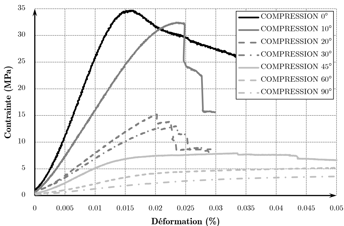
Figure II-45 : Courbes des essais en compression uniforme selon un angle
