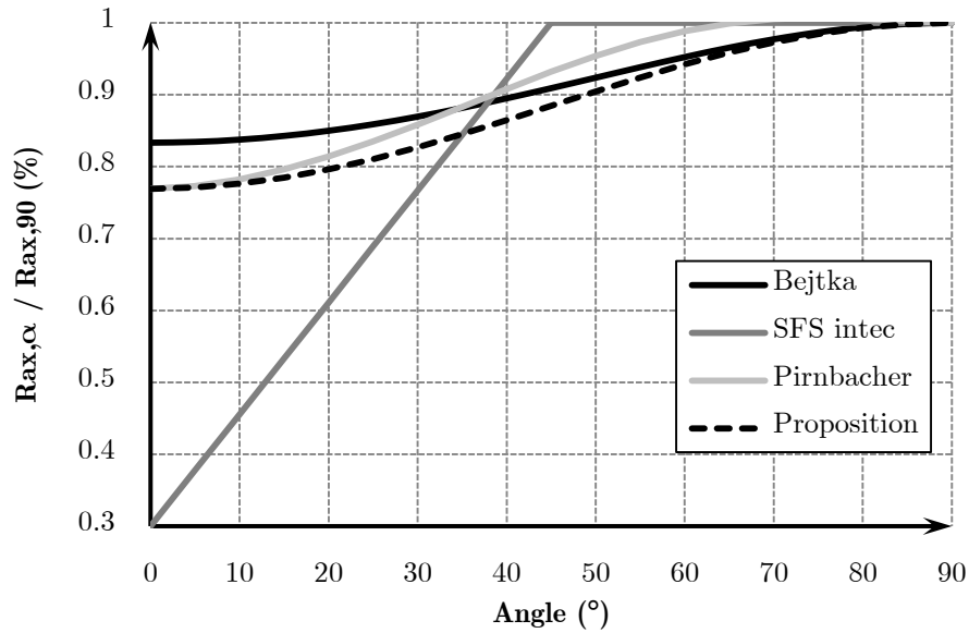
Figure III-89 : Capacité résistance à l'arrachement en fonction de l'angle
