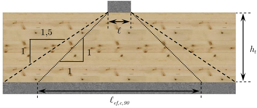
Figure I-22 : Distribution des contraintes selon Van Der Put [63]
