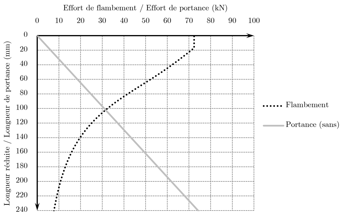
Figure III-95 : Détermination de la longueur réduite maximale des vis WB-16
