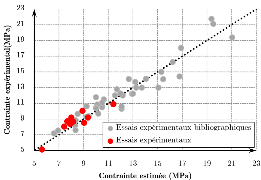
Figure III-129 : Prédiction du modèle en contrainte vs Essais expérimentaux renforcés
