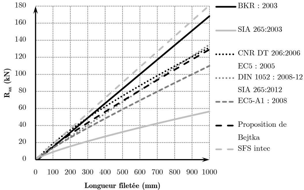
Figure I-37 : Capacité résistance à l'arrachement en fonction de la longueur avec un diamètre de vis de 13mm et une masse volumique de 385 kg/m³.
