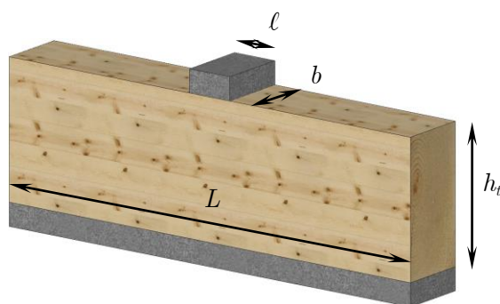
Figure III-97 : Echantillon expérimenté
