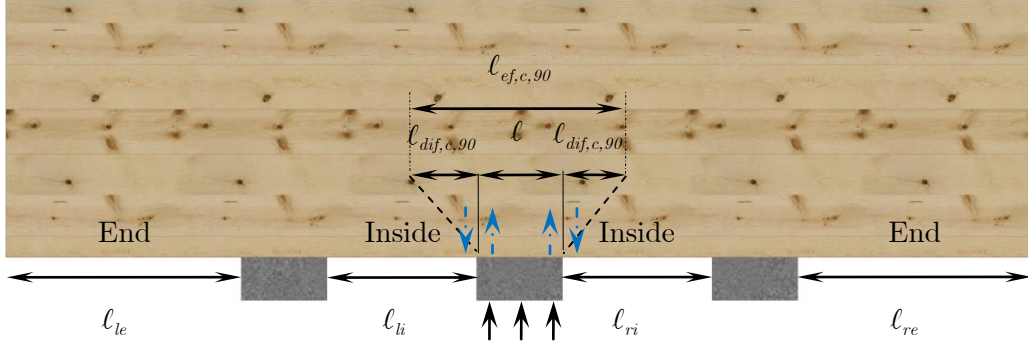
Figure II-68: Détermination de la longueur efficace en compression perpendiculaire au fil
