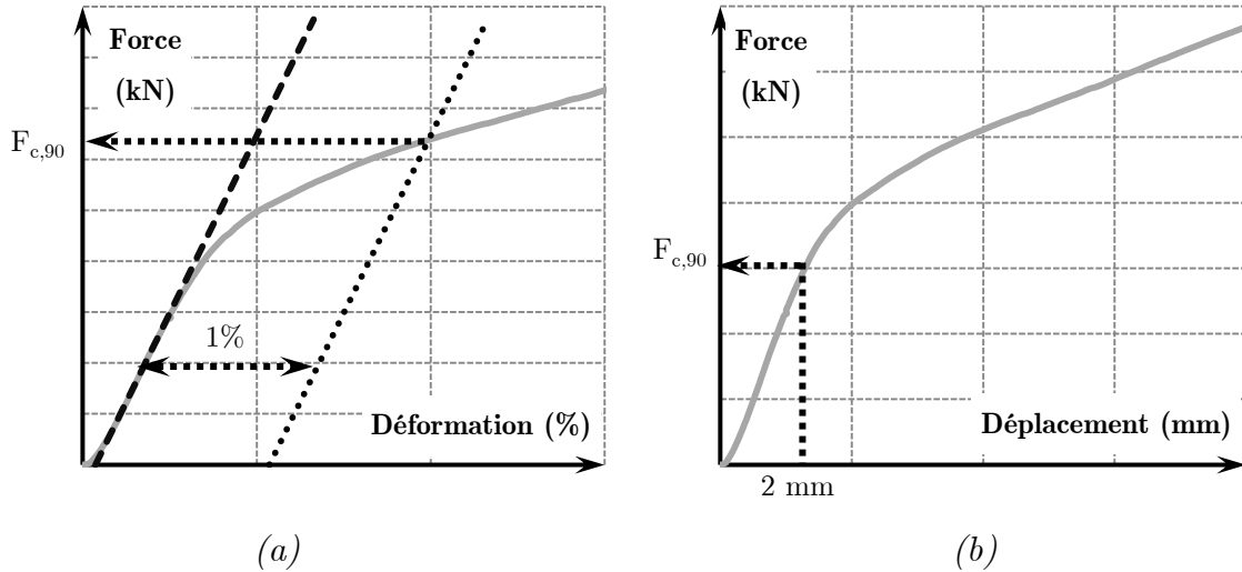
Figure I-18 : Détermination de la résistance en compression selon la norme EN 408 [10] (a) et la norme ASTM D3737-12 [28] (b)
