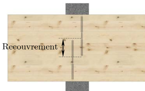
Figure III-127 : Recouvrement des vis
