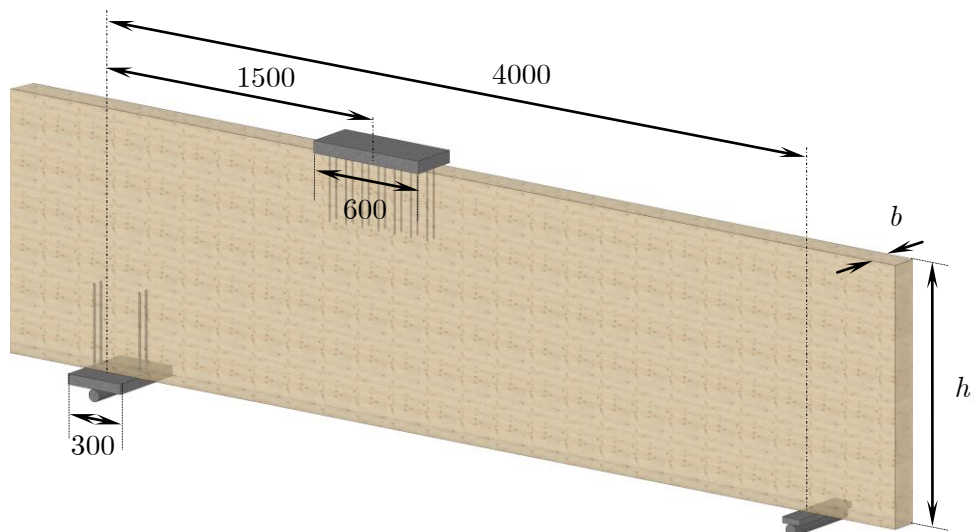
Figure III-119: Renforcement en compression perpendiculaire au fil sur des essais de flexion à l'échelle structurale
