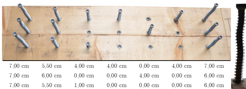
Figure III-124: Longueurs de flambement des essais à 21 vis
