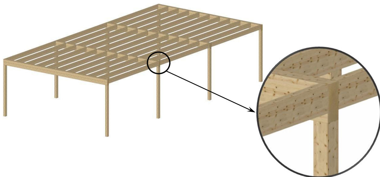
Figure I-5 : Système poteau/poutre
