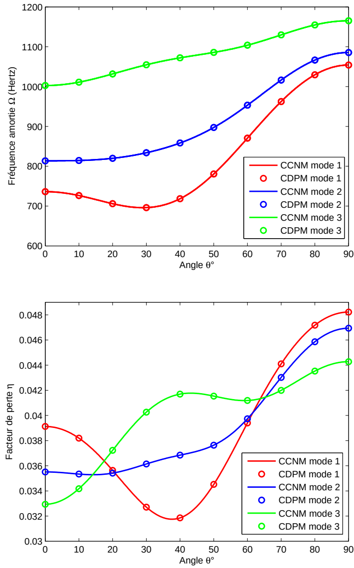
Figure 4.9 – Etude continue des propriétés modales de la plaque 7, CL : CCCC
