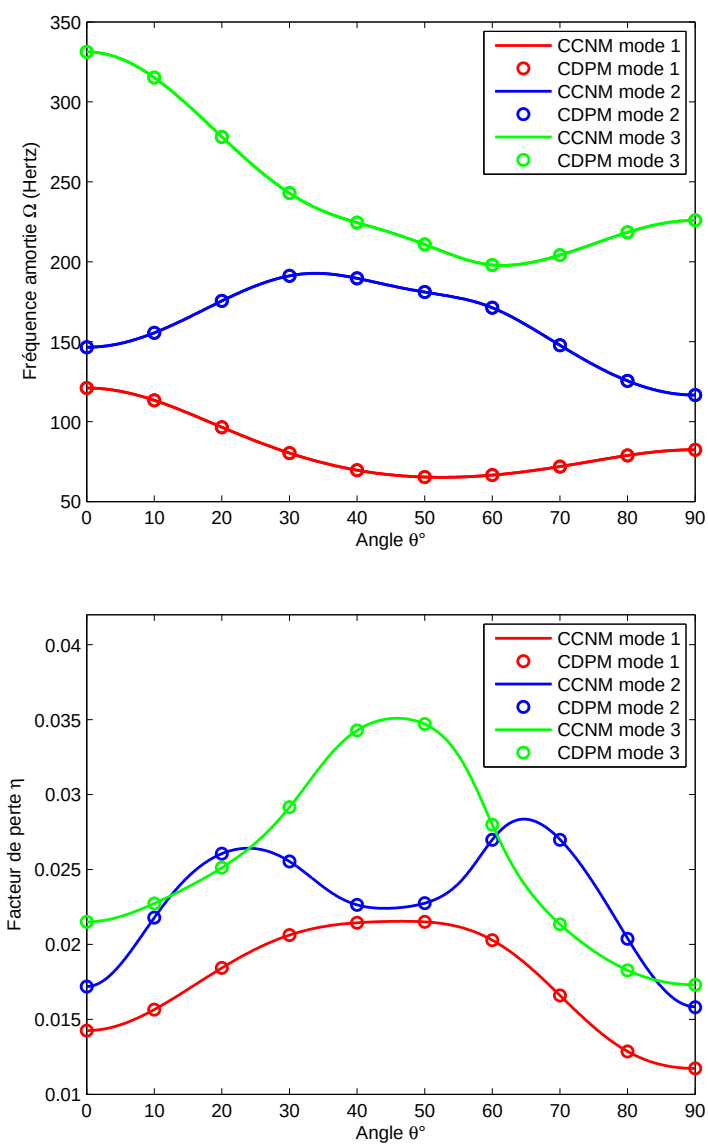
Figure 4.11 – Etude continue des propriétés modales de la plaque 7, CL : CFCF
