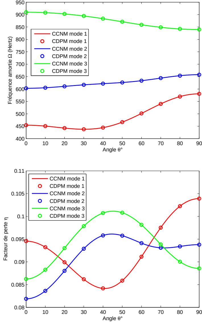
Figure 4.13 – Etude continue des propriétés modales de la plaque 8, CL : CCCC
