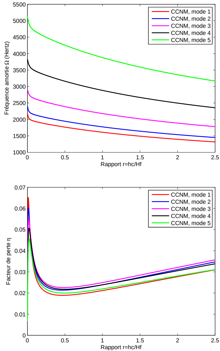
Figure 5.18 – Etude continue des propriétés modales de la plaque 9 en fonction de l'épaisseur du cœur en ISD112 à 27°C (cinq premiers modes pour la séquence [0^\circ/90^\circ/0^\circ/90^\circ/c]_s ), CL : CCCC
