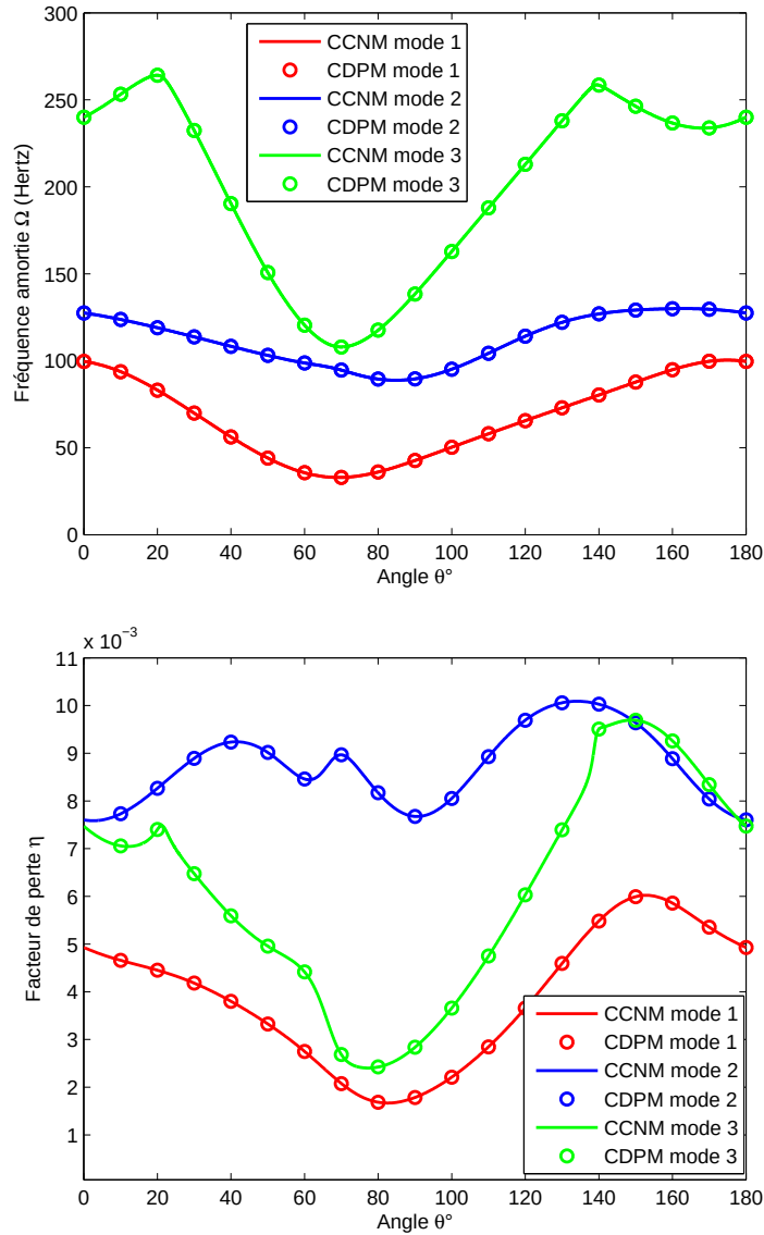
Figure 4.15 – Étude continue des propriétés modales de la plaque 9, CL : CFSF
