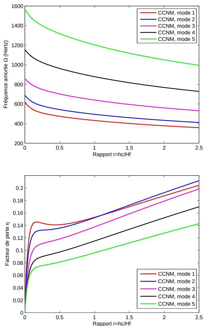
Figure 5.16 – Etude continue des propriétés modales de la plaque 7 en fonction de l'épaisseur du cœur en ISD112 à 27°C (cinq premiers modes pour la séquence [0^\circ/90^\circ/0^\circ/c]_s ), CL : CCCC
