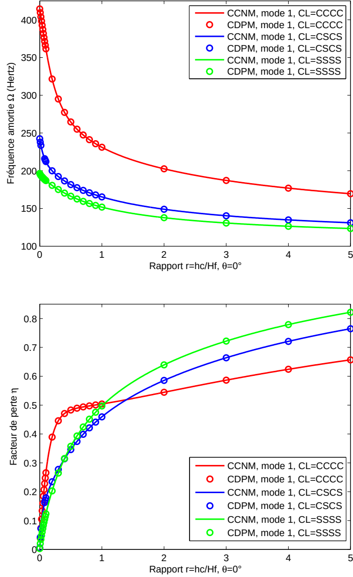
Figure 5.4 – Etude continue des propriétés modales de la plaque 6 en fonction de l'épaisseur du cœur ( \theta = 0^\circ mode 1)
