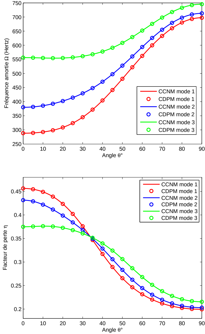
Figure 4.6 – Etude continue des propriétés modales de la plaque 6, CL : CCCC
