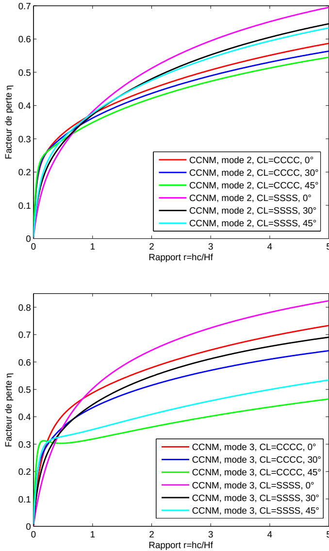
Figure 5.15 – Etude continue des propriétés modales de la plaque carrée en fonction de l'épaisseur du cœur (amortissement des modes 2 et 3), CL : CCCC et SSSS
