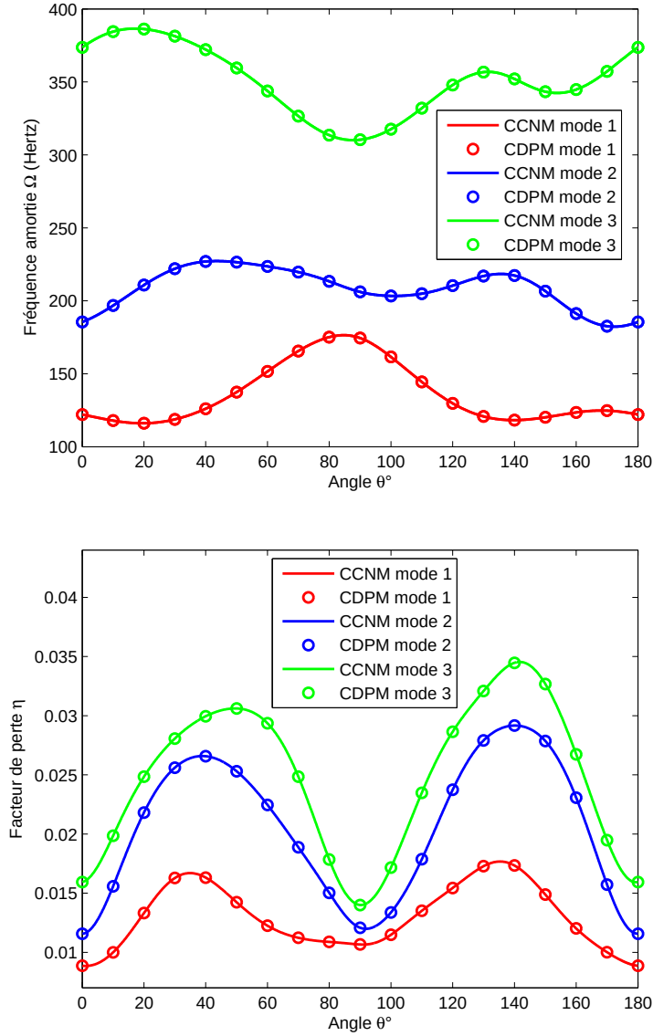
Figure 4.12 – Etude continue des propriétés modales de la plaque 7, CL : CCFF
