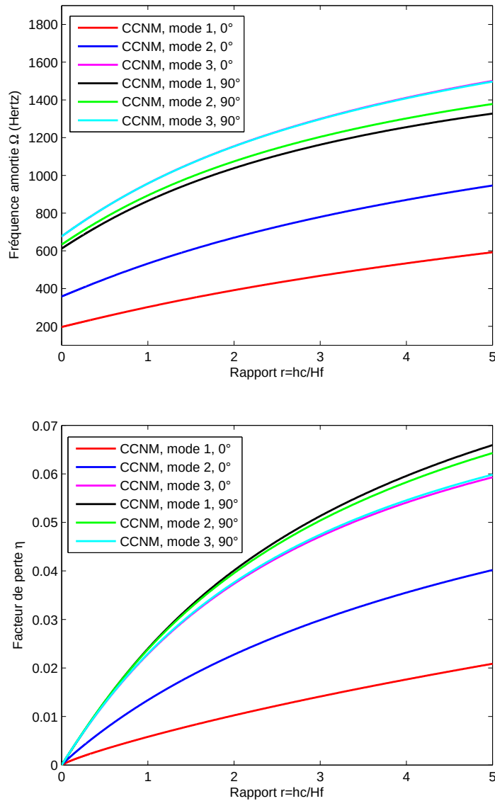
Figure 5.13 – Etude continue des propriétés modales de la plaque 6 en fonction de l'épaisseur du cœur en PVB à 20^\circ\text{C} (trois premiers modes pour \theta = 0^\circ et \theta = 90^\circ ), CL : SSSS
