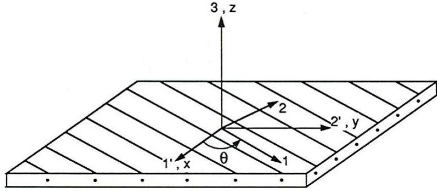
Figure 1.7 – Matériau : repère matériau et de référence de la structure
