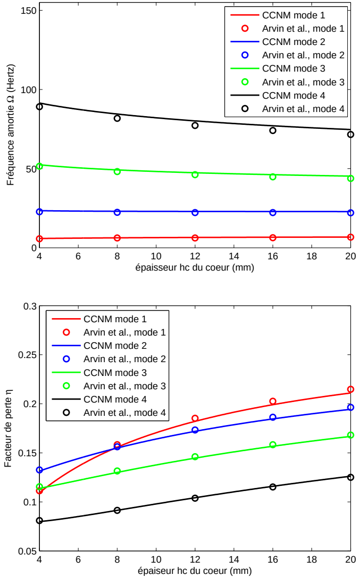
Figure 5.3 – Étude continue des propriétés modales de la poutre en fonction de l'épaisseur du cœur ( \theta = 30^\circ )
