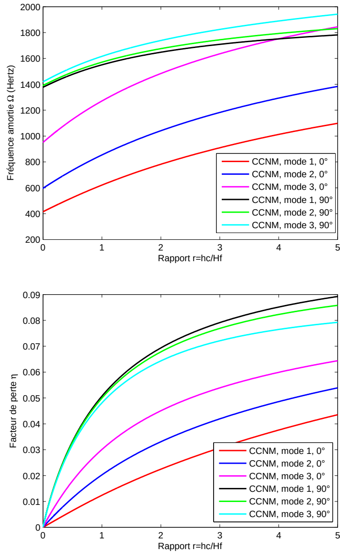
Figure 5.12 – Etude continue des propriétés modales de la plaque 6 en fonction de l'épaisseur du cœur en PVB à 20°C (trois premiers modes pour \theta = 0^\circ et \theta = 90^\circ ), CL : CCCC
