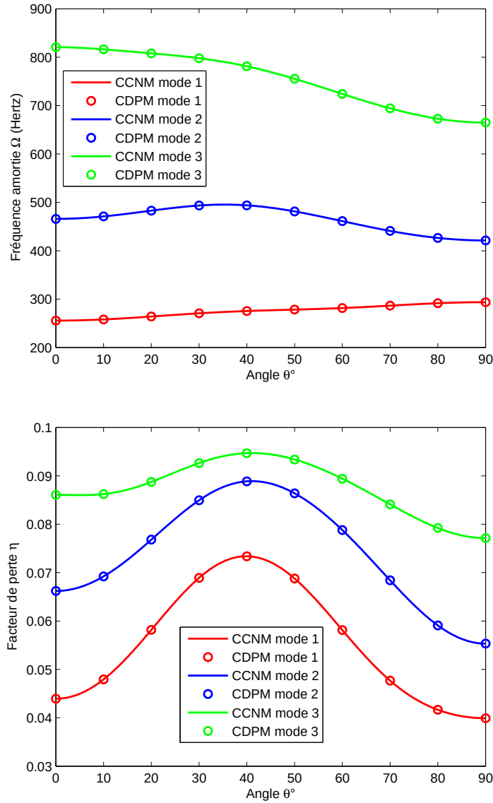
Figure 4.14 – Etude continue des propriétés modales de la plaque 8, CL : CSCS
