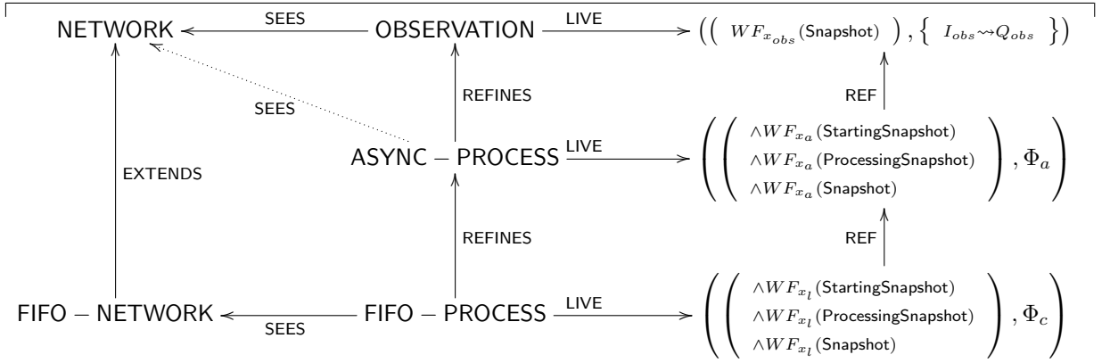
FIGURE 7.9 – Algorithme de Chandy et Lamport
