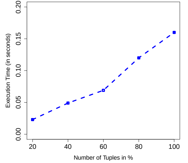
(d) Runtime for Building \mathcal{L}_{DBpedia}
