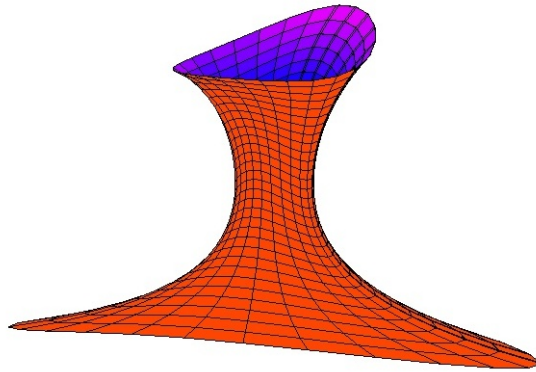
FIGURE 1.5 – Caténoïde pour \alpha = -0.6 avec Scilab®.
