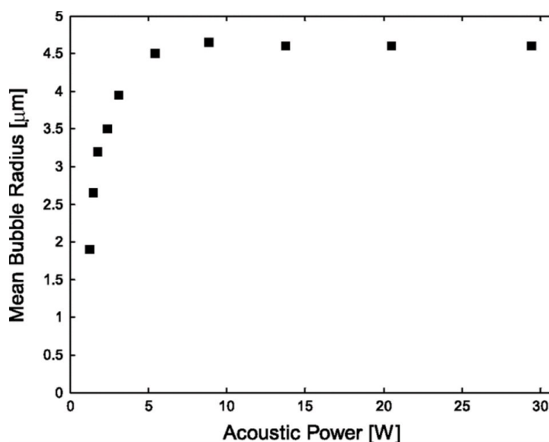
Figure 15 : Variation des rayons des bulles de cavitation (moyenne de la distribution de taille) sous sonication par ultrasons 1056 kHz de fréquence en fonction de la puissance acoustique. (Brotchie, Grieser et al. 2009).
