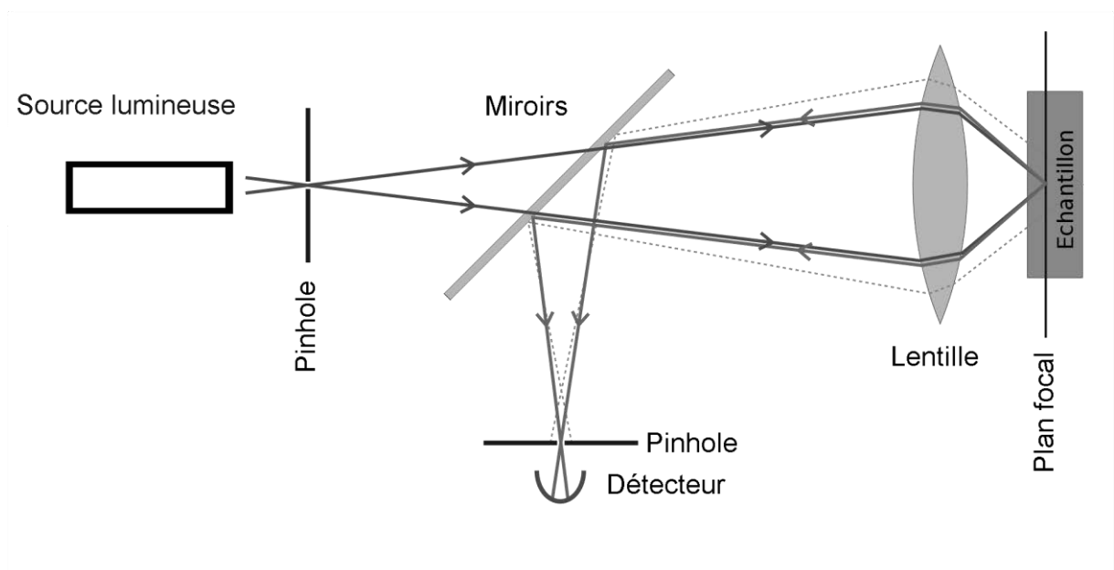
Fig. 169 : Schéma de fonctionnement d'un microscope confocal.
