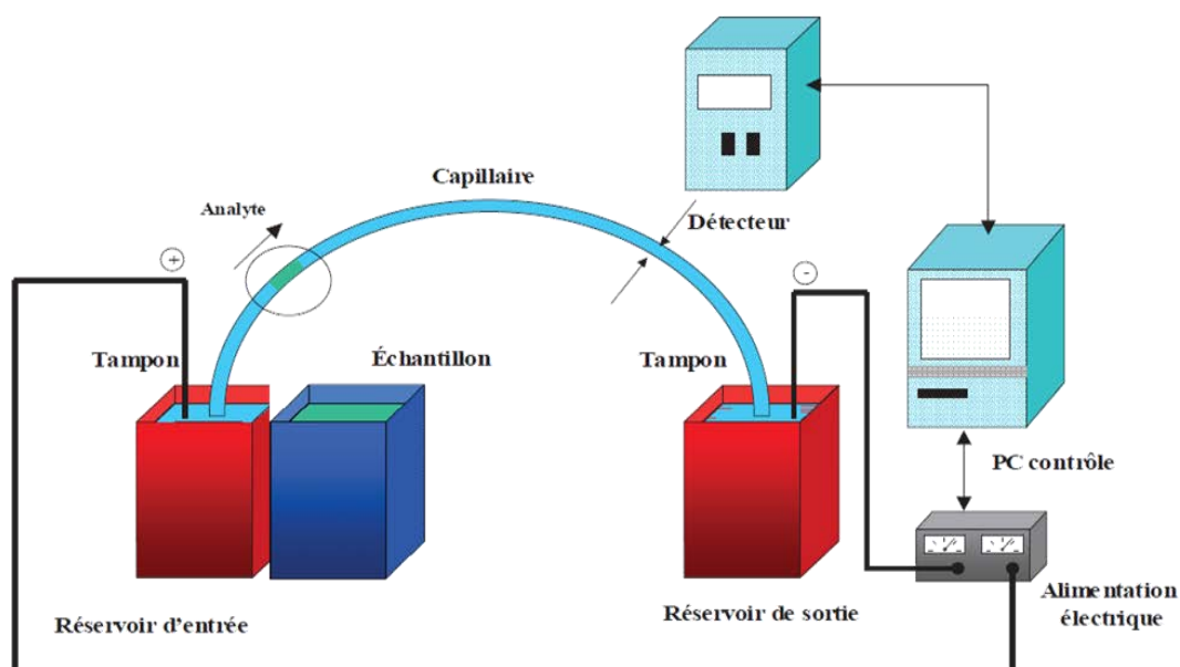
Fig. 147 : Schéma des composants principaux d'une électrophorèse capillaire.
