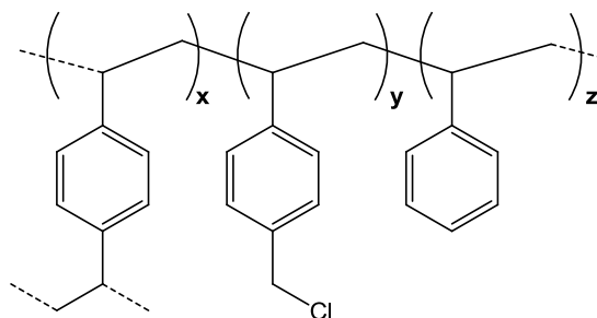
Fig. 69 : Schéma d'une résine de Merrifield polymérisée vierge
