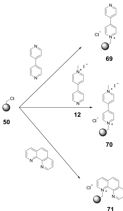
Fig. 159 : Greffages de motifs 4,4'-bipyridinium et phénantroline sur la résine de Merrifield vierge 50 .
