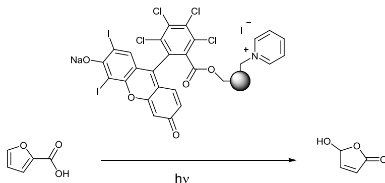
Fig. 34 : Photooxydation de l'acide 2-furoïque en 5-hydroxy-5H-furan-2-one par l'utilisation d'un catalyseur supporté par Burguete et al. 60
