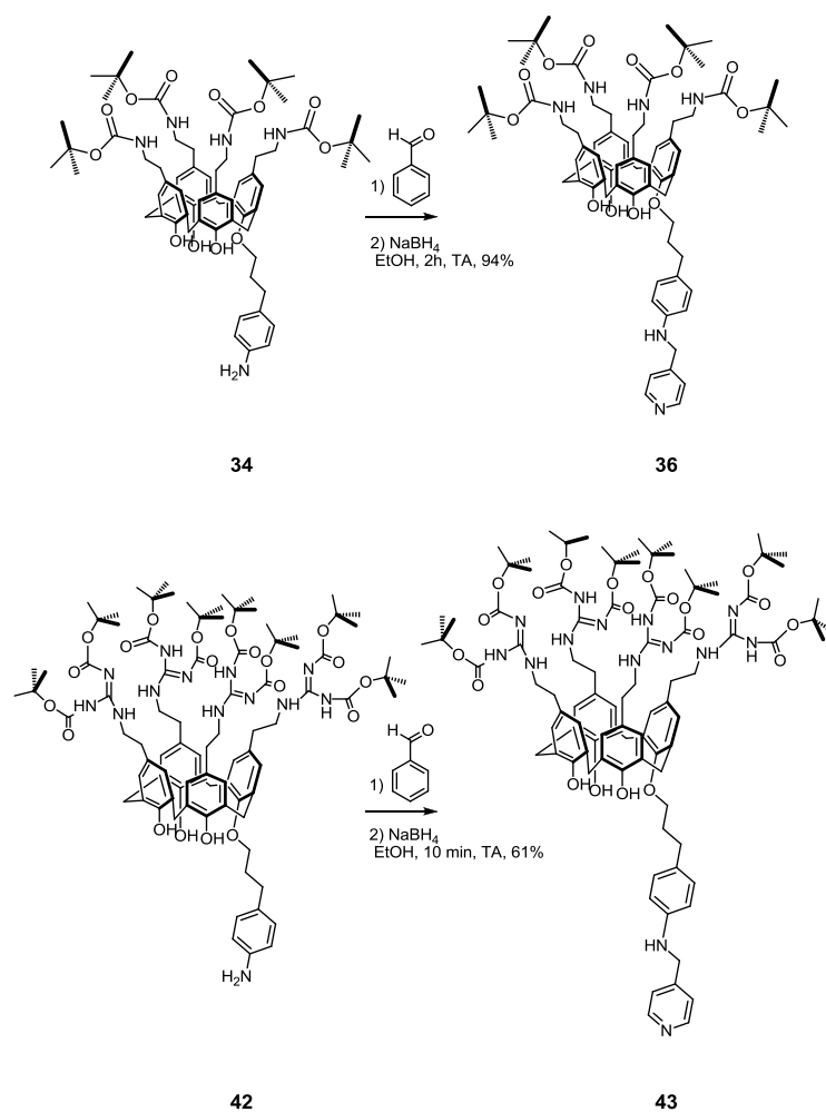
Fig. 65 : Synthèse des dérivés calixaréniques pyridinés par amination réductrice de la 4-pyridinecarboxaldéhyde.
