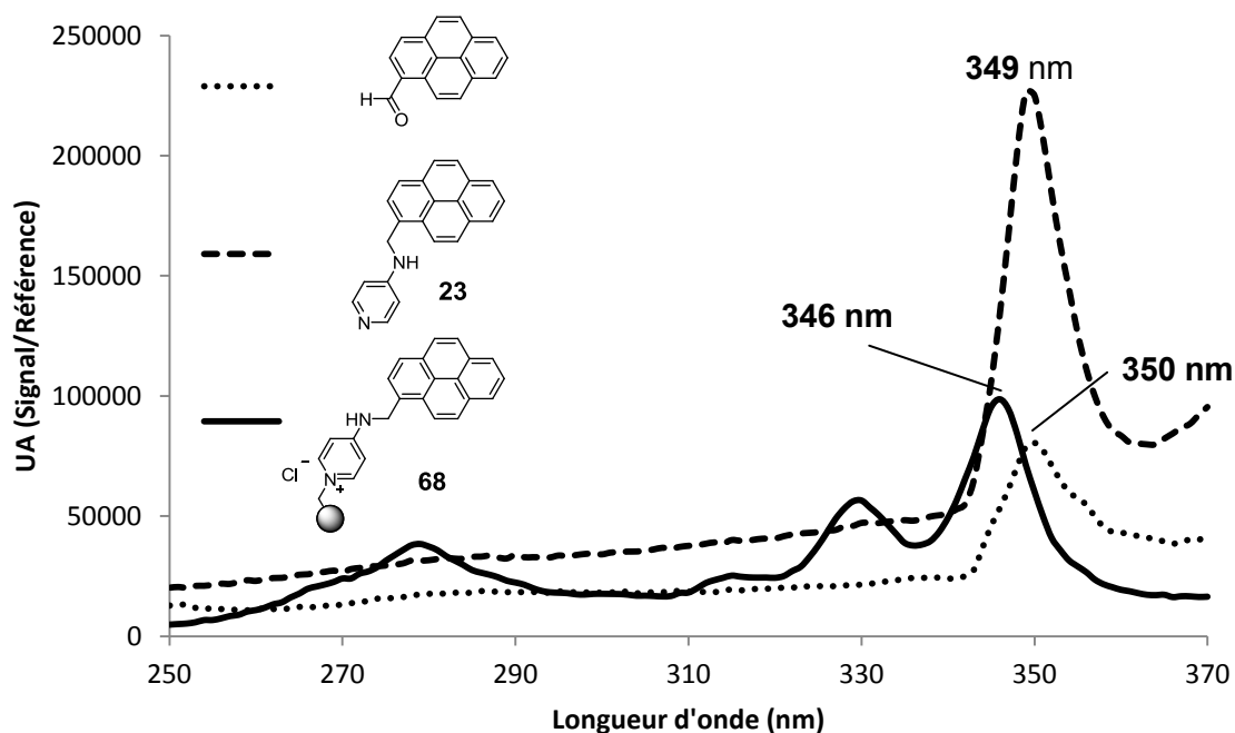
Fig. 88 : Spectres d'excitation du 1-pyrèncarboxaldéhyde, de la 4-[(pyrène-1-yl)-méthylamino]-pyridine 23 et de la résine pyrène-pyridinium 68
