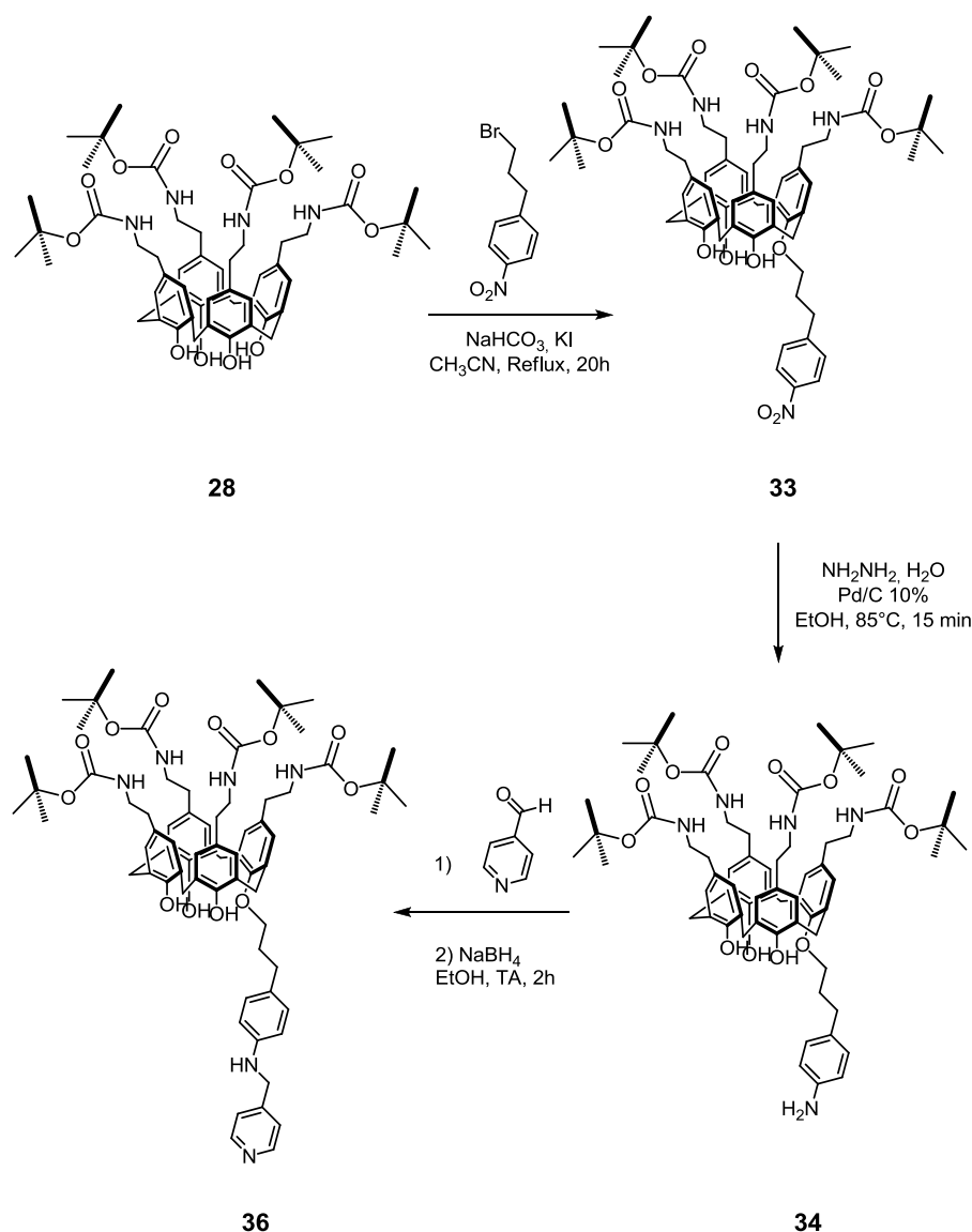
Fig. 92 : Voie de synthèse du dérivé pyridiné 36.
