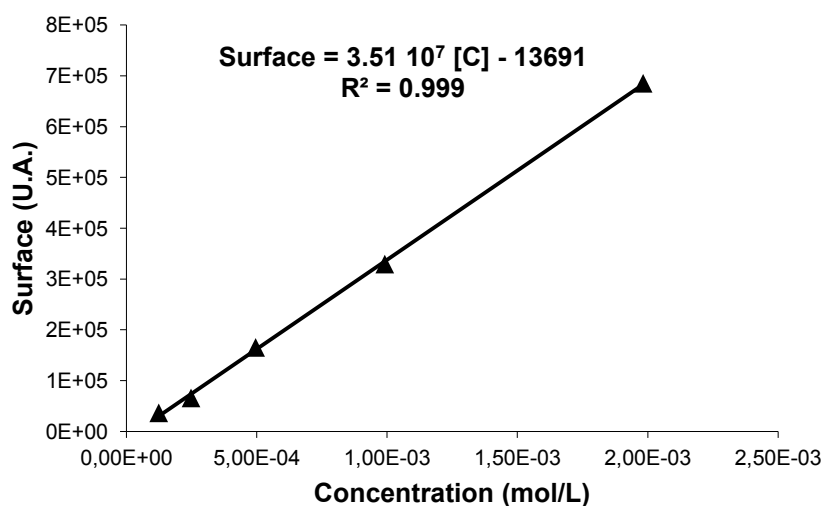
Fig. 136 : Etude de linéarité du pénicillinate de potassium en CLHP.
