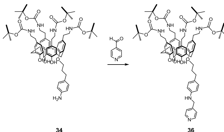
Fig. 97 : Amination réductrice du dérivé anilino 34 sur la 4-pyridinecarboxaldéhyde.
