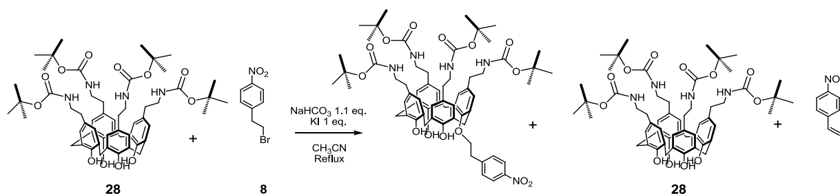
Fig. 62 : Tentatives de formation du dérivé calixarène mono-O-éthyl-( para -nitrobenzyle).
