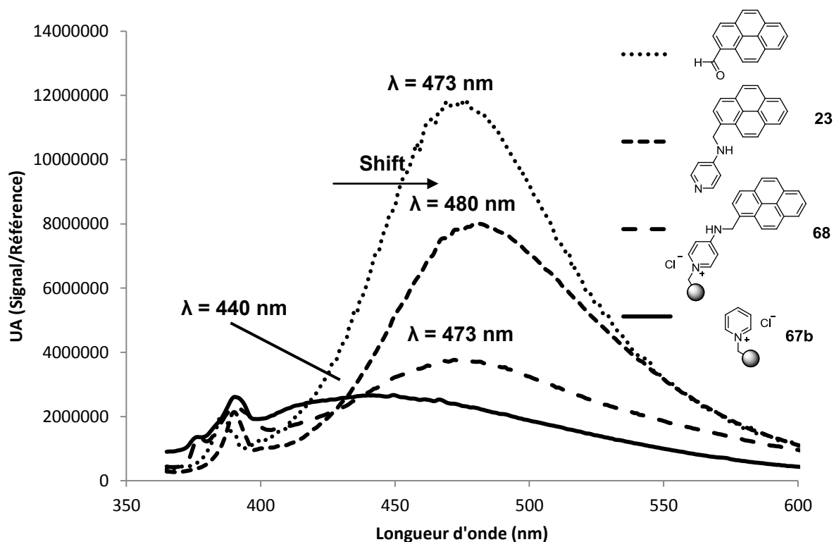
Fig. 89 : Spectres d'émission des composés 23 , 67b , 68 et du 1-pyrènegarboxaldéhyde à l'état solide.
