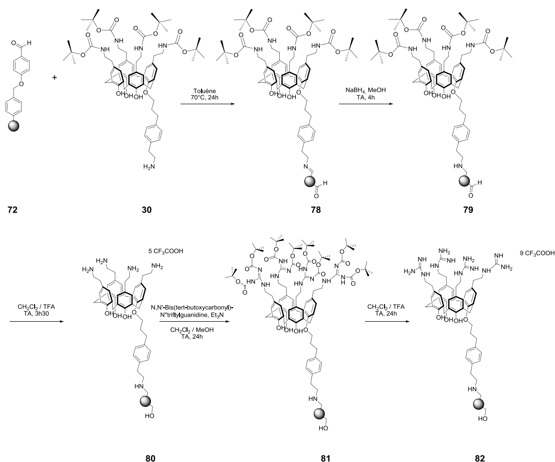
Fig. 116 : Voie de synthèse du calixarène tétra -guanidinium 82 . La structure de la résine de Wang benzaldéhyde ( 72 ) est omise pour plus de clarté.
