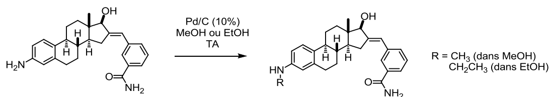
Fig. 96 : Synthèse d'un dérivé anilinoalkyle par utilisation de Pd/C par Poirier et al. 121 .
