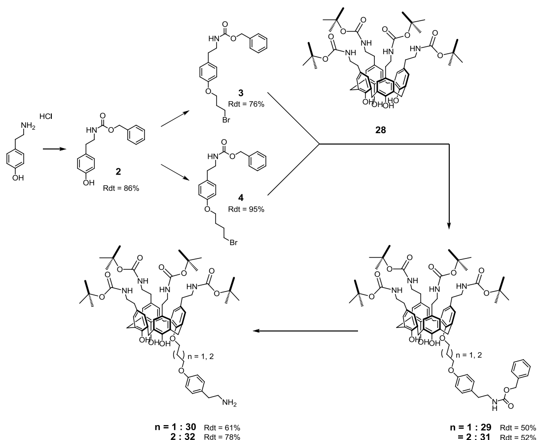
Fig. 64 : Synthèse des deux dérivés calixaréniques 30 et 32 monosubstitués par une tyramine.
