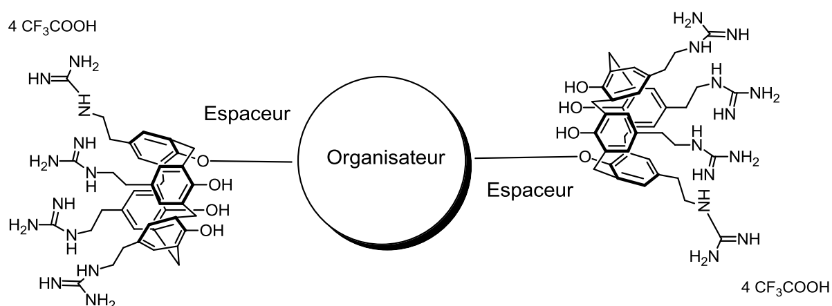
Fig. 126 : Schéma de synthèse de molécules possédant plusieurs têtes poly-guanidiniums.
