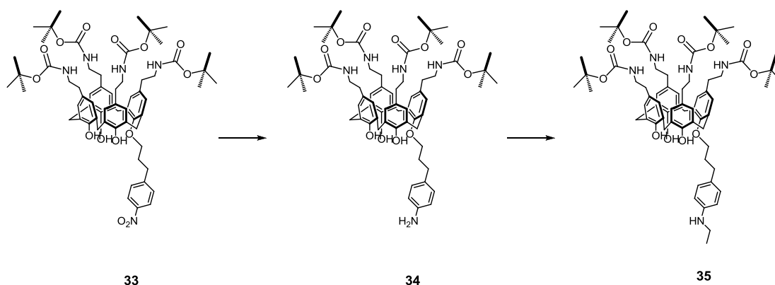
Fig. 94 : Formation du sous-produit de réaction 35 .
