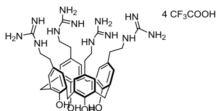
Fig. 54 : Tétra-guanidinoéthylcalix[4]arène ou Cx1 37 .
