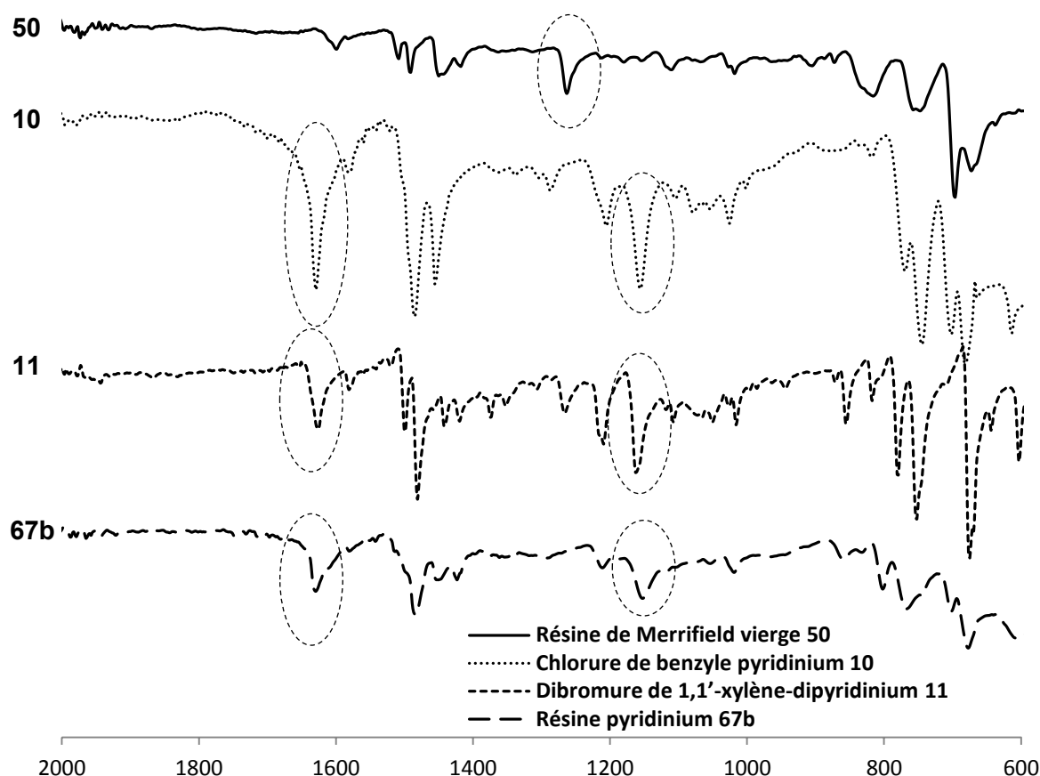
Fig. 76 : Comparaison des spectres infrarouge des résines 50 et 67b avec le chlorure de benzylpyridinium 10 et le dibromure de 1,1'-xylène-bis(pyridinium) 11 .
