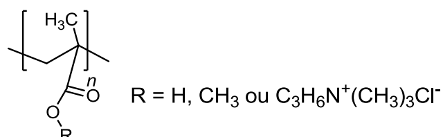
Fig. 44 : Copolymères chargés négativement (H et CH 3 ) ou positivement (C 3 H 6 N + (CH 3 ) 3 Cl) par Gottenbos et al. 78
