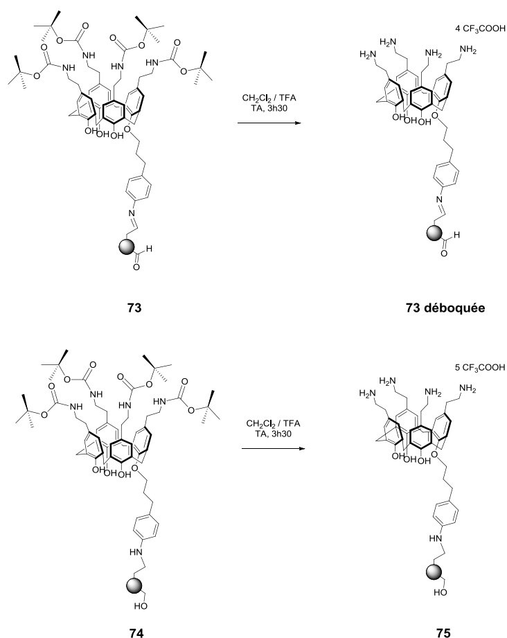
Fig. 115 : Test de la solidité de la liaison imine de la résine 73 en comparaison à celle de la liaison amine de la résine 74 en milieu acide fort.
