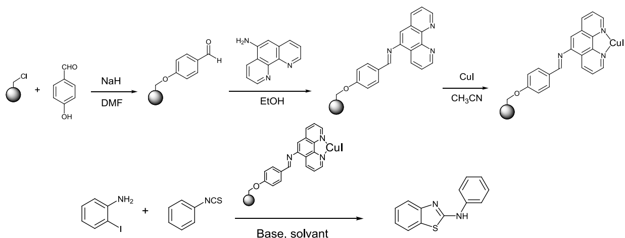
Fig. 24 : Synthèse et utilisation du catalyseur d'iodure de cuivre (I) supporté sur résine de Merrifield par Yang et al. 48 pour la synthèse de benzothiazoles.
