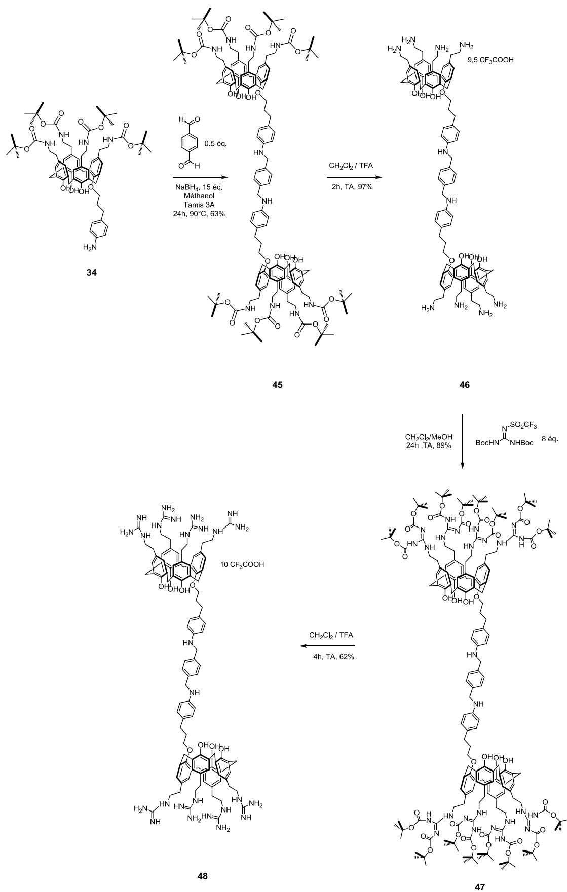
Fig. 127 : Synthèse du bis[tétra-guanidinoéthyl-calix[4]arène] 48 .
