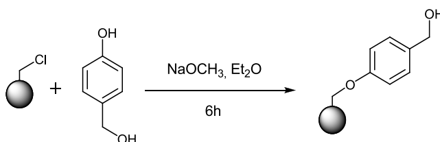
Fig. 27 : Préparation de la résine de Wang à partir de la résine de Merrifield par Su-Sun Wang et al. 50 .
