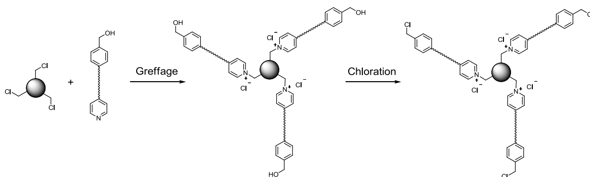
Fig. 79 : Stratégie de synthèse d'une résine de Merrifield possédant des bras d'ancrage plus longs.
