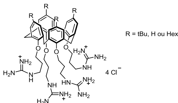
Fig. 15 : Dérivés tétra-guanidiniums calix[4]arènes par Ungaro et al. 33
