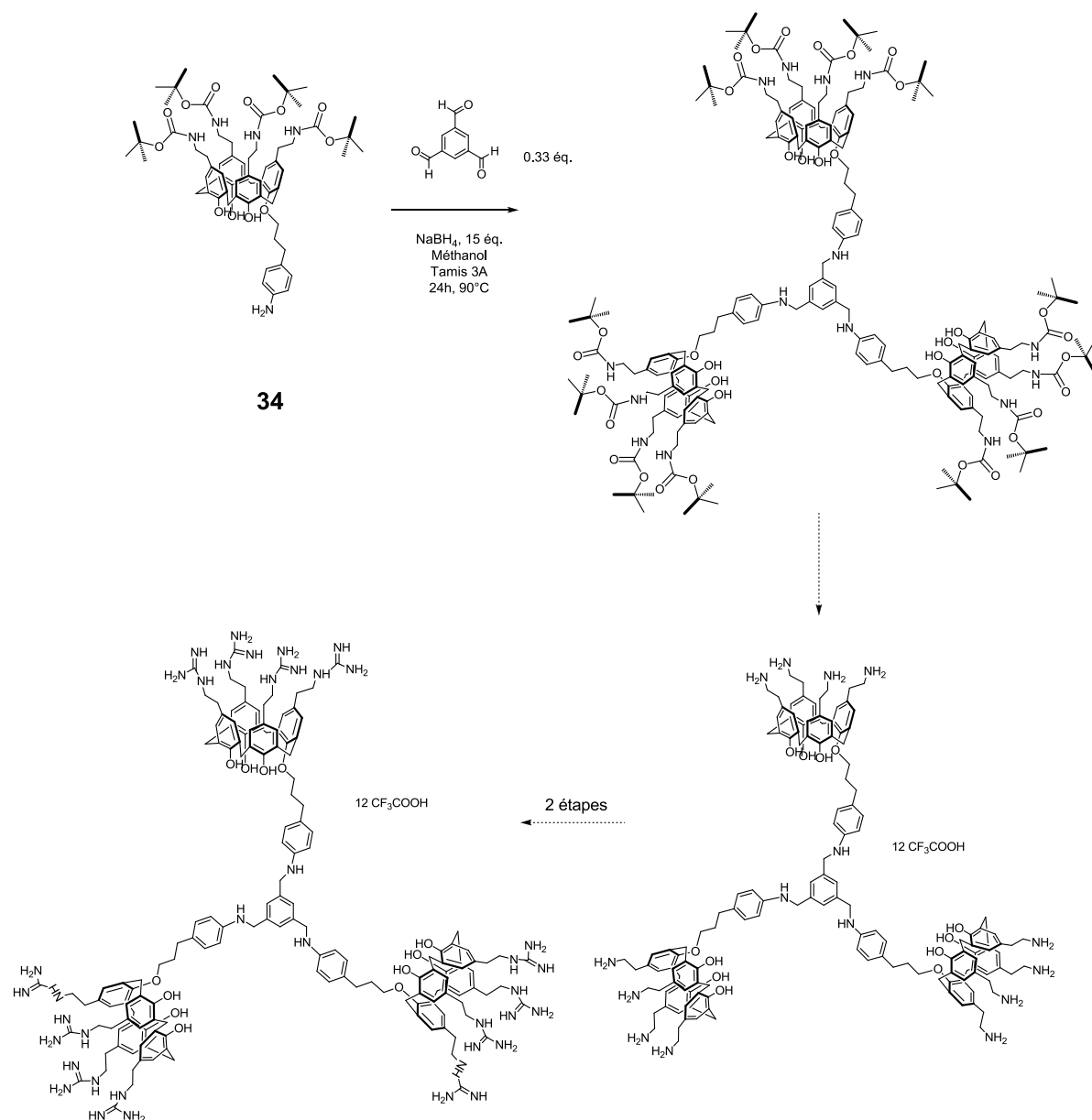
Fig. 128 : Tentative de synthèse du tris-[tétraguanidinoéthyl-calix[4]arène].
