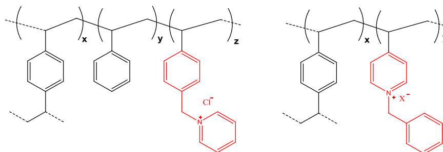
Fig. 33 : Comparaison de la résine pyridinium 67 (à gauche) et de la résine de poly(vinylpyridinium) de Kawabata et al. 59 (à droite).
