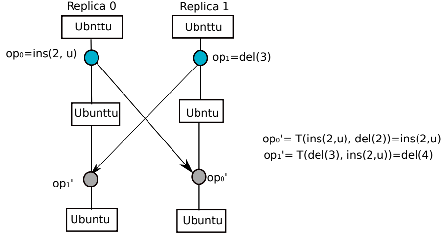
FIGURE 2.7 – Transformées opérationnelles
