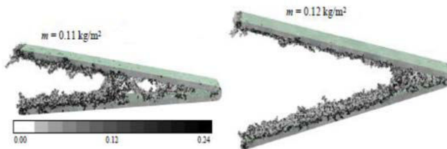
Figure 27 : illustration du dépôt formé dans un pli pour une vitesse de filtration de 50\ \text{cm/s} et des aérosols de 1\ \mu\text{m} de diamètre pour deux pas de plissage différents (Saleh et al. 2014)
