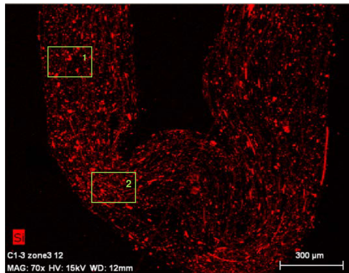
Figure 34 : Vue en coupe de la zone plissée d'un medium. En vert, les zones mesurées. La compacité est de 0,076 dans la zone non affectée (1) et de 0,13 dans la zone comprimée (2)
