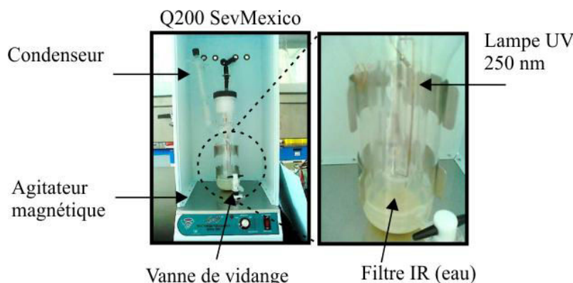
Figure 1. Phtoréacteur utilisé pour la synthèse du système catalytique Ag/ZnO
