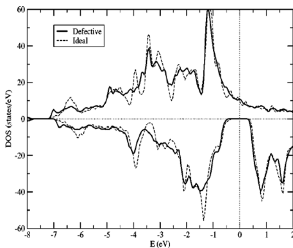
Figure 10 : DOS de \text{Co}_2\text{MnSi} dans la structure idéale (ligne en pointillé) et dans la structure présentant des échanges entre Mn et Si (ligne pleine). La DOS positive correspond aux spins majoritaires et la DOS négative aux spins minoritaires. Figure tirée de Picozzi et al. [43]
