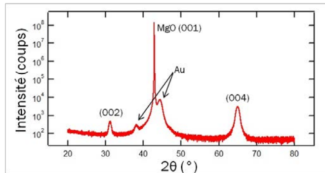
Figure 45: Diffractogramme XRD de Co 1.5 Fe 1.5 Ge le long de la direction [001].
