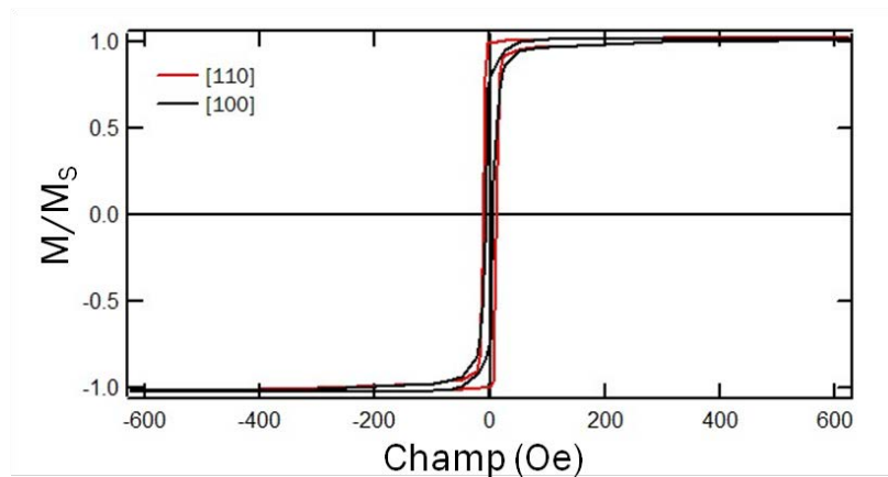
Figure 73 : Cycles d'hystérèse de \text{Co}_2\text{MnSi} le long de la direction [100] et [110].
