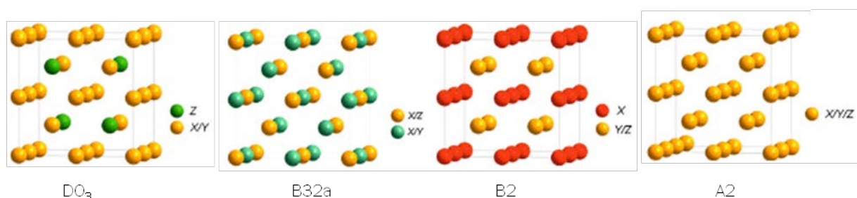
Figure 6: Phases cristallographiques incluant du désordre chimique tirées de Graf et al. [18]
