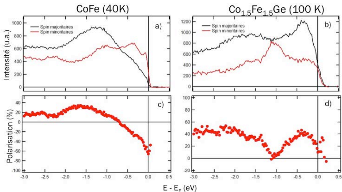
Figure 62 : Spectre de photoémission résolue en spin (en haut) et de polarisation en spin (en bas) pour CoFe à 40 K en a) et c), et \text{Co}_{1.5}\text{Fe}_{1.5}\text{Ge} à 100 K en b) et d).
