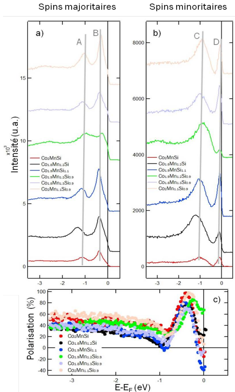
Figure 86 : Densités d'états (DOS) pour les a) spins majoritaires et les b) spins minoritaires pour différents alliages \text{Co}_{2-x-y}\text{Mn}_{1+x}\text{Si}_{1+y} . c) Polarisation en spin des différents alliages \text{Co}_{2-x-y}\text{Mn}_{1+x}\text{Si}_{1+y} .
