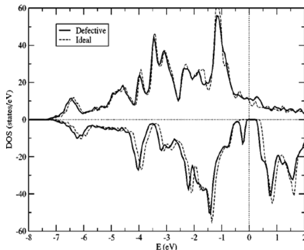
Figure 9 : DOS de \text{Co}_2\text{MnSi} dans la structure idéale (ligne en pointillé) et dans la structure présentant des échanges entre Mn et Co (ligne pleine). La DOS positive correspond aux spins majoritaires et la DOS négative aux spins minoritaires. Figure tirée de Picozzi et al. [43]
