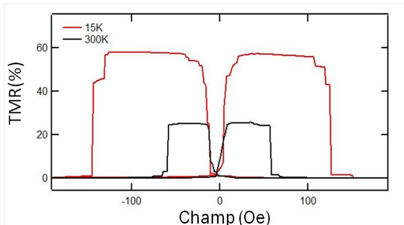
Figure 61 : Courbe de TMR pour CFG/MgO/CFG(001) à température ambiante et à 15 K.
