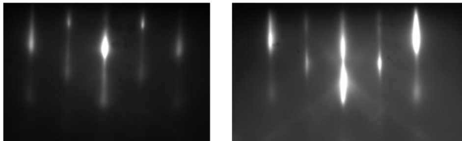
Figure 33: Clichés RHEED du MgO suivant la direction [100] (à droite) et [110] (à gauche) après homoépitaxie du MgO.
