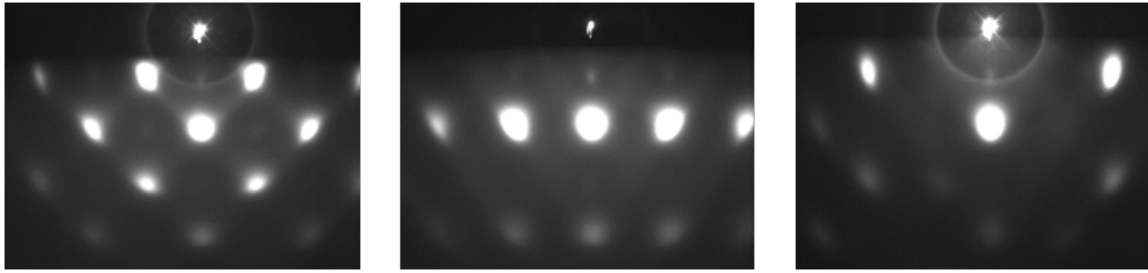
Figure 34: Clichés RHEED de \text{Co}_{1.5}\text{Fe}_{1.5}\text{Ge} de 20 nm dans les trois directions différentes avant recuit. À gauche, la direction [100] , au milieu la direction [110] et à droite la direction [120] .
