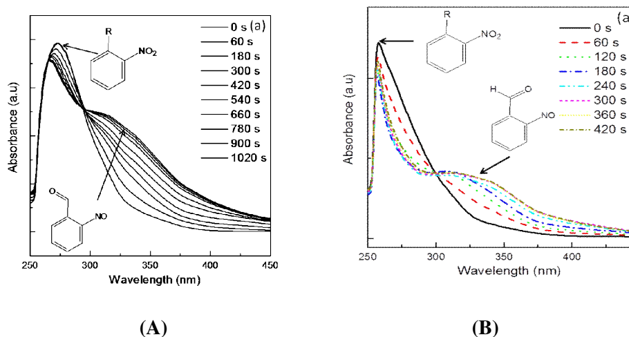
Figure 4. Absorption UV du A) Dex-b-PNBA 9800 et B) Dex(15)-g-12PNBA 9800 pendant l'irradiation dans du DMSO (0.1mg/mL et 0.07 mg/mL, respectivement)) avec une lampe UV équipée d'un filtre de 320 -500 nm (puissance 1150 \text{ mW / cm}^2 ).
