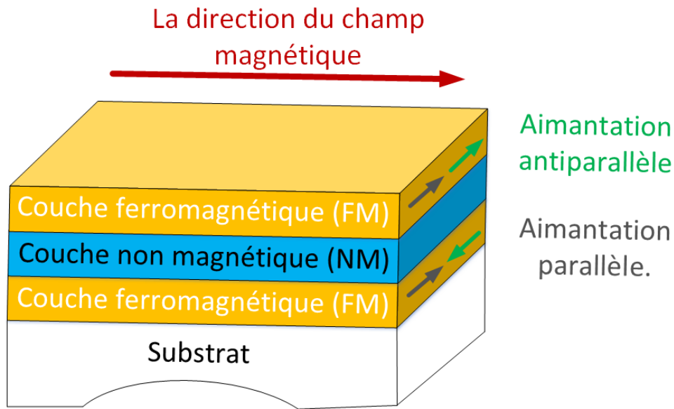
Figure a. Structure de la GMR.
