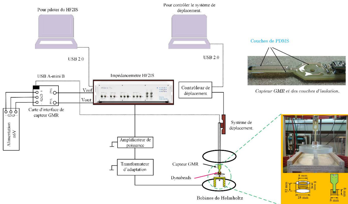
Figure f. Schéma de mesure pour la détection des propriétés magnétiques de Dynabeads.
