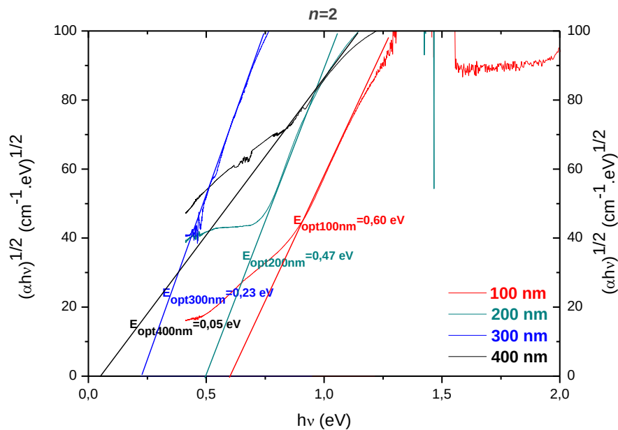
Figure IV-12 : Courbes de Tauc pour une configuration de transition électronique indirecte autorisée ( n=2 ) pour la phase \text{VO}_2 avec des épaisseurs de 100, 200, 300 et 400 nm
