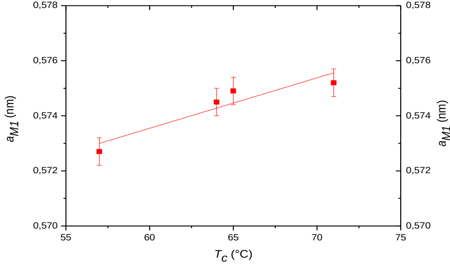
Figure IV-10 : Valeurs du paramètre de maille a_{M1} en fonction de T_c pour la phase \text{VO}_2/\text{SiO}_2 synthétisée sur substrat de verre à température ambiante
