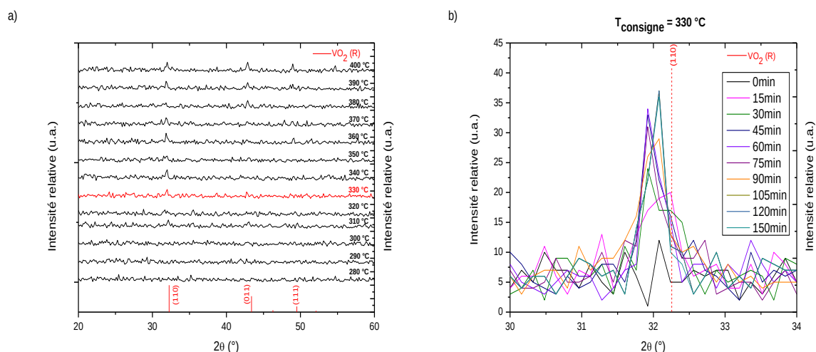
Figure III-14 : Étude de la température de cristallisation de la phase \text{VO}_2/\text{SiO}_2 par diffraction des rayons X (a) (b)
