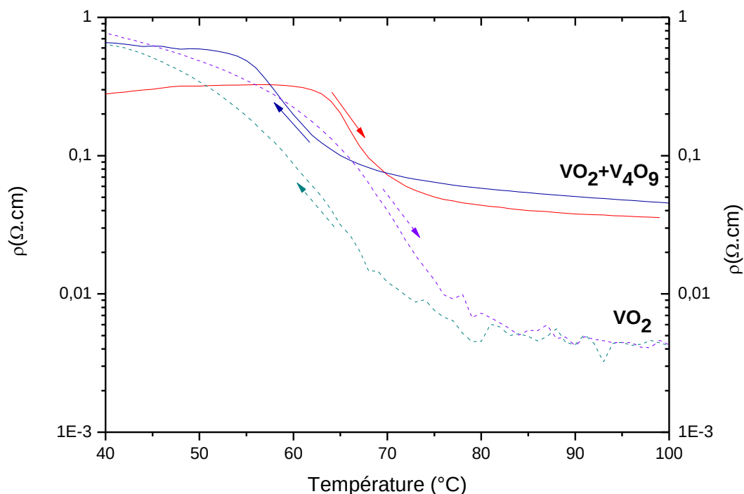
Figure IV-24 : Mesures de résistivité électrique en fonction de la température d'un système biphasé \text{VO}_2/\text{V}_4\text{O}_9 et d'une phase \text{VO}_2 synthétisés sur un substrat de silicium à la température de 500 °C
