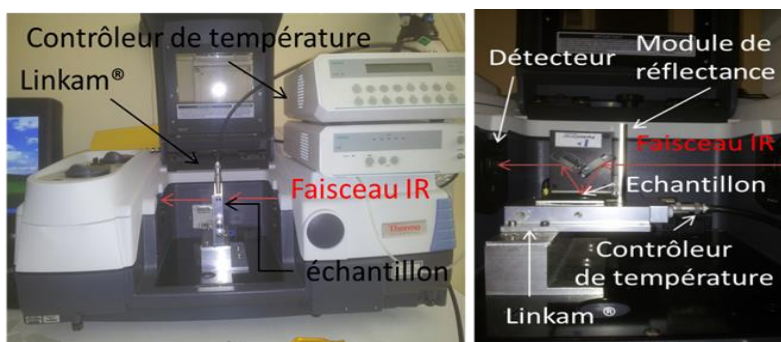
Figure II-17 : Montages du spectromètre FTIR pour les mesures en température de transmittance et de réflectance
