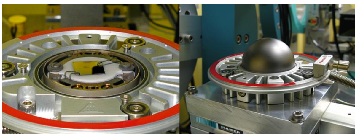
Figure II-10 : Illustrations du four de recuit « DHS1110 » avec la platine chauffante et le dôme en carbone
