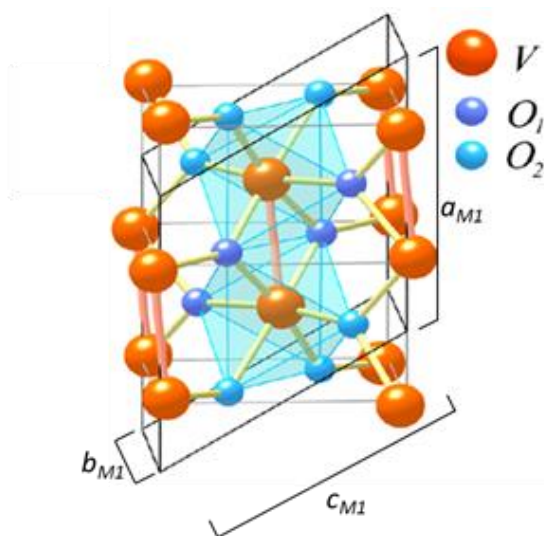
Figure I-8 : Structure monoclinique basse température \text{VO}_2(\text{M1}) [9]
