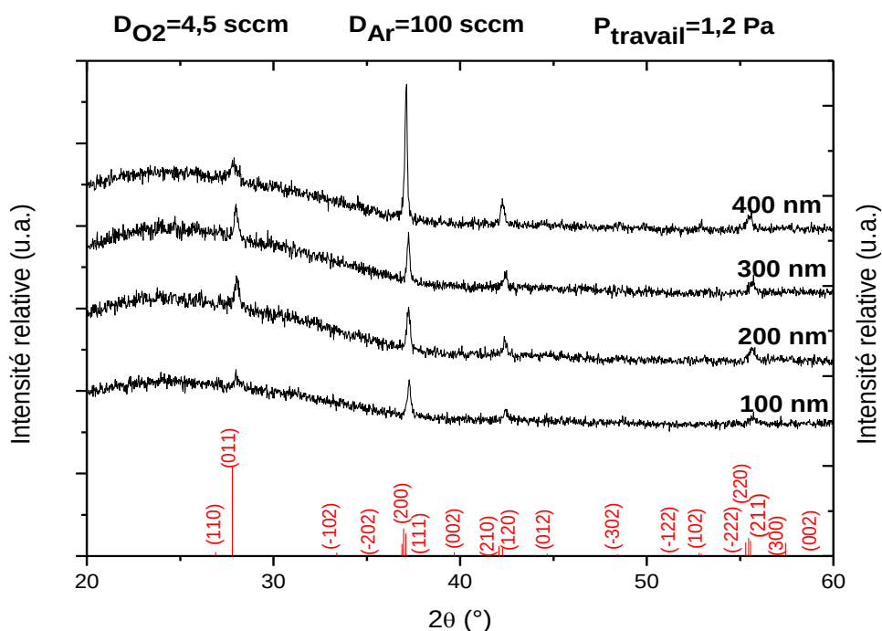
Figure IV-4 : Diffractogrammes des rayons X de la phase \text{VO}_2/\text{SiO}_2 pour quatre épaisseurs de \text{VO}_2 de 100, 200, 300 et 400 nm synthétisées sur substrat de verre après un recuit sous air durant deux heures à la température de 350 °C
