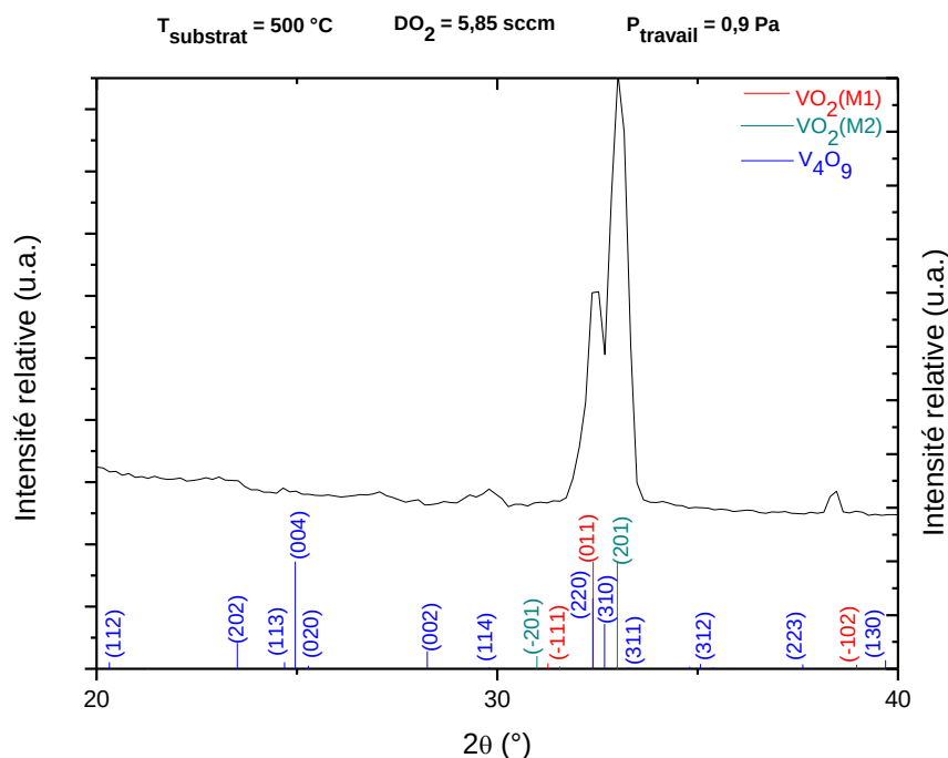
Figure III-22 : Diffractogrammes des rayons X après détecturation d'un système biphasé \text{VO}_2 + \text{V}_4\text{O}_9 synthétisé sur substrat de silicium à la température de 500^\circ\text{C} à 0,9 \text{ Pa}
