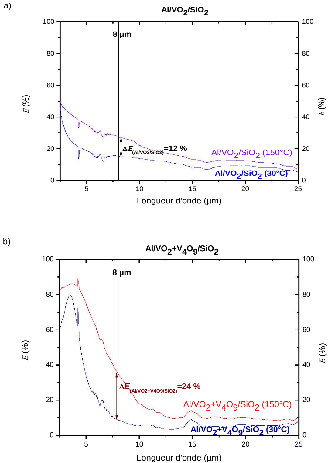
Figure IV-30 : Estimations de mesures d'émissivité infrarouge à 30 et 150 °C en fonction de la longueur d'onde des systèmes \text{Al/VO}_2/\text{SiO}_2 (a) et \text{Al/VO}_2+\text{V}_4\text{O}_9/\text{SiO}_2 (b) avec une épaisseur de \text{VO}_2 de 100 nm synthétisés sur un substrat d'aluminium à température ambiante
