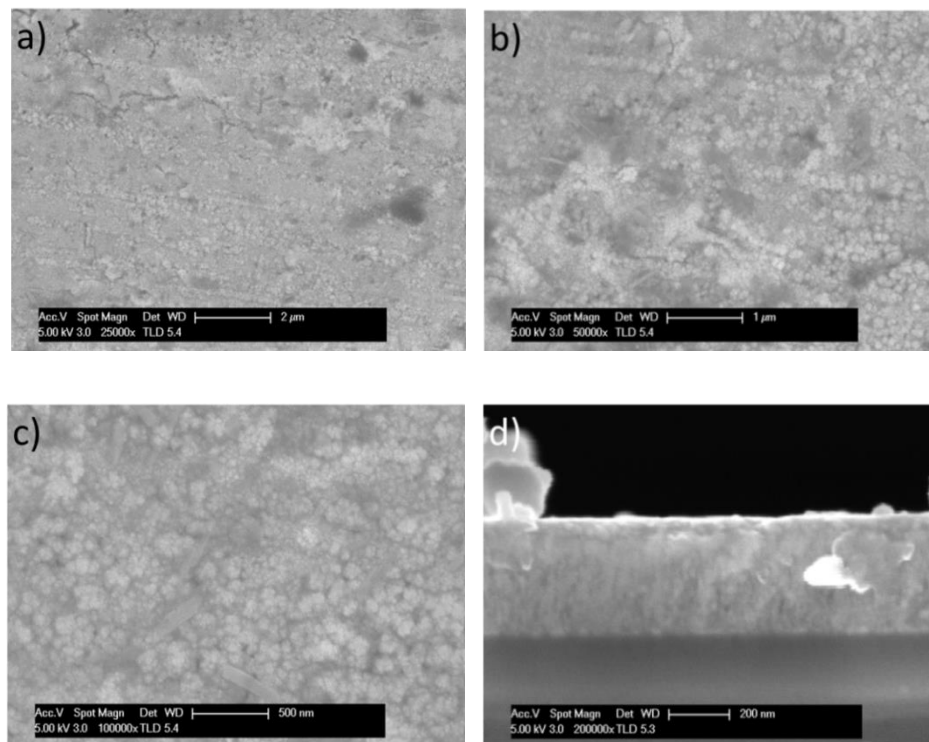
Figure III-13 : Micrographies de la morphologie de surface (a) (b) (c) et coupe transverse (d) de la phase \text{VO}_2/\text{SiO}_2 réalisée sur substrat de verre après recuit sous air à la température de 350^\circ\text{C} durant deux heures
