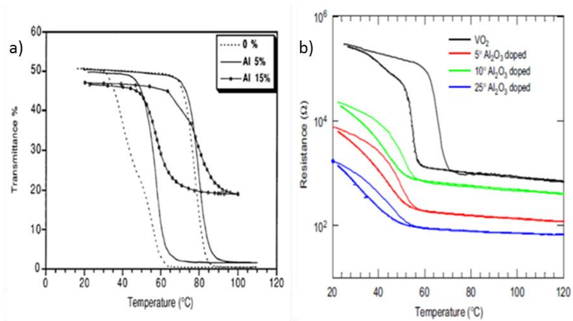
Figure I-29 : Dopage de \text{VO}_2 par de l'Al réalisés par sol-gel (a) [76] et par laser pulsé (b) [75]
