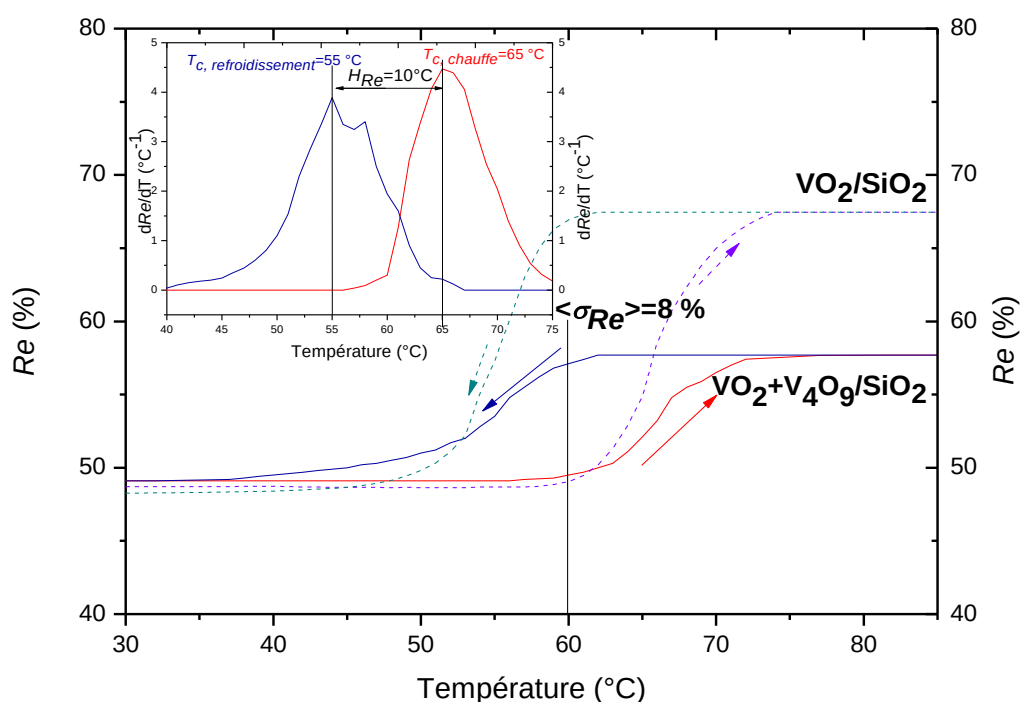
Figure IV-19 : Mesures de réflectance en fonction de la température et dérivées premières des courbes de chauffe et de refroidissement en réflectance par rapport à la température pour une longueur d'onde 8\text{ }\mu\text{m} d'un système biphasé \text{VO}_2+\text{V}_4\text{O}_9/\text{SiO}_2 et une phase \text{VO}_2/\text{SiO}_2 synthétisés sur substrat verre à température ambiante
