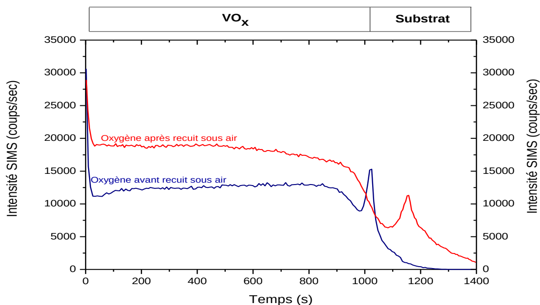
Figure III-10 : Profils de composition en oxygène réalisés sur deux échantillons avant et après un recuit sous air durant deux heures à une température de 350 °C
