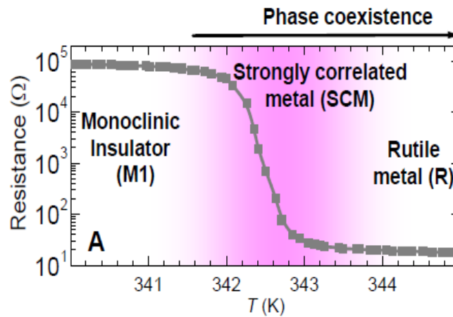
Figure I-11 : Mesures de résistance électrique en fonction de la température d'un film mince de \text{VO}_2 [25]
