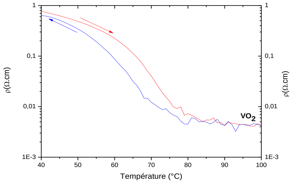
Figure IV-23 : Mesures de résistivité en fonction de la température d'une phase \text{VO}_2 synthétisée sur un substrat de silicium à la température de 500 °C
