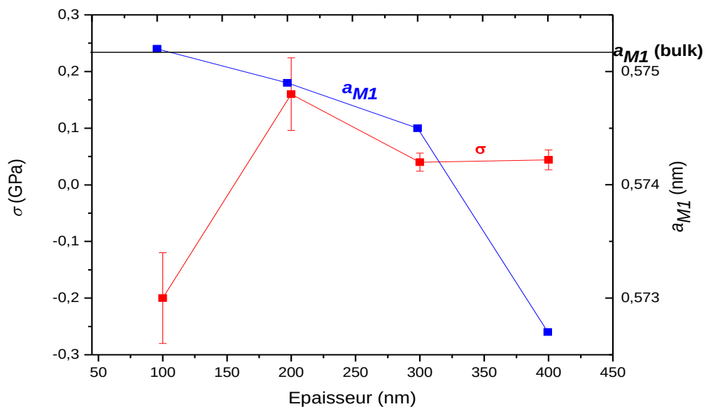
Figures IV-7 : Mesures de contraintes et du paramètre de maille a_{M1} pour quatre épaisseurs de \text{VO}_2
