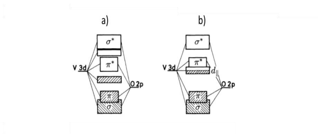
Figure I-17 : Structure de bandes schématique de \text{VO}_2 à basse température avant la transition de phases (a) et à haute température après la transition de phases (b) [32]
