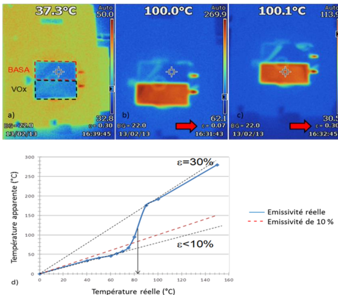
Figure I-3 : Image thermique avec mesure d'émissivité d'un capteur recouvert de la sous-couche sélective (partie « BASA ») à basse température (a), image thermique avec mesure d'émissivité d'un capteur recouvert de la sous-couche sélective (partie « BASA ») à haute température (b), image thermique avec mesure d'émissivité d'un capteur recouvert de la sous-couche sélective et revêtu d'un film mince d'oxyde de vanadium (partie « \text{VO}_x ») dans l'état métallique à haute température (c) et courbe d'émissivité infrarouge en fonction de la température du système couche-sélective/ \text{VO}_x (d)
