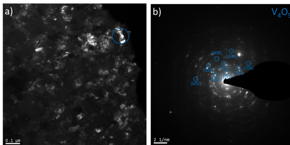
Figure III-24 : Micrographie en champ sombre (a) et cliché de diffraction indexé (b) d'un système biphasé \text{VO}_2 + \text{V}_4\text{O}_9 synthétisé sur substrat de silicium à la température de 500 °C. La zone entourée de bleu sur la figure (a) correspond à la zone sélectionnée pour réaliser le cliché de micro-diffraction présenté sur la figure (b)
