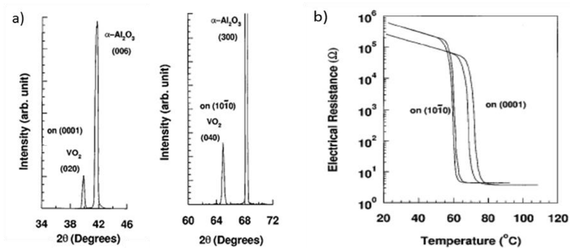
Figure I-22 : Diffractogrammes RX de films minces de \text{VO}_2 synthétisés sur des substrats de saphir orientés (0001) et (10-10) (a) et mesures de résistance en fonction de la température de films minces de \text{VO}_2 synthétisés sur des substrats de saphir orientés (0001) et (10-10) (b)
