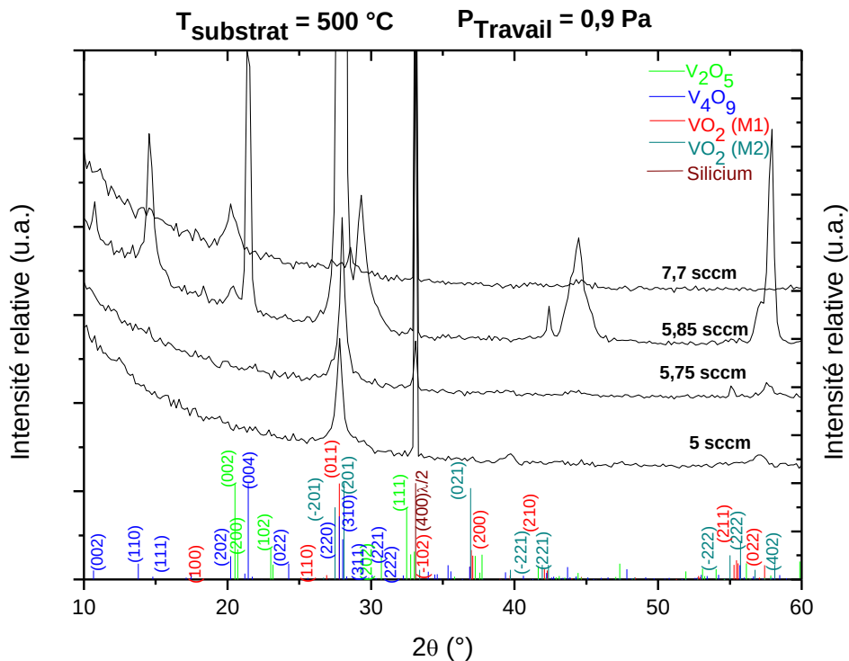
Figure III-19 : Diffractogrammes des rayons X de films de VO 2 purs sur substrat de silicium synthétisés à la température de 500 °C pour différents débits d'O 2
