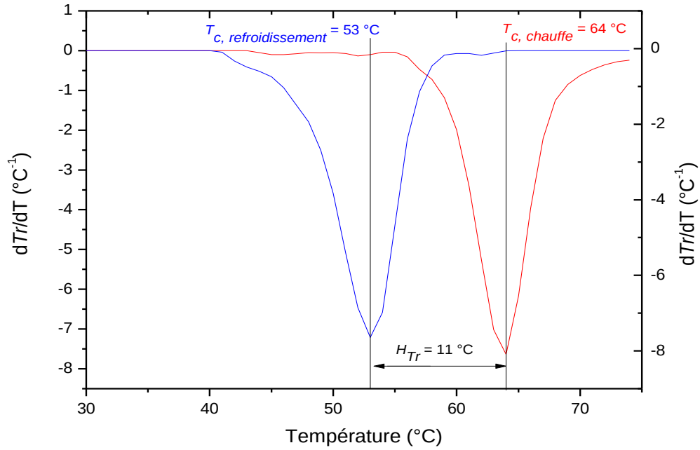
Figure IV-3 : Dérivée première des courbes de chauffe et de refroidissement en transmittance par rapport à la température pour une longueur d'onde 2,5 µm de la phase VO 2 /SiO 2 synthétisée sur substrat de verre à température ambiante
