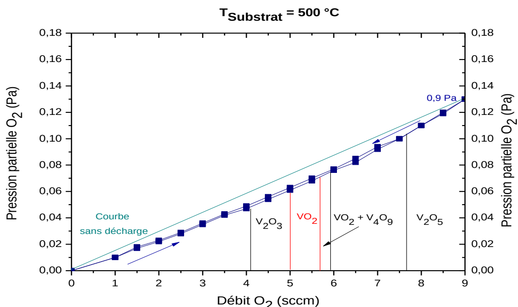
Figure III-17 : Étude de la pression partielle en oxygène en fonction du débit d' \text{O}_2 pour une température de 500^\circ\text{C} et une pression de travail de 0,9 Pa et domaines de synthèse des différentes phases d'oxydes de vanadium obtenus après analyses DRX
