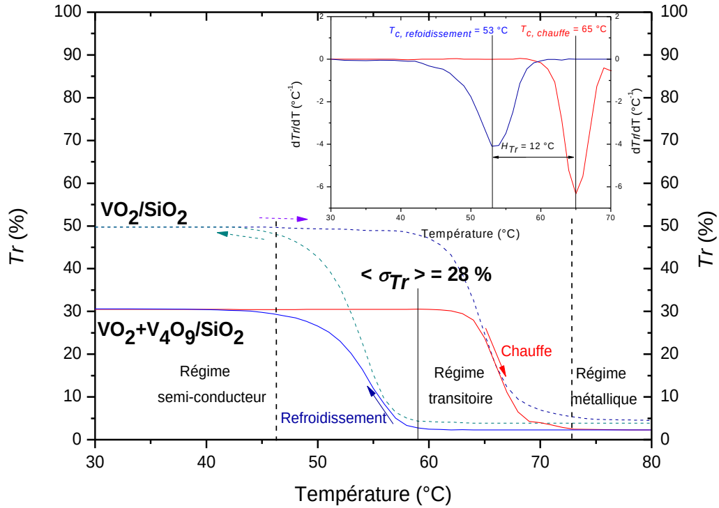
Figure IV-15 : Mesures de transmittance pour une longueur d'onde 2,5\text{ }\mu\text{m} en fonction de la température pour un système biphasé \text{VO}_2+\text{V}_4\text{O}_9/\text{SiO}_2 et pour une phase \text{VO}_2/\text{SiO}_2 synthétisés sur substrat de verre à température ambiante
