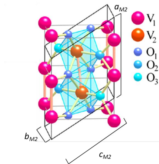
Figure I-10 : Structure monoclinique base centrée basse température \text{VO}_2(\text{M2}) [9]
