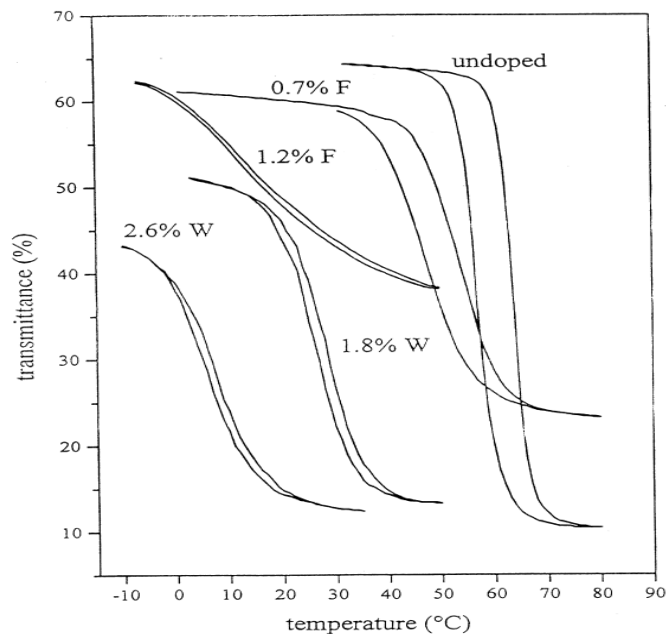
Figure I-30 : Mesures de transmittance en fonction de la température de films minces de \text{VO}_2 dopés avec différents pourcentages atomiques de W et de F [78]
