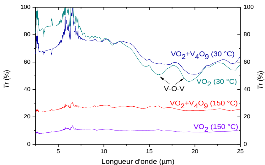
Figure IV-27 : Mesures de transmittance à 30 et 150 °C en fonction de la longueur d'onde pour une phase \text{VO}_2 et un système biphasé \text{VO}_2+\text{V}_4\text{O}_9 synthétisés sur substrat de silicium à la température de 500 °C
