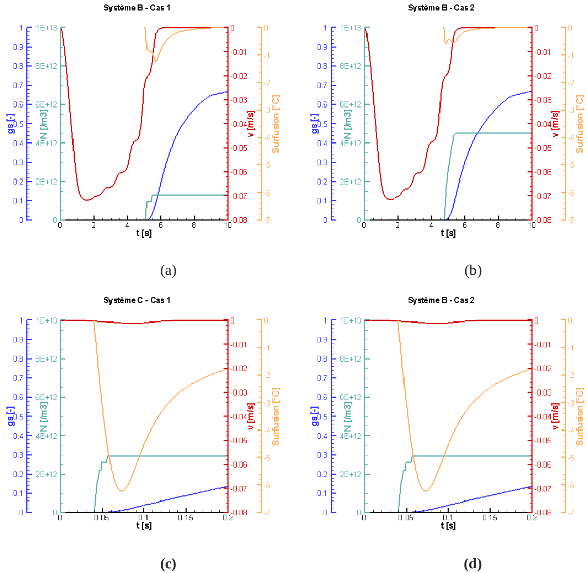
Figure 3- 49 : Evolution avec le temps de la fraction solide g_s [-], la densité de grains N [/m³], la vitesse verticale intrinsèque de la phase liquide v [m/s] et la surfusion [°C] à mi-hauteur de la paroi refroidie ((x,y)=(0,37)\text{mm}) pour le Système B ((a) et (b)) et pour le système C ((c) et (d)).
