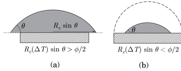
Figure 1- 5 : Schéma de germination hétérogène dans le cas \left| \frac{\gamma_{il} - \gamma_{is}}{\gamma_{sl}} \right| \leq 1 : (a) le rayon de la particule affinant \phi/2 est trop faible pour qu'il y ait germination à la surfusion donnée et (b) le rayon est suffisant- tiré de (Dantzig J.A. 2009).
