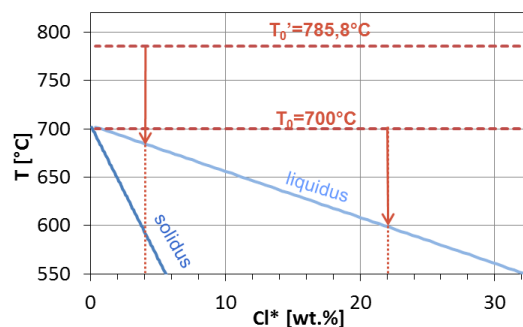
Figure 3- 45 : Diagramme de phases Al-Cu avec les différents systèmes étudiés: système A (22wt.%Cu et T_0=700^{\circ}\text{C} ), système B (4wt.%Cu et T_0'=785,8^{\circ}\text{C} ) et système C (4wt.%Cu et T_0=700^{\circ}\text{C} )
