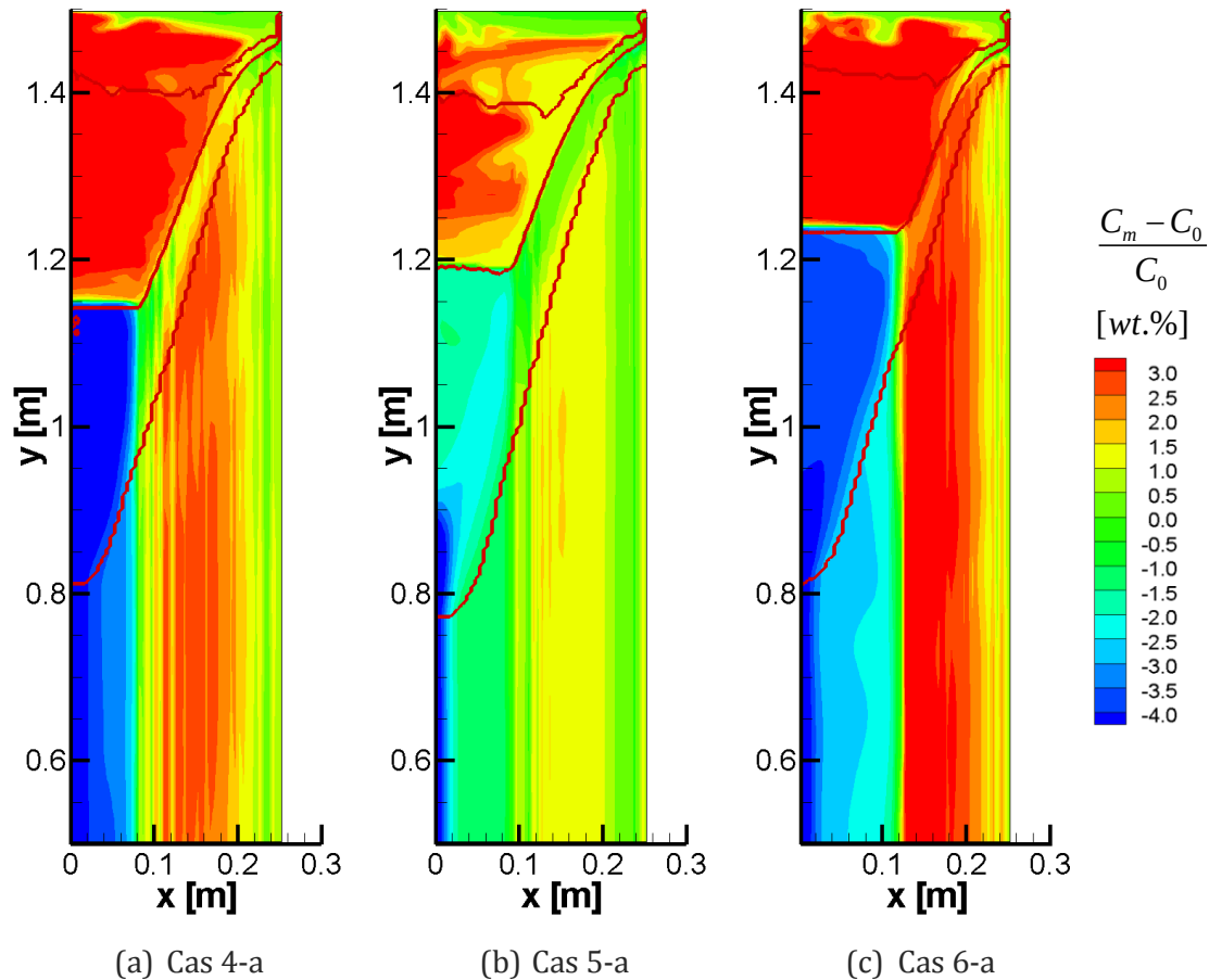
Figure 4- 41 : Carte de composition relative en soluté et position des liquidus et solidus (en rouge) pour (a) Cas 4-a, (b) Cas 5-a et (c) Cas 6-a ( g^{loc}=0,3 ).
