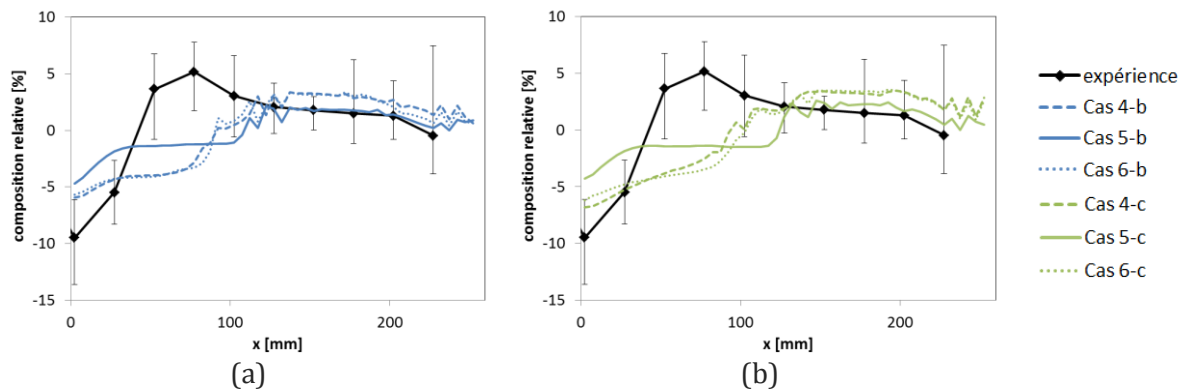
Figure 4- 45 : (a) Profil de composition relative en soluté pour le Cas 4, le Cas 5 et le Cas 6 pour (a) g_{\text{bloc}}=0,4 et (b) g_{\text{bloc}}=0,5 , ainsi que les résultats expérimentaux.
