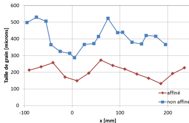
Figure 1- 30 : Profil expérimental de taille finale de grains selon l'épaisseur x à z=450mm dans le cas non affiné et le cas affiné- tiré de (Daloz D. 2002)
