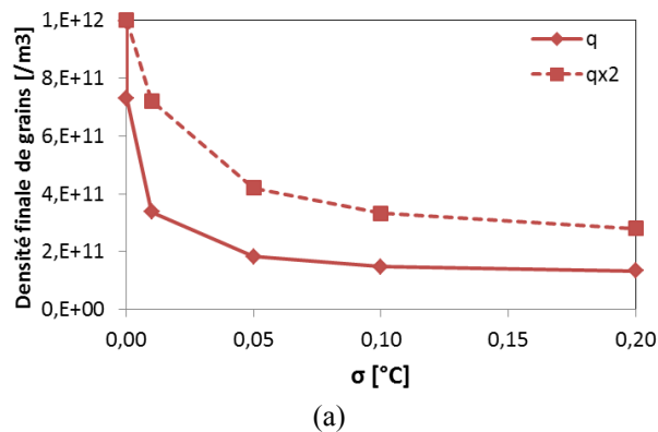
Figure 3- 6 : Impact de l'écart type de la distribution de germes sur la densité finale de grains pour le modèle de croissance globulaire pour le refroidissement initial ( q=4.10^6 W/m 3 ) et pour un refroidissement deux fois plus important.
