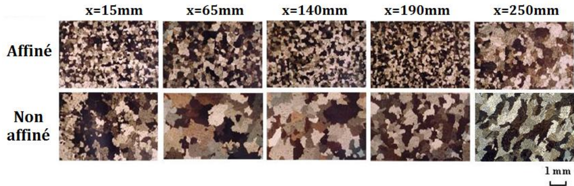
Figure 4- 20 : Microstructure selon la distance au centre, pour les cas affiné et non affiné – tiré de (Joly A. 2000).
