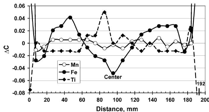
Figure 1- 28 : Alliage 2024, vitesse de coulée 120 mm/min, Profil de ségrégation des éléments Mn, Fe et Ti ( \Delta C(\text{Ti}) divisé par 10) – (E. D. Nadella R. 2008)
