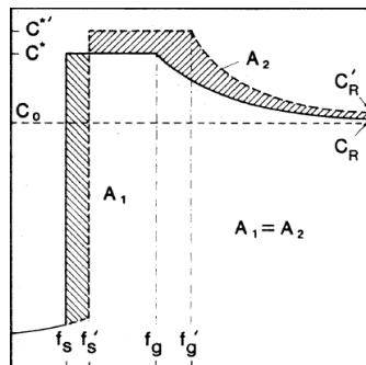
Figure 1- 16 : Profil de concentration en soluté à t et t+dt d'après le modèle de M. Rappaz et Ph. Thévoz (T. P. Rappaz M. 1987).
