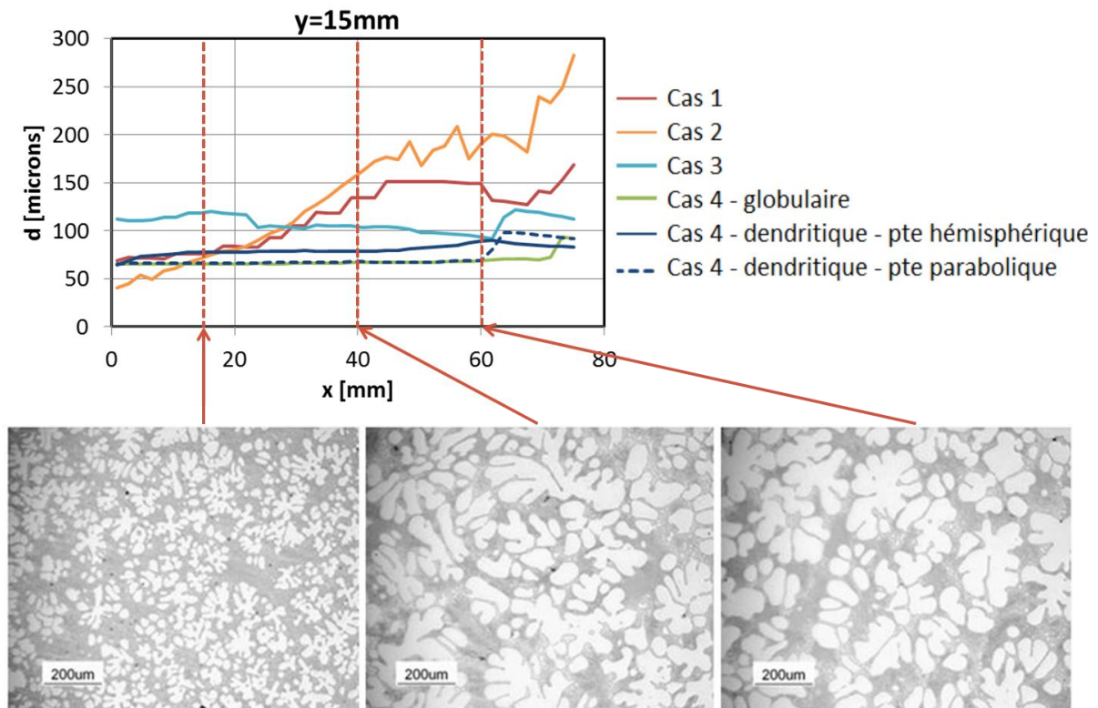
Figure 3- 33 : Comparaison du profil de taille finale de grain obtenu par le modèle pour les différents cas à y=15\text{mm} aux micrographes obtenus par l'expérience à cette même hauteur en trois abscisses : x=15\text{mm} , 40\text{mm} et 60\text{mm} .
