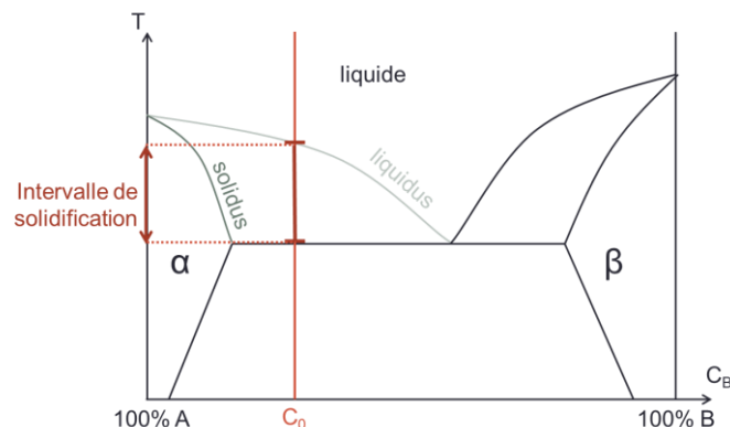
Figure 0- 2 : Représentation schématisée d'un diagramme de phase dans le cas d'un alliage binaire.
