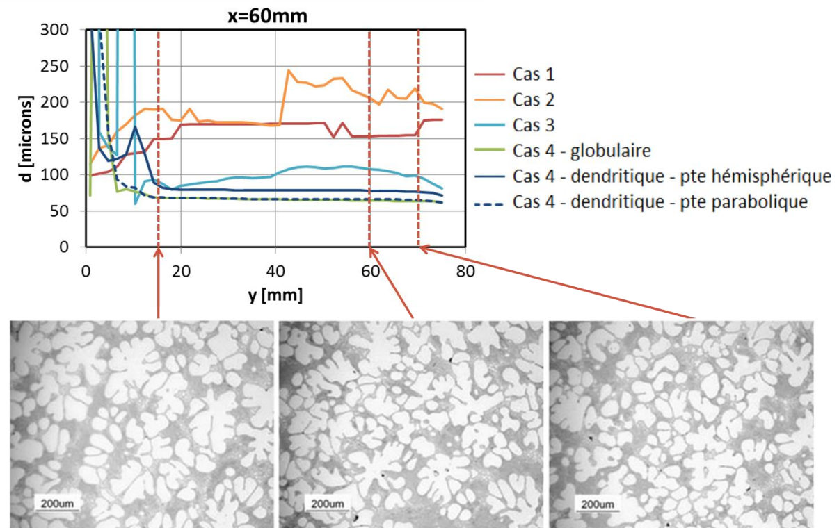
Figure 3- 34 : Comparaison du profil de taille finale de grain obtenu par le modèle pour les différents cas à x=60\text{mm} aux micrographes obtenus par l'expérience à cette même abscisse à trois hauteurs : y=15\text{mm} , 60\text{mm} et 70\text{mm} .
