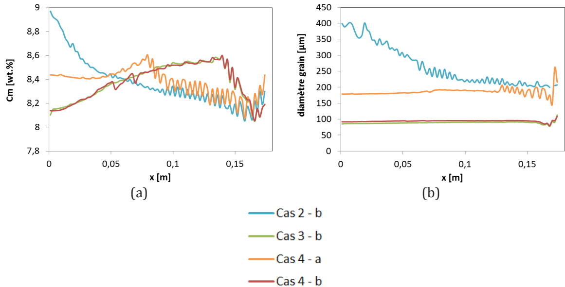
Figure 4- 16 : (a) Profil de composition en soluté et (b) profil de diamètre de grain, dans les cas avec mouvement des germes : pour le Cas2-b sans mouvement des grains, et les Cas 3 et 4 avec mouvement des grains (Cas3-b : grains globulaires, Cas4-a : grains dendritiques et V_{pointe} hémisphérique et Cas4-b : grains dendritiques et V_{pointe} paraboloidale).
