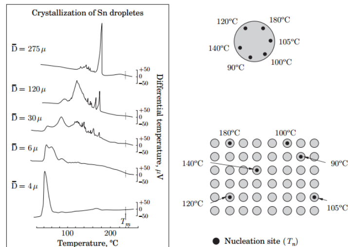
Figure 1- 4 : Spectre d'analyse thermique différentielle obtenu sur des gouttes d'étain (Perepezko J.H. 1996) et schéma illustrant l'isolement des particules affinantantes lors de la diminution de taille des gouttes – tiré de (Dantzig J.A. 2009).
