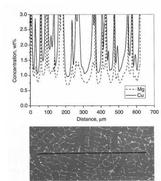
Figure 1- 25 : Microségrégation mesurée sur 700μm sur un échantillon prélevé au centre d'une billette de 200mm de diamètre coulée à 80mm/min pour un alliage de type 2024 – issu de (Eskin D.G. 2008).
