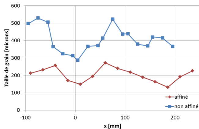
Figure 4- 21 : Profil expérimental de taille finale de grains selon l'épaisseur x à z=450\text{mm} dans le cas non affiné et le cas affiné- tiré de (Daloiz D. 2002)
