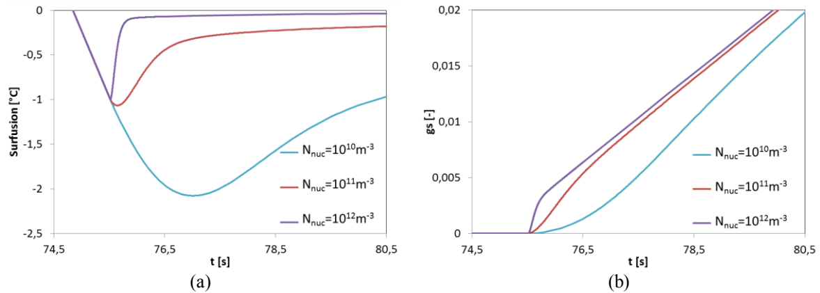
Figure 3- 3 : Evolution (a) de la surfusion et (b) de la fraction solide avec le temps pour trois densités de germes N_{nuc} , activées -1^{\circ}\text{C} de surfusion (modèle de croissance globulaire).
