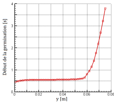
Figure 3- 43 : Profil vertical de l'instant de début de germination le long de la paroi refroidie, pour T_{\text{ext}}=440^{\circ}\text{C} pour le Cas 2.
