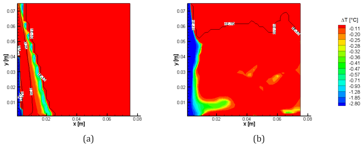
Figure 3- 20 : Carte de surfusio n et isolignes de fraction solide en noir après 30s pour (a) Cas 1 et (b) Cas 3 (les cartes pour les Cas 2 et Cas 4 ne sont pas données car elles sont très proches respectivement des Cas 1 et Cas 3). Les intervalles de surfusio n choisis correspondent à la surfusio n d'activation des classes de germes ( \Delta T_c^i ).
