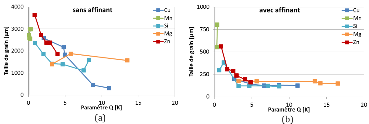
Figure 1- 21 : Taille de grain en \mu\text{m} en fonction du paramètre Q, pour différents solutés, a) sans et b) avec affinage par 10kg/t de Al-5Ti-1B – données issues de [Spittle J.A. 1995].
