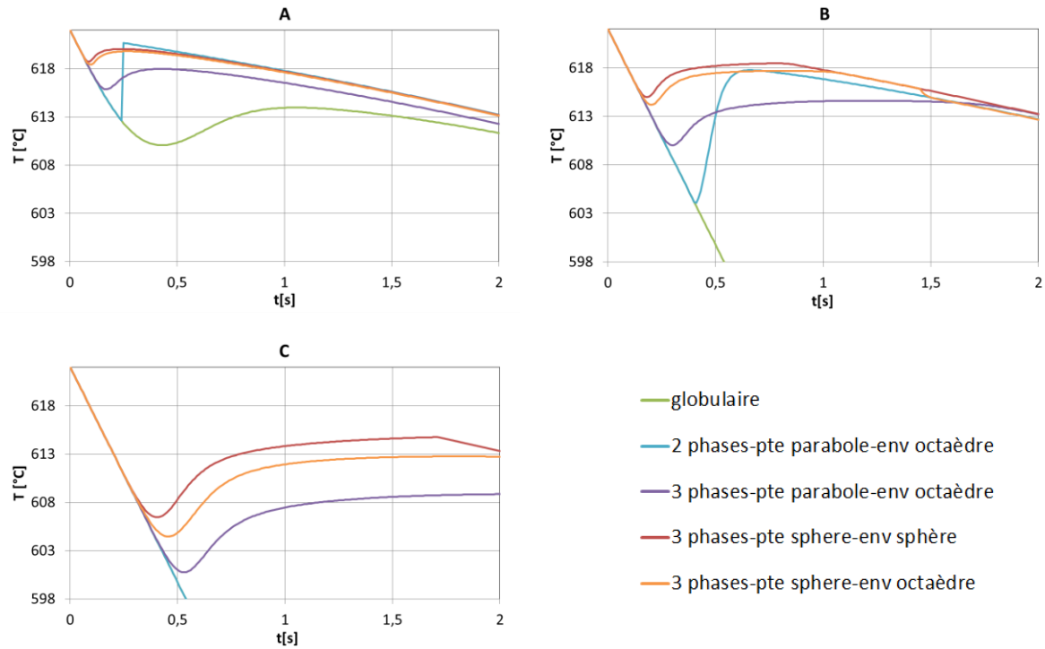
Figure 2- 19 : Evolution de la température obtenue par 5 modèles de croissance pour un cas 0D, pour l'alliage Al-5wt.%Si, refroidi à dT/dt=45\text{K/s} , pour trois tailles finales de grain : A-0,1mm, B-1mm et C-10mm (tous les germes sont activés au liquidus).
