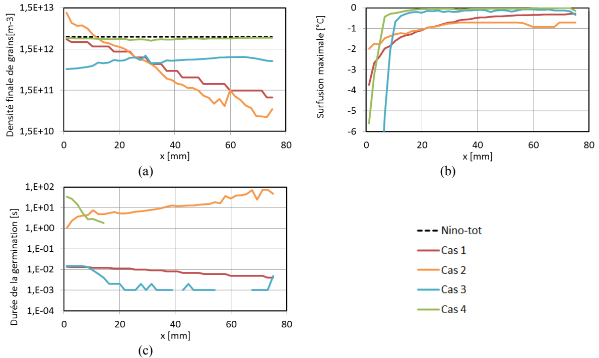
Figure 3- 19 : Profils horizontaux à mi-hauteur ( y=37\text{mm} ) pour les cas 1 à 4 (a) densité finale de grains, (b) surfusio n maximale atteinte, (c) durée de la germination (les lignes sont coupées lorsque la germination n'a localement pas lieu). La ligne en pointillés dans la figure (a) notée Nino-tot indique la somme de toutes les classes de germes de la distribution initiale.
