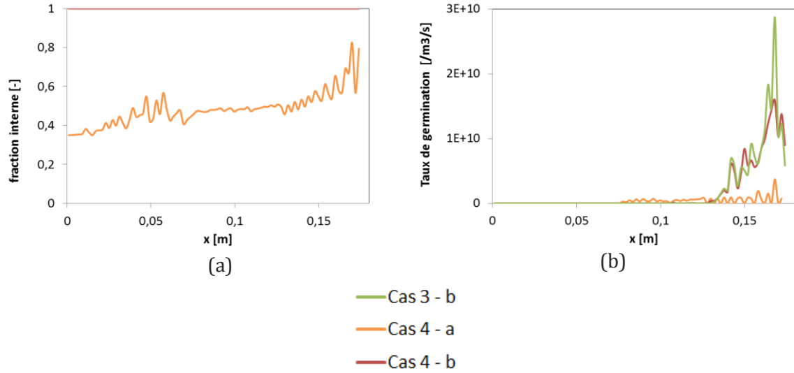
Figure 4- 15 : (a) Profil de fraction interne ( g_i = g_s / g_{env} ) au moment du blocage des grains ( g_{env} = 0,3 ) et (b) profil de taux de germination, pour le Cas 3-a (grains globulaires), le Cas 4-a ( V_{pointe} hémisphérique) et le Cas 4-b ( V_{pointe} paraboloidale).
