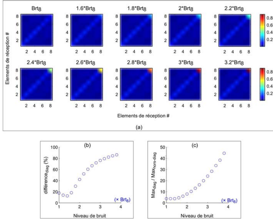
FIGURE 4.8 – (a) Matrices de covariance calculées après des dégradations du bruit de l'antenne #8 ; ces dégradations sont d'amplitudes peu élevées. (b) Évolution des différences au seins des termes diagonaux pour ces dégradations. (c) Évolution du rapport entre les termes diagonaux et les termes hors-diagonaux pour ces dégradations.
