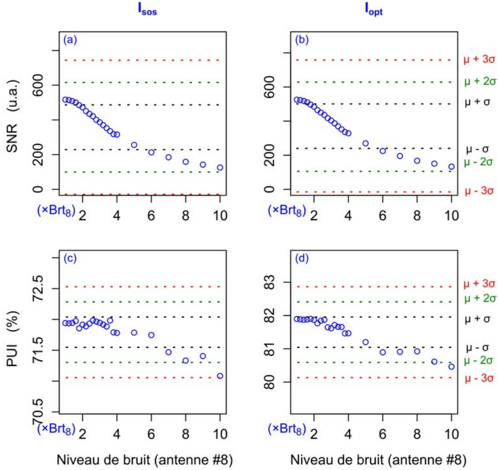
FIGURE 4.10 – Courbe d'évolution des métriques de contrôle en fonction de l'augmentation du bruit acquis par l'antenne #8, pour les images reconstruites suivant la technique I_{\text{sos}} (a,c) et suivant I_{\text{opt}} (b,d).
