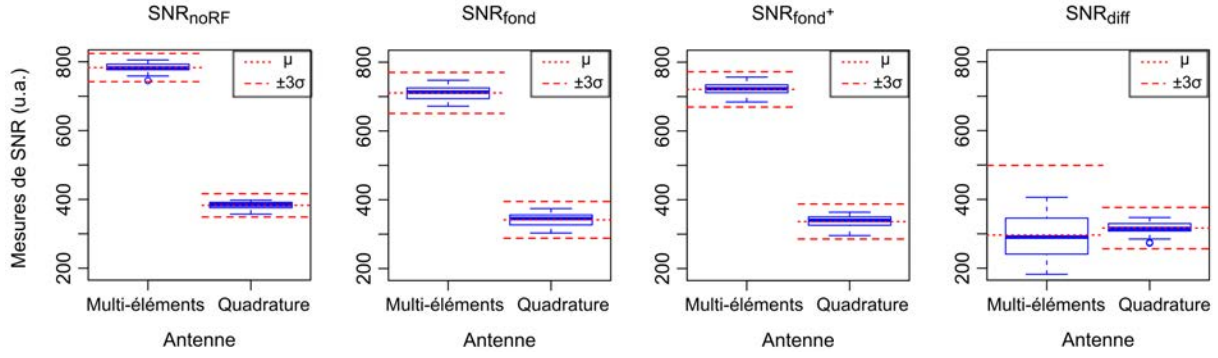
FIGURE 3.5 – Représentation graphique des mesures de SNR réalisées pour les deux types d'antenne suivant les quatre différentes techniques de calcul.
