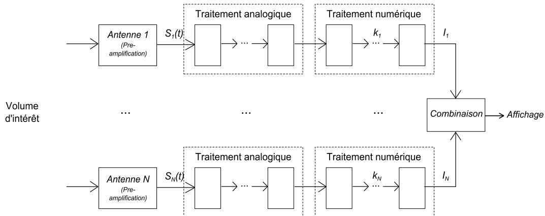
FIGURE 1.9 – Schéma du système de réception et de traitement du signal pour une antenne multi-éléments
