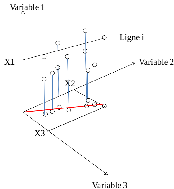
Figure 23 Présentation d'un nuage de points dans un espace de trois dimensions
