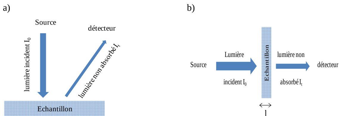
Figure 13 principe de mesure a) en réflexion b) en transmission
