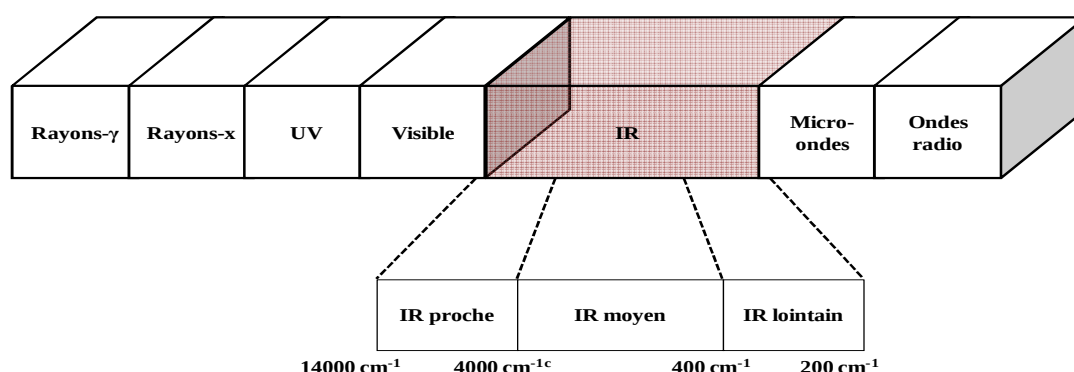
Figure 11 le spectre électromagnétique
