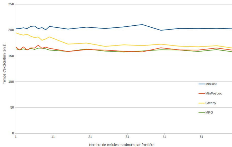
FIGURE 7.5 – Impact de la taille des groupes sur les performances des algorithmes MinDist , MinPos (MinPosLoc), Glouton ( Greedy ) et MPG sur l'environnement bureau avec 5 robots
