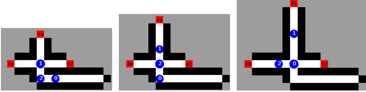
FIGURE 2.6 – Coordination implicite : trois robots sortent d'un couloir exploré et se répartissent de manière équilibrée dans les trois couloirs. Les frontières sont de couleur rouge, les robots de couleur bleu. Chaque robot se dirige vers la frontière la plus proche de lui.
