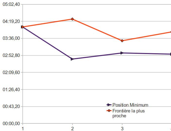
FIGURE 9.2 – Résultat des expériences d’exploration de l’arène en faisant varier le nombre de robots de 1 à 4 (moyenne sur 4 expériences). L’unité en ordonnée est le temps en minutes et secondes et en abscisse le nombre de robots
