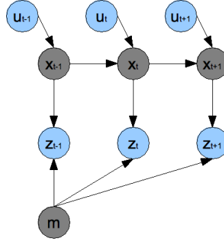
FIGURE 8.6 – SLAM, en bleu les variables observées et en gris les variables cachées
