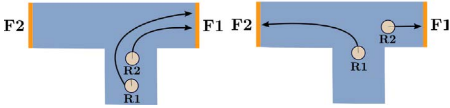
FIGURE 4.11 – Deux robots se séparant sur une intersection en T avec l'algorithme MinPos .
