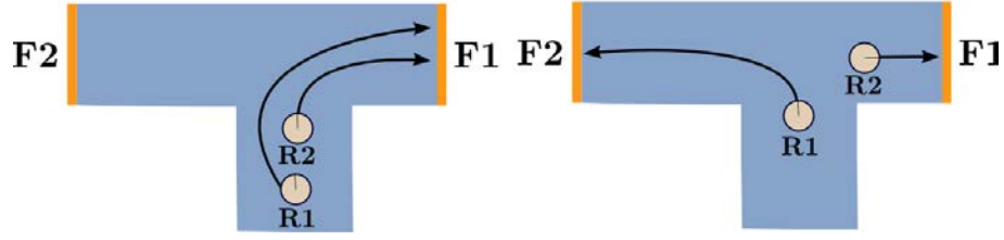
FIGURE 5.11 – Deux robots se séparant sur une intersection en T avec l'algorithme MinPos .
