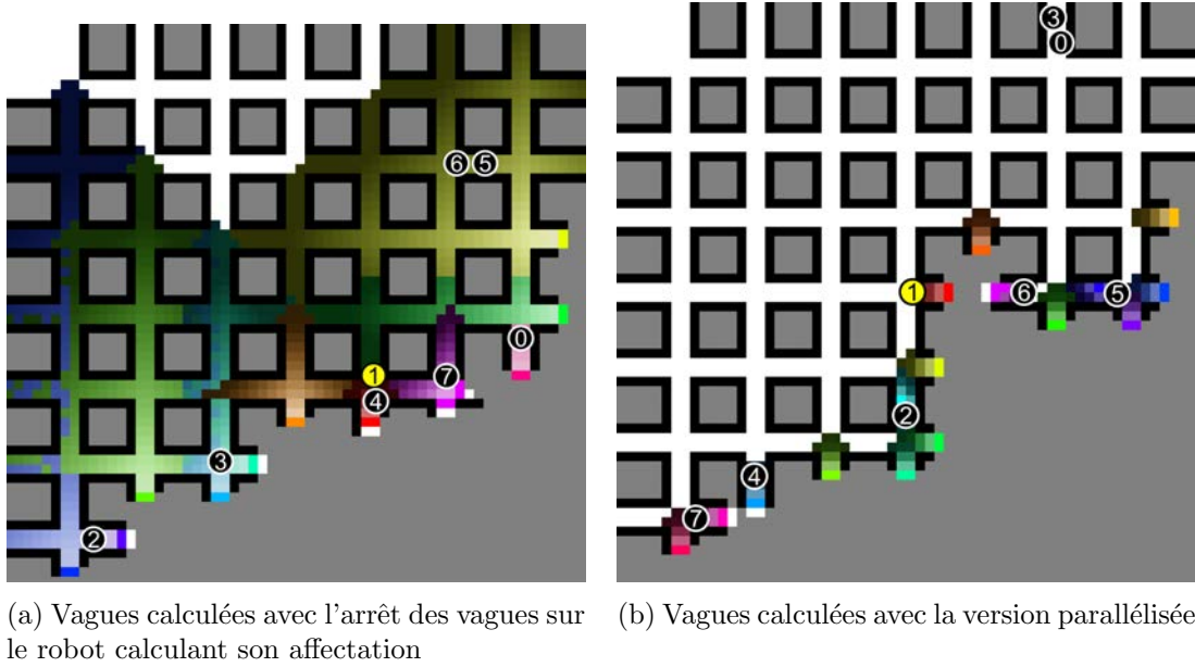
FIGURE 6.10 – Comparaison de l'implémentation de MinPos avec l'arrêt des vagues sur le robot qui calcule son assignation et la version parallélisée.
