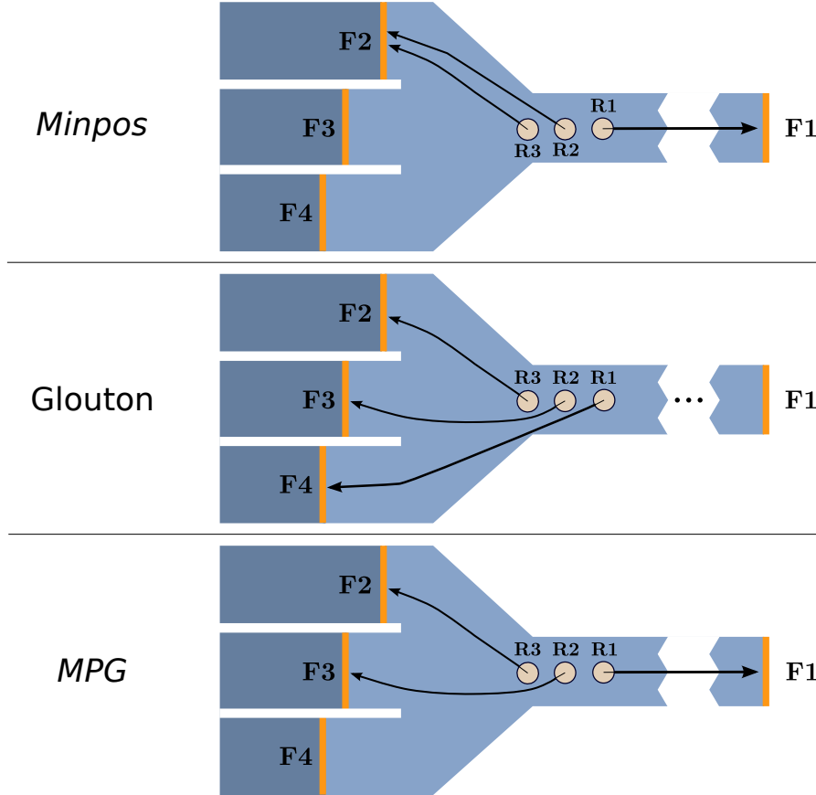
FIGURE 4.13 – Comparaison des assignations MinPos (en haut) Glouton (au centre) et MPG (en bas).
