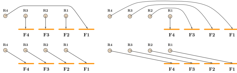
FIGURE 10.1 – Détection des groupes de robots pouvant échanger leur frontière pour améliorer les performances. Le robot R4 est en quatrième position vers la F1 qui lui est affectée. Un échange de frontière entre les robots ( R1 , en 1 re position vers F1 R2 en 2 me , R3 en 3 me et R4 ) est souhaitable. En haut avant l'échange ; en bas après l'échange les sommes de coûts sont égales mais le coût maximum de l'affectation est inférieur.
