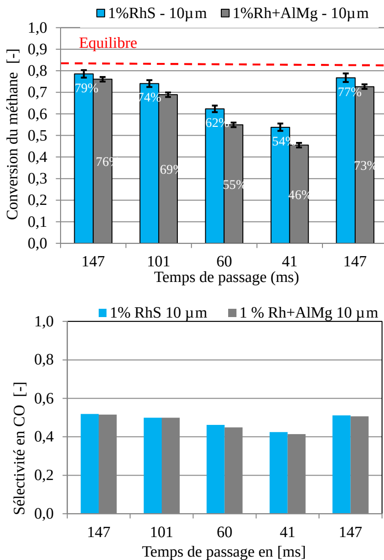
Figure 4.10: Impact du support sur la conversion et la sélectivité pour différents temps de contact et des dépôts de catalyseurs (support commercial et support par voie sol-gel) de 10 μm et contenant 1 % de rhodium.
