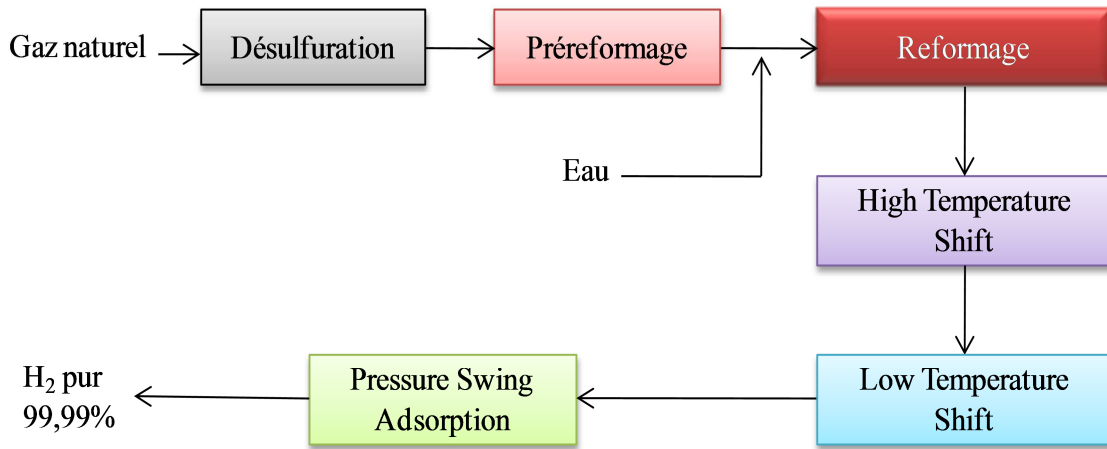
Figure 1.1 : Production d'hydrogène par vaporeformage.
