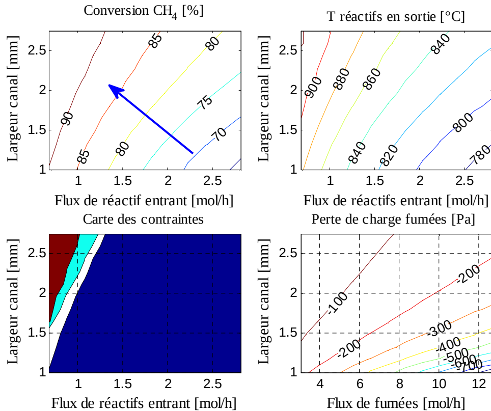
Figure 5.17 : Influence de la largeur des canaux et du débit total sur différentes caractéristiques du procédé en considérant la cinétique de la réaction SMR.
