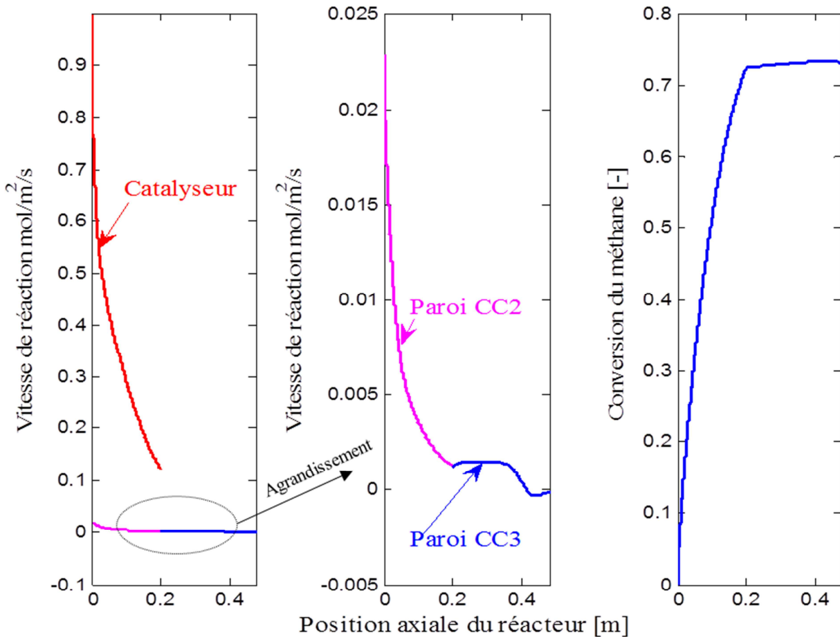
Figure 4.25: Evolution des vitesses de réaction le long du réacteur sur les différentes zones réactives (850°C, 20 bar et 60 ms). Le profil de température présenté sur la Figure 4.17 est utilisé comme condition limite.
