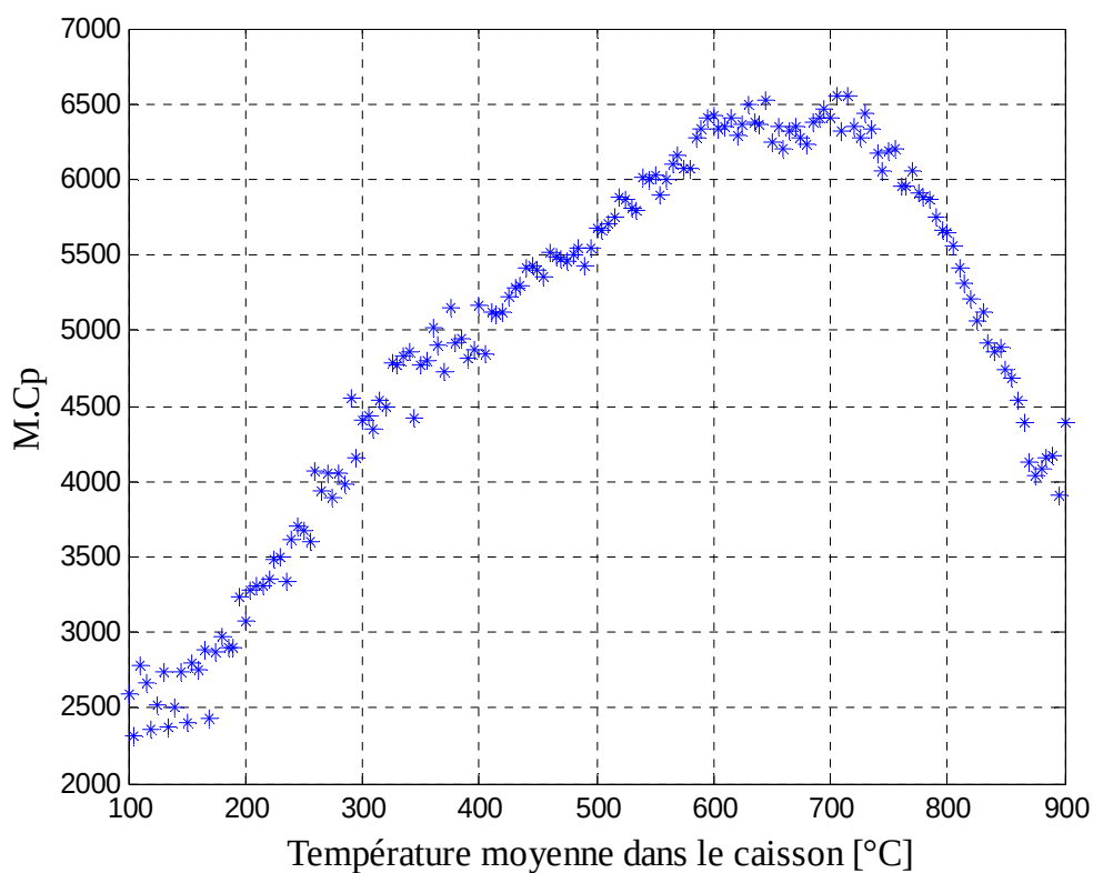
Figure 2.25 : Capacité calorifique de l'ensemble du caisson en fonction de la température moyenne dans le caisson.
