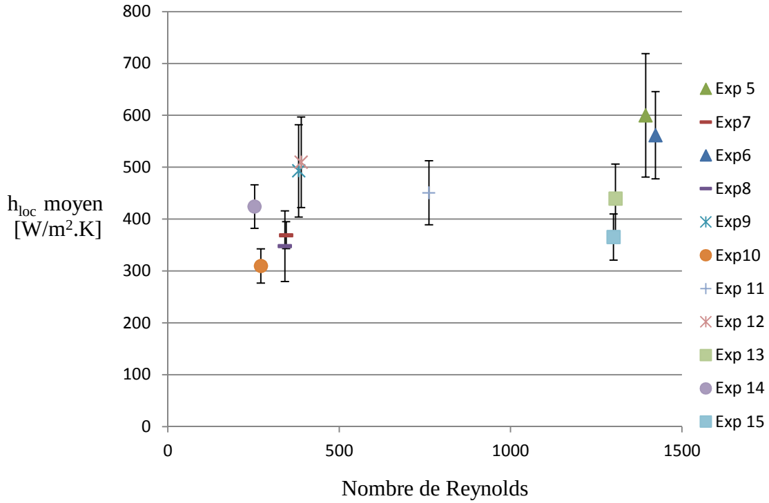
Figure 2.9: Variation de h_{loc} en fonction du nombre de Reynolds.
