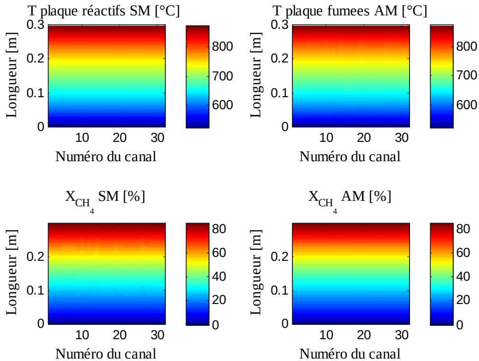
Figure 6.13 : Influence de la maldistribution de catalyseur sur la température des plaques et la conversion. SM : sans maldistribution, AM : avec maldistribution, T : température, X_{\text{CH}_4} : conversion.
