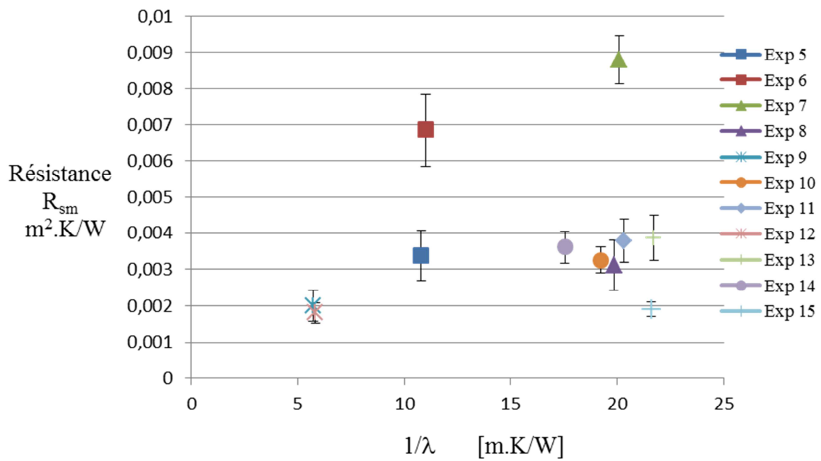
Figure 2.10 : Résistance expérimentale R_{sm} en fonction de 1/\lambda .
