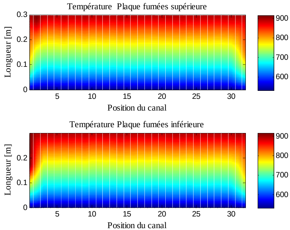
Figure 6.30 : Cartes de température pour une maldistribution des diamètres hydrauliques de 0,2 %.
