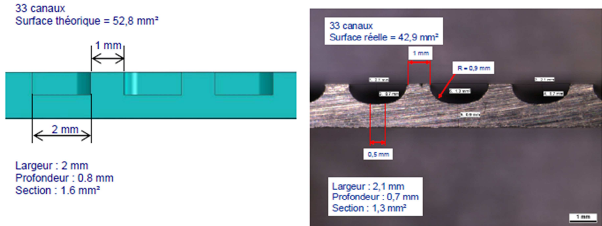
Figure 5.29 : Comparaison entre la forme théorique des canaux et celle usinée Chimiquement (largeur 2 mm).
