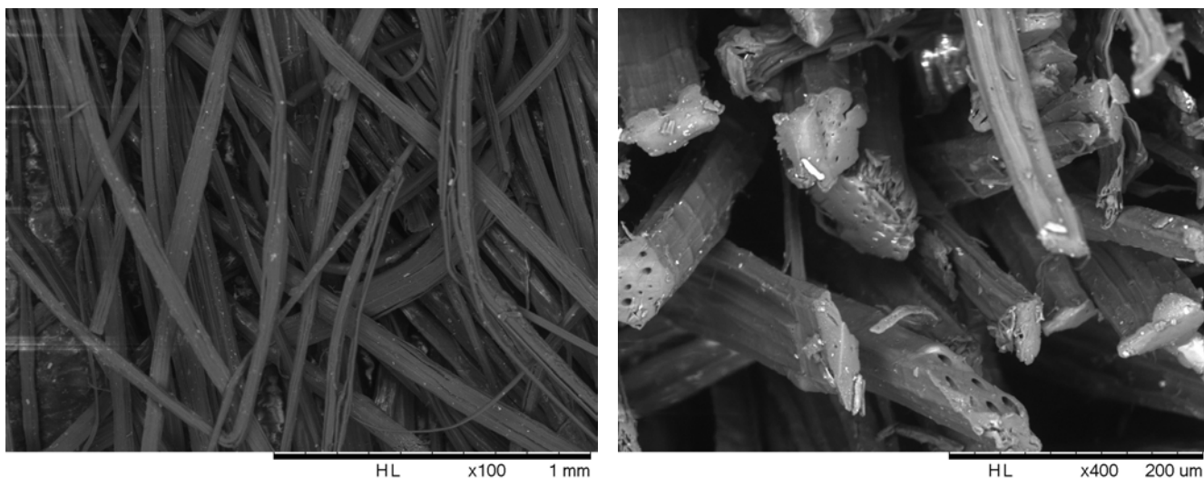
Figure 29 KENAF B en vue longitudinale et en coupe après cardage
