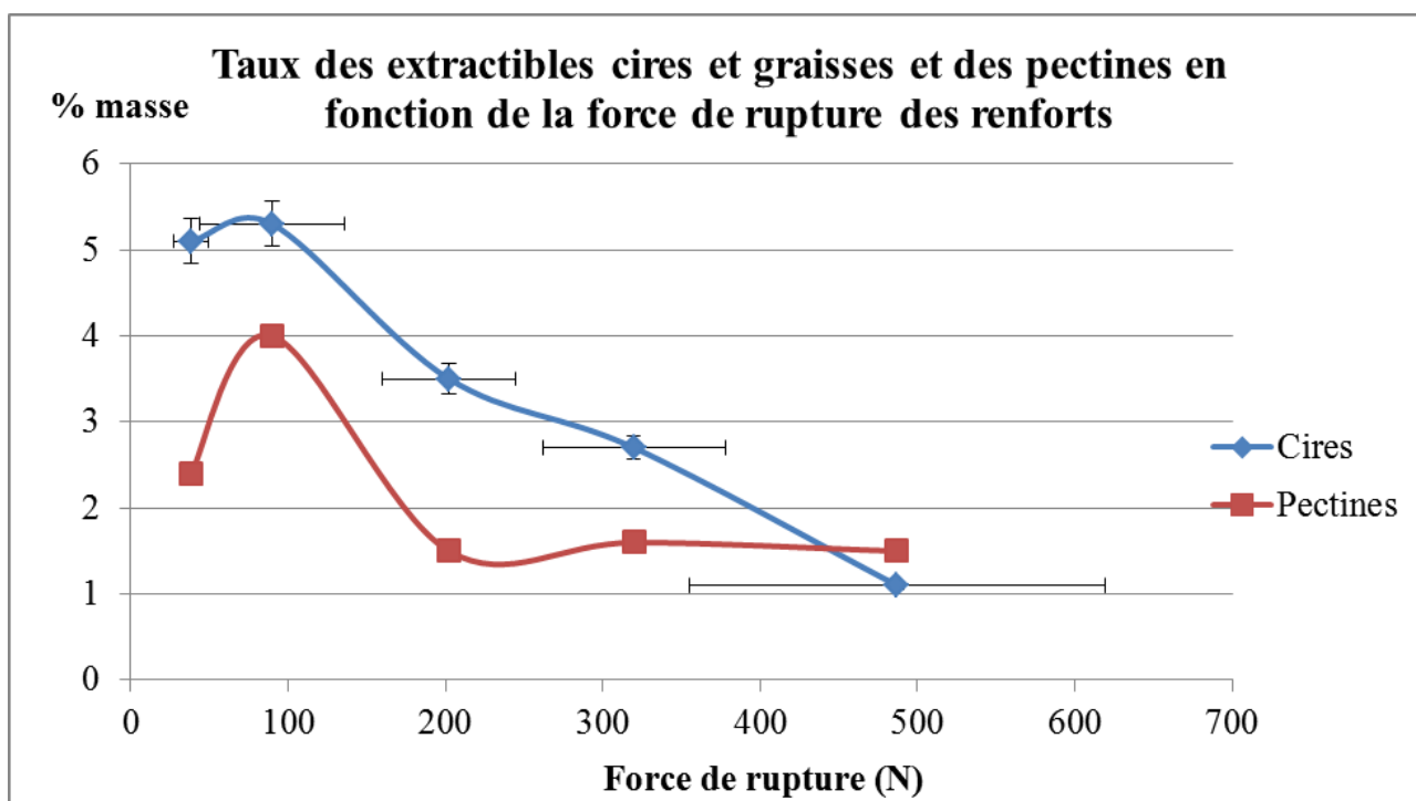
Figure 42 Taux des extractibles cires et graisses et des pectines en fonction de la force de rupture des renforts
