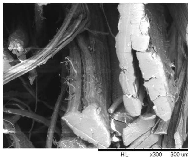
Figure 6 : CHAN1 en vue longitudinale et en coupe après cardage
