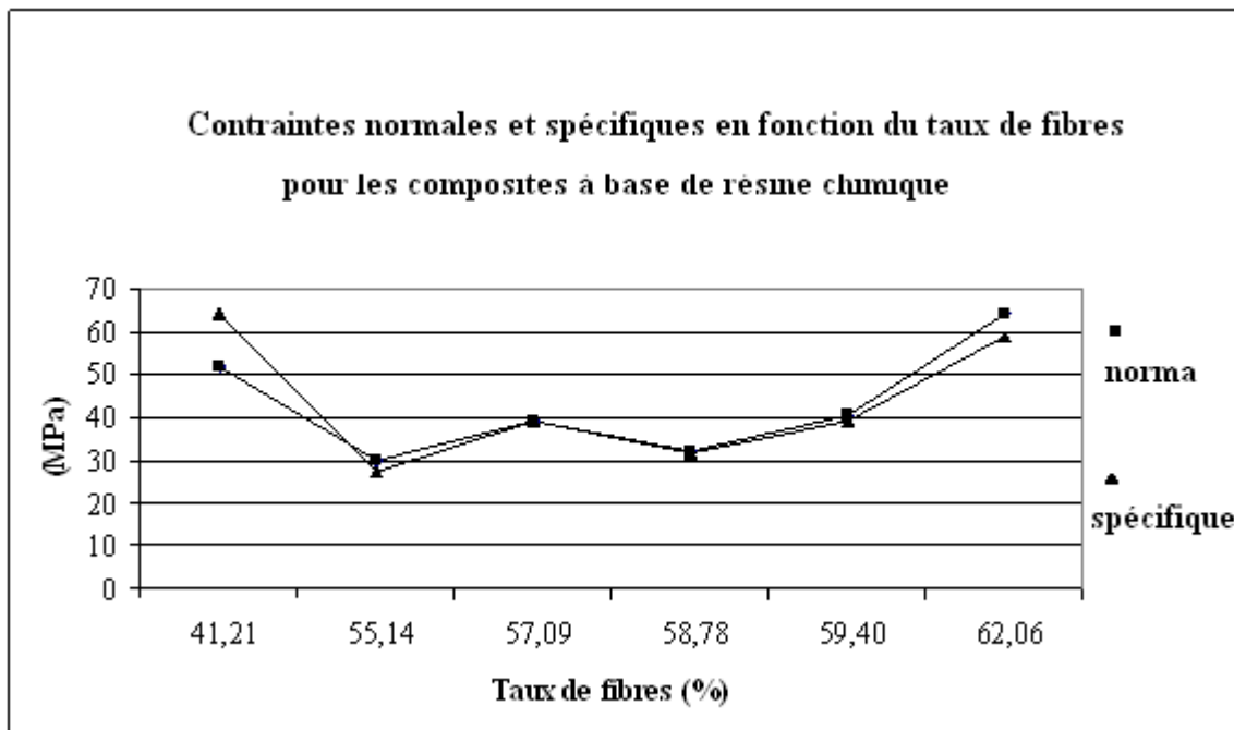
Figure 53 Contrainte en fonction du taux de fibres pour les composites à résine synthétiques
