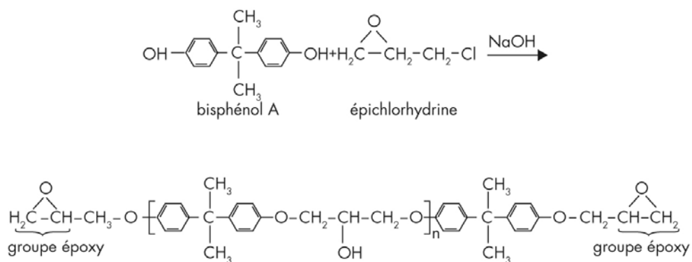
Figure 10 Réaction entre le bisphénol A et l'épichlorhydrine : obtention du diglycidyléther (DGEBA)
