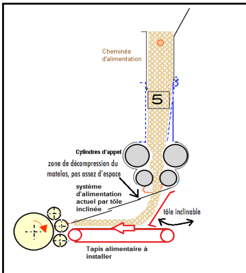
Figure 19 Schéma de la cheminée d'alimentation de la carde
