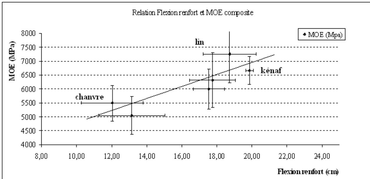
Figure 52 Relation entre flexion du renfort et MOE du composite
