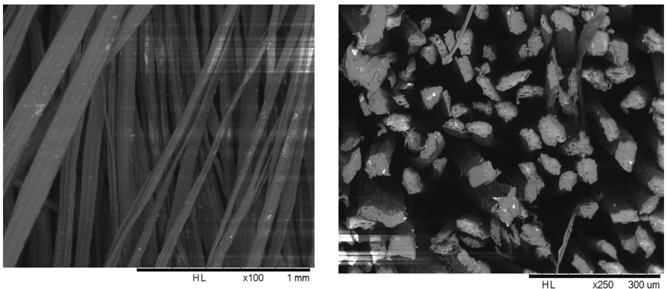
Figure 28 KENAF B en vue longitudinale et en coupe avant cardage Fibres après cardage
