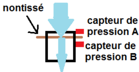
Figure 8 Vue en coupe du perméabilimètre à air
