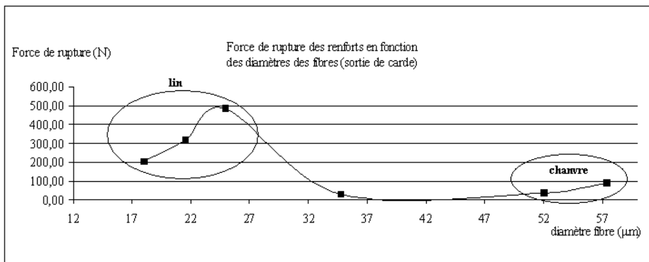
Figure 47 Force de rupture des renforts en fonction des diamètres des fibres (sortie de carde)
