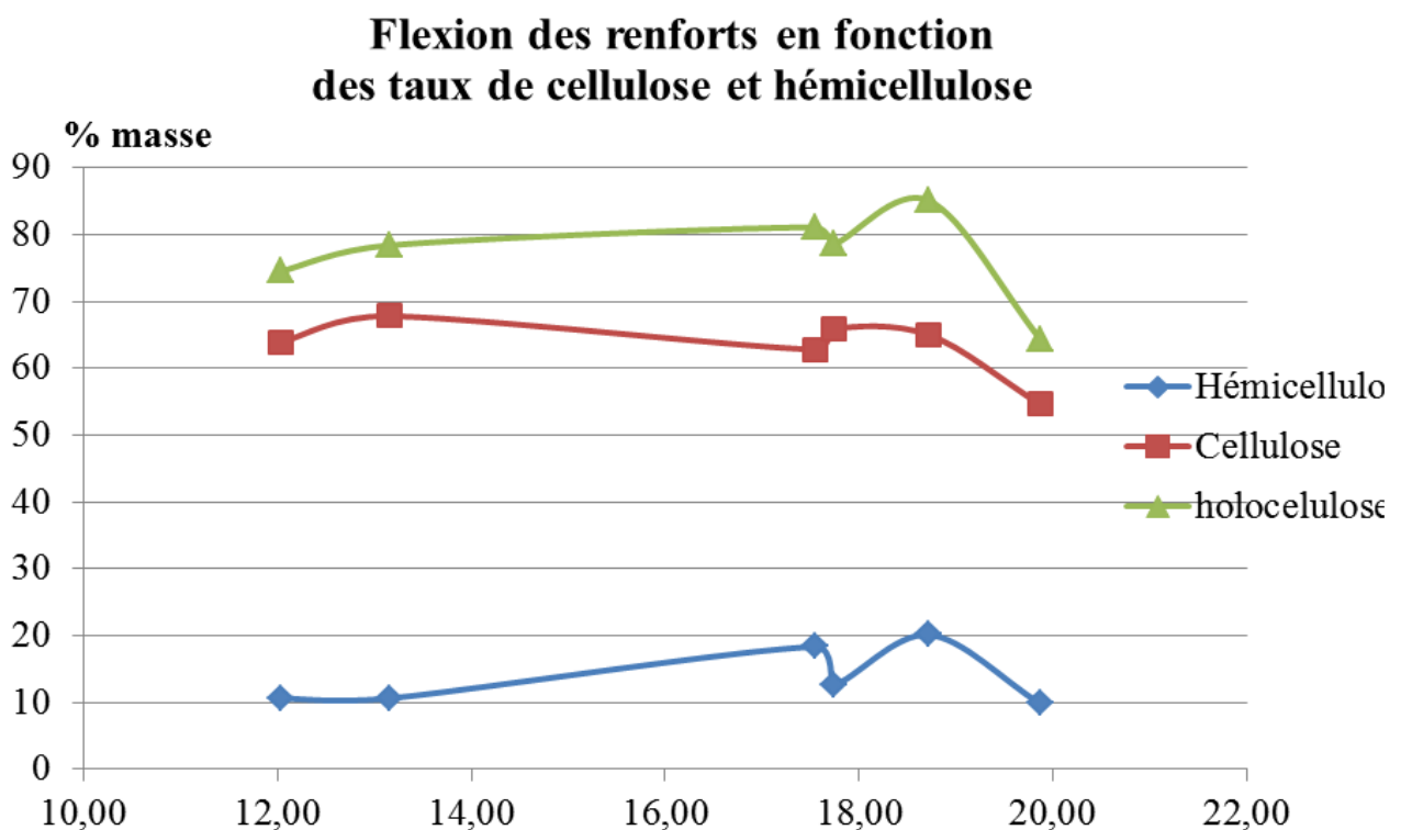
Figure 44 Flexion des renforts en fonction des taux de cellulose et hémicelluloses
