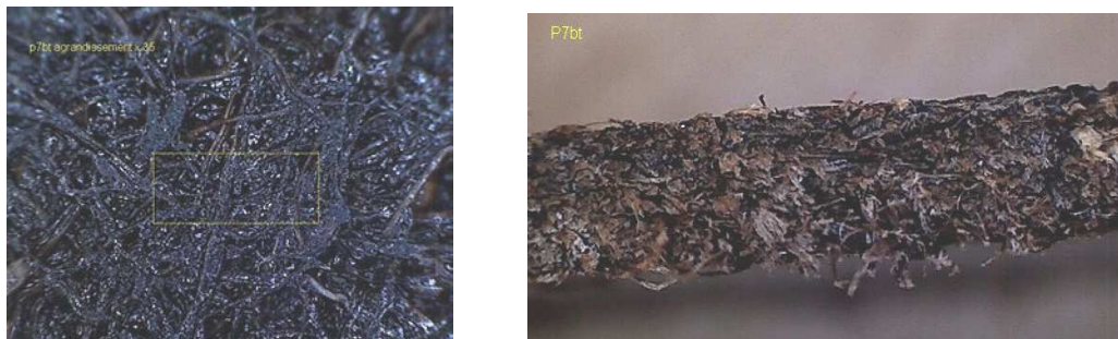
Figure 45 P7bt vue de face (x200) et en coupe (x35)
