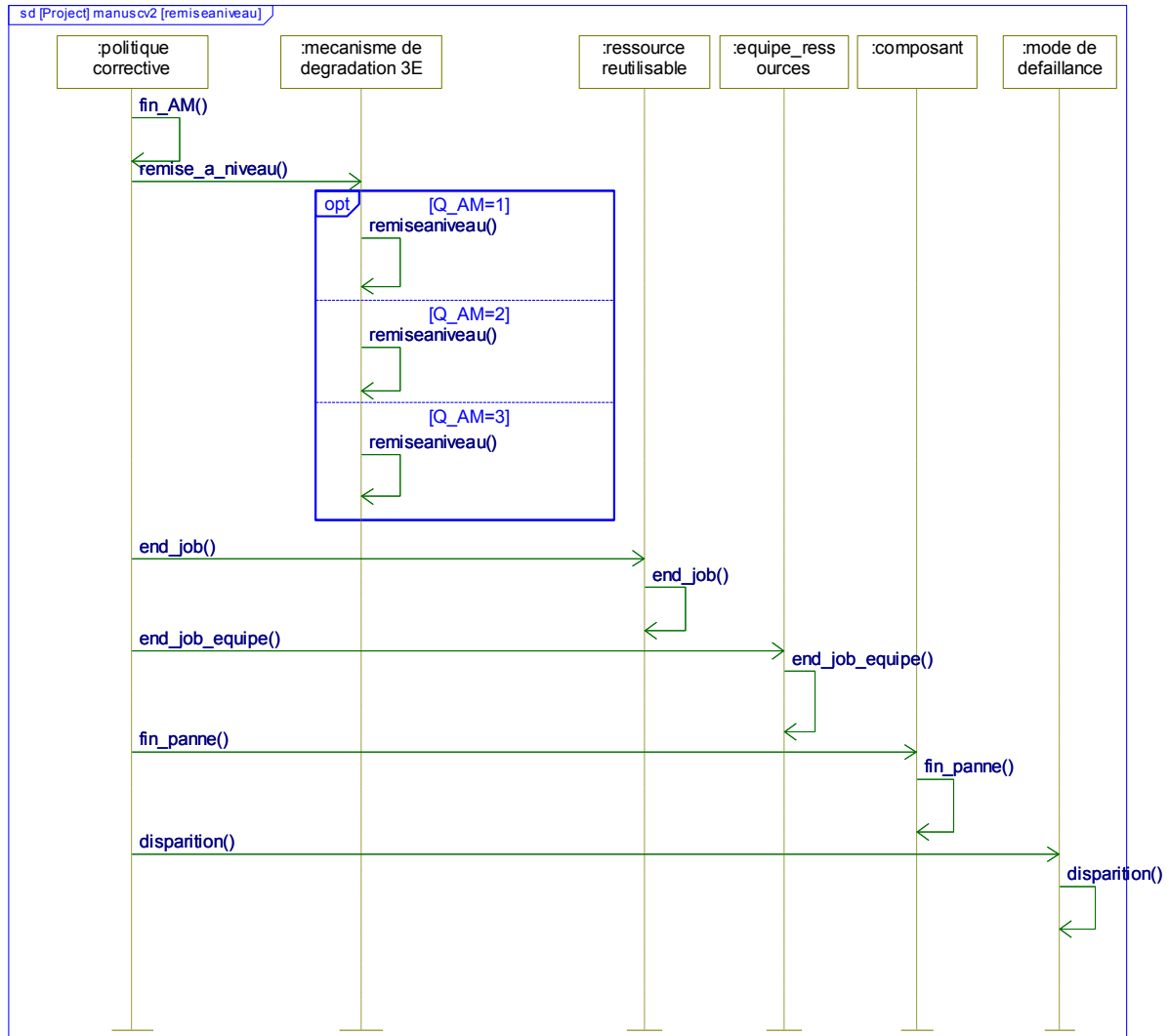
Figure 32 – SD relatif à la fin d’une politique corrective
