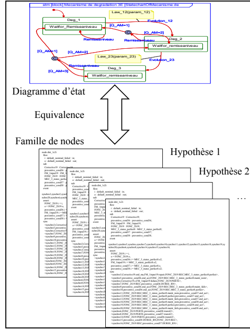
Figure 45 – Correspondances entre un diagramme d'état et une famille de nodes
