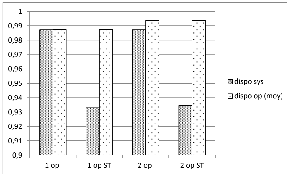
Figure 73 – Disponibilité du système et des opérateurs
