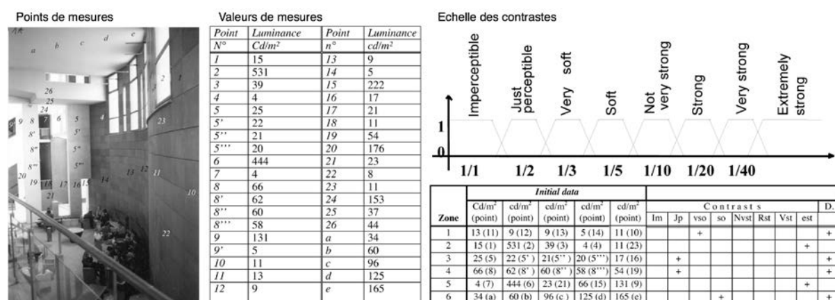
Fig 56. Caractérisation quantitative et qualitative de la lumière naturelle (Mudri, Lenard, 1999)
