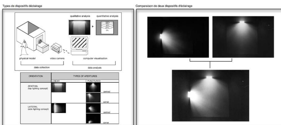
Fig 69. Méthode de création et de combinaison d'effets de lumière naturelle à partir d'images de référence (Demers, 2000)
