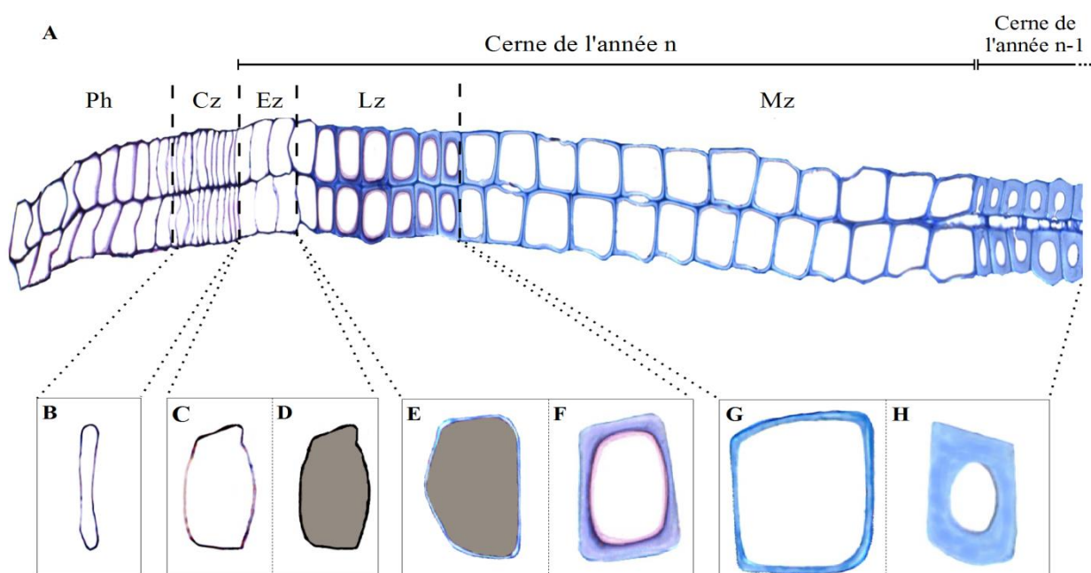
Figure III.6 : Maturation du xylème observée chez le pin sylvestre. La figure III.6A montre deux files radiales isolées d'une section anatomique de bois (6 \mu\text{m} d'épaisseur, coloration à l'actétate de violet de crésyl) coupée transversalement à partir d'un échantillon prélevé le 14 août 2009. Elles contiennent le phloème (Ph), les zones cambiale (Cz), d'élargissement (Ez), d'épaississement et lignification (Lz) et mature (Mz) de différenciation des trachéides. Les figures III.6B à III.6H illustrent des cellules isolées de chaque zone de différenciation avec une cellule cambiale (B), une cellule en élargissement en lumière normale (C) et polarisée (D), une cellule en épaississement en lumière polarisée (E) et normale (F), une cellule mature du bois initial du cerne de l'année en cours (G) et une cellule mature du bois final du cerne de l'année précédente (H).
