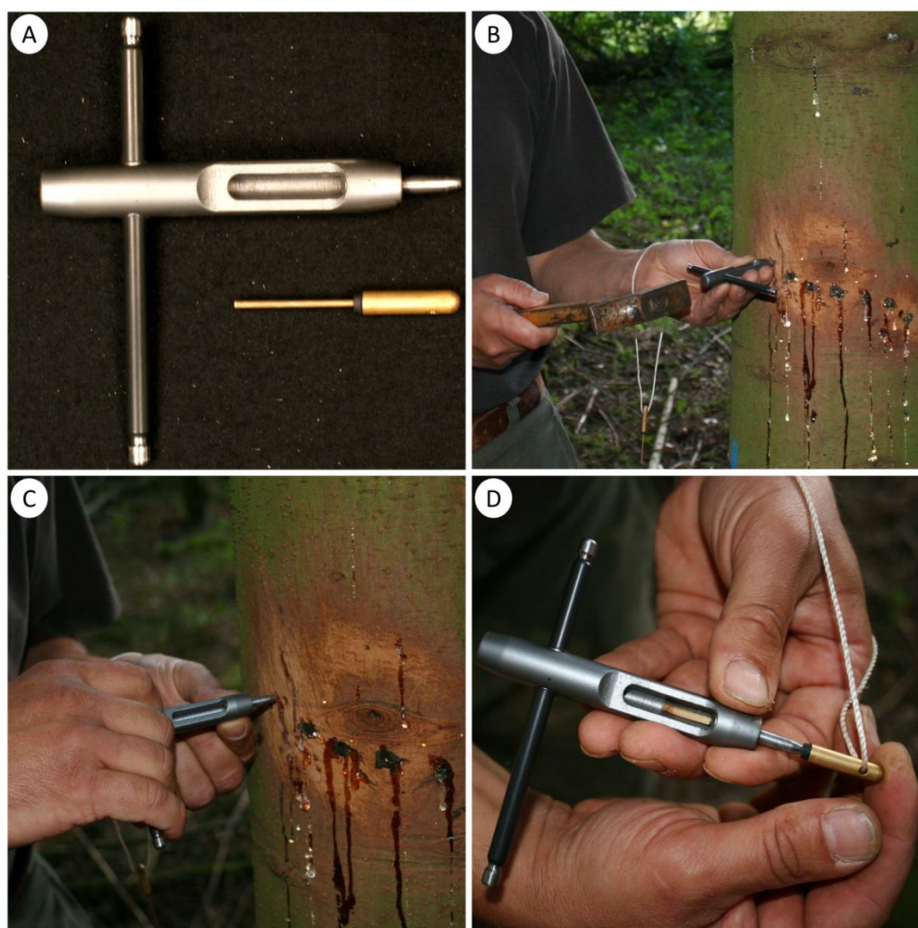
Figure III.4 : Prélèvement des microcarottes avec un Trephor. A. Le Trephor accompagné de sa baguette de laiton utilisée comme extracteur. B. Insertion du Trephor dans le tronc à l'aide d'un marteau. C. Retrait du Trephor en tournant l'appareil comme un tire-bouchon. D. Récupération de la microcarotte dans la chambre d'extraction à l'aide de l'extracteur.
