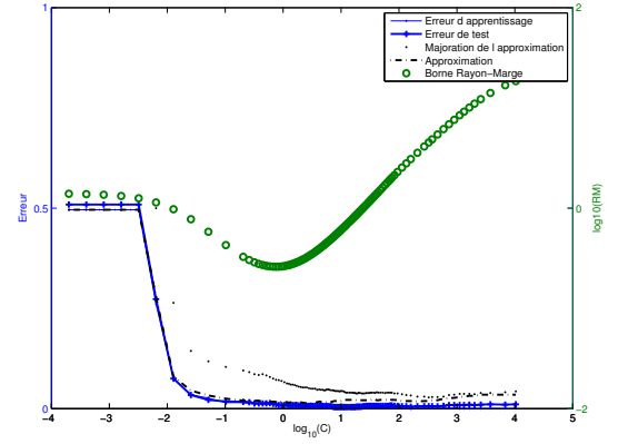
(d) : Toy (gaussien)
