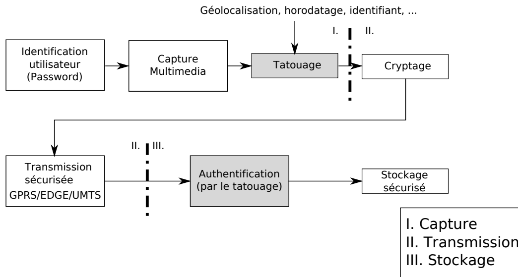
Figure 1.1 – La chaîne de certification de CodaSystem, de la prise de photo au stockage sécurisé
