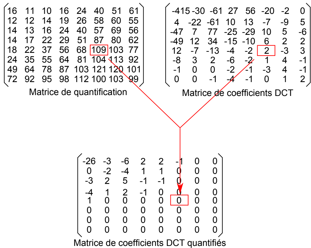
Figure 2.3 – Quantification des coefficients DCT par la matrice de quantification, où par exemple, 2 / 109 = 0
