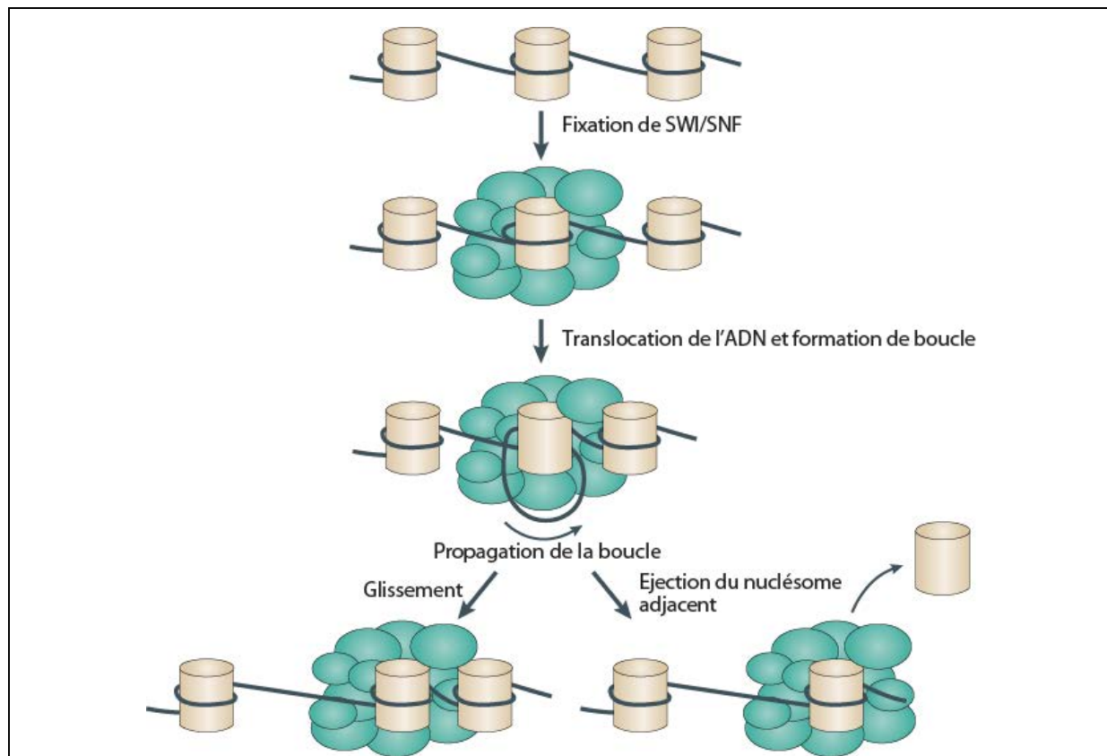
Figure 11 : Modèle d'action de SWI/SNF
