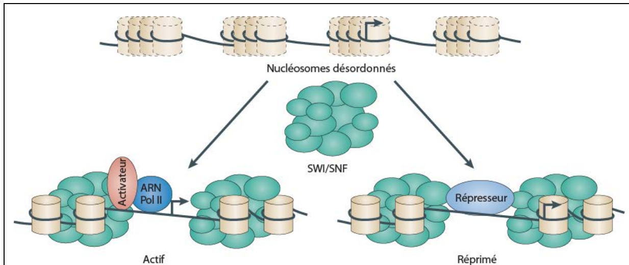
Figure 12 : Effet de l'action de SWI/SNF sur l'accès des facteurs de fixation à l'ADN
