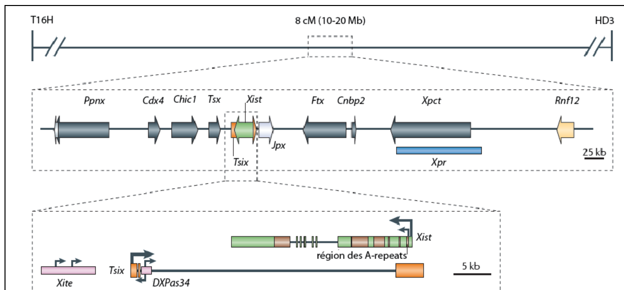
Figure 25 : Le centre d'inactivation du chromosome X (XIC) murin
