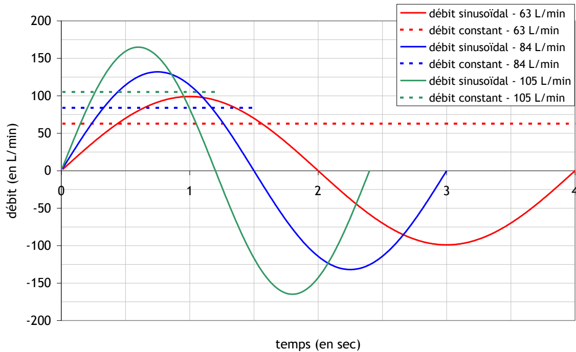
Figure D-1. Débits sinusoïdaux et débits constants correspondants pour les trois respirations
