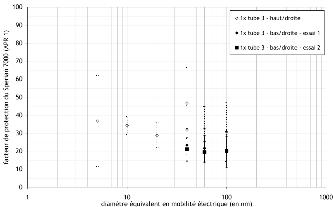
Figure 5-4. Facteurs de protection expérimentaux en présence d'une fuite de 2,8 mm et en débit constant de 84 L/min
