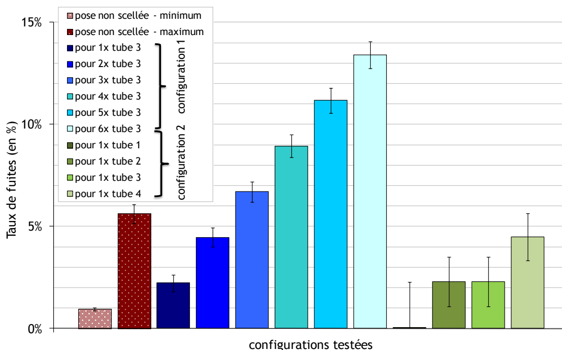
Figure 5-18. Comparaison des taux de fuites en présence de tubes calibrés et en pose non scellée
