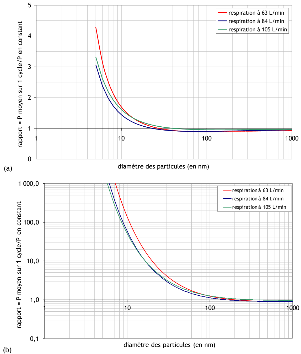
Figure D-4. Rapport de la perméance moyenne au cours d'un cycle sur la perméance en aspiration constante en fonction de la taille des particules dans le cas des trois respirations et pour le medium 4 (a) et le medium 7 (b)
