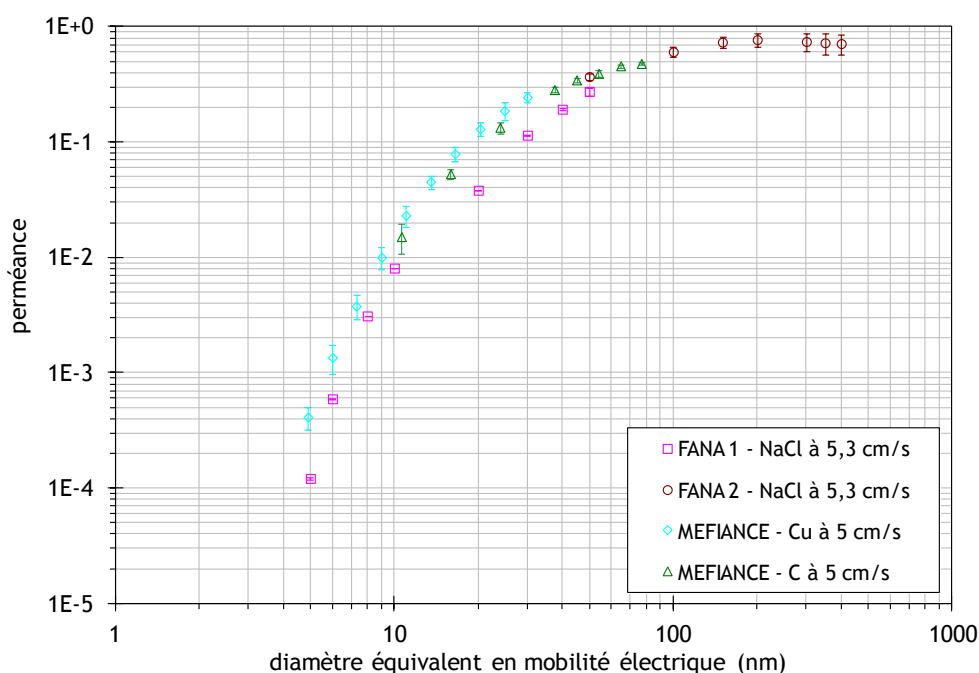
Figure 2-11. Perméance spectrale du medium 1 pour des nanoparticules de nature diverses
