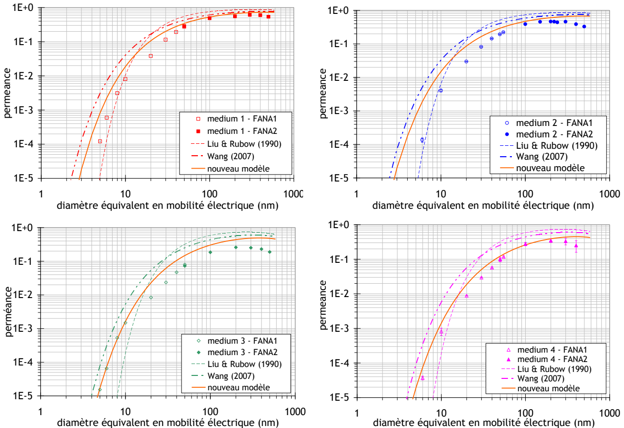
Figure 2-17. Comparaison des modèles avec les perméances spectrales des media 1 à 4
