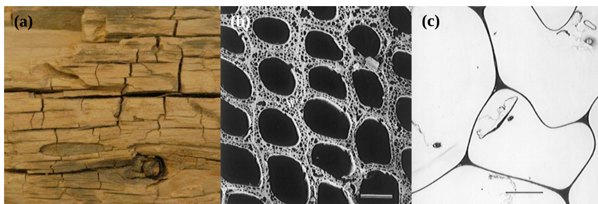
Figure 21 : Attaque du bois par la pourriture molle à différentes échelles. (a) Caractéristique macroscopique de l'attaque. (b) Caractéristique microscopique de l'attaque de type 1 : apparition des cavités au sein de la paroi secondaire. (c) Caractéristique microscopique de l'attaque de type 2 : érosion complète de la paroi secondaire laissant intacte la lamelle moyenne (Blanchette, 2000).
