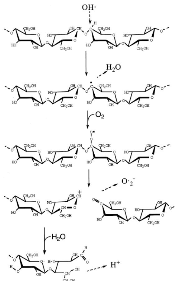
Figure 28 : Mécanisme de scission des polysaccharides par les radicaux hydroxyles générés lors de la réaction de Fenton (ici exemple de la cellulose) (Henriksson et al., 2000). Un atome d'hydrogène est extrait du carbone 4 par le radical hydroxyle créant un radical sur ce dernier. Celui-ci est oxydé avec formation d'un anion superoxyde suivi du clivage de la liaison glycosidique. Un carbonyle et un carbanion sont formés sur les nouvelles extrémités. Ce dernier sera déprotonné avec ouverture du cycle grâce à une molécule d'eau.
