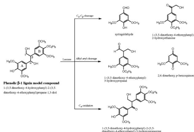
Figure 51 : Oxydation des modèles de dimères phénolique \beta -1 de la lignine catalysée par les laccases (Kawai et al., 1988).
