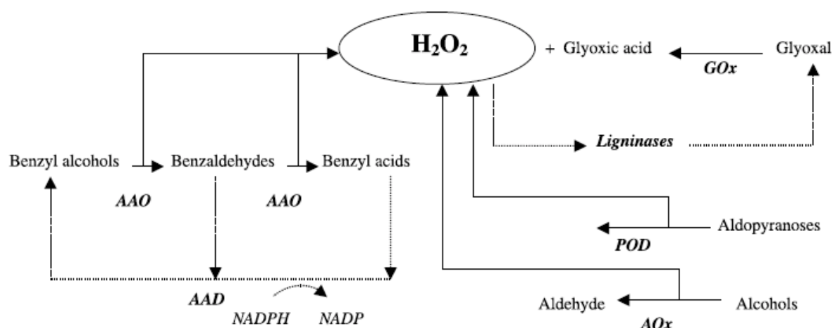
Figure 54 : Représentation schématique des différentes voies de biosynthèse de l' \text{H}_2\text{O}_2 (Shah et Nerud, 2002). GOx, glyoxal oxydase ; POD, pyranose oxydase ; AOx, alcool oxydase ; AAD, aryl alcool déshydrogénase ; AAO, aryl alcool oxydase.
