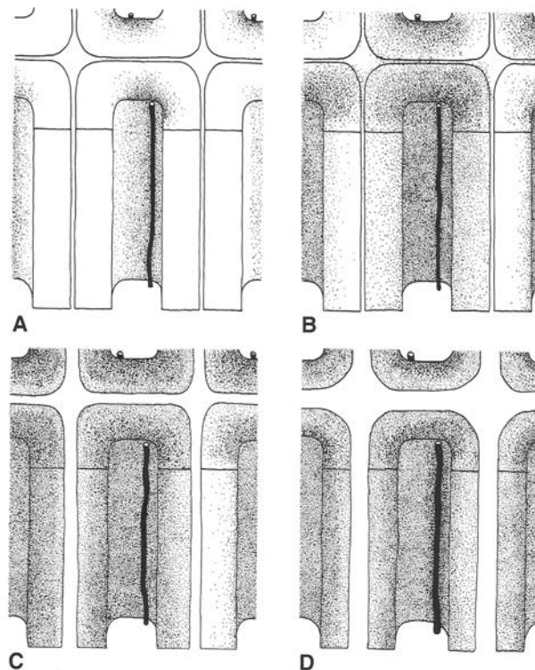
Figure 25 : Stades de progression de la pourriture sélective. (A),(B) Au stade précoce les enzymes (représentées par des points) diffusent dans la paroi secondaire depuis l'hyphe en croissance dans la lumière causant la dégradation de la lignine qui s'étend jusqu'à la lamelle moyenne. (C),(D) Au stade tardif la dégradation préférentielle de la lignine conduit à la séparation des cellules (Schwarze et al., 2000).
