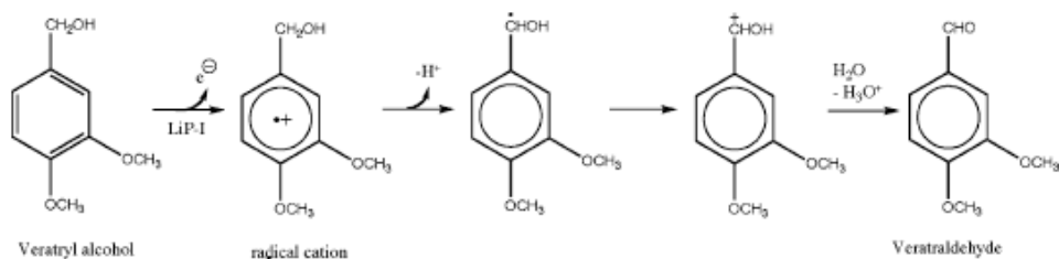
Figure 41 : Déclin du radical cationique de l'alcool vératryl par déprotonation du C \alpha (Baciocchi et al., 2002).
