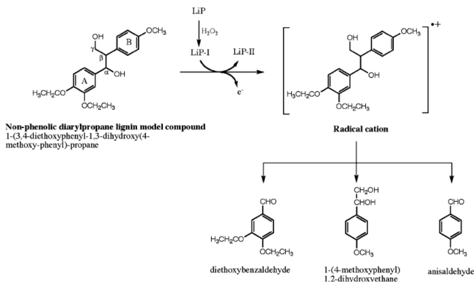
Figure 39 : Oxydation des composés modèles de dimères non phénolique diarylpropanes de la lignine catalysée par les LiP. L'oxydation du noyau A donnant lieu au clivage de la liaison C \alpha -C \beta représente la voie majeure (Lundell et al., 1993; Renganathan et al., 1985).
