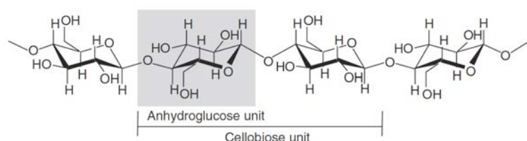
Figure 6 : Structure chimique de la cellulose montrant la répétition des molécules de \beta -D-glucose (entouré en gris) ainsi que l'unité de cellobiose (Pereira et al., 2003).
