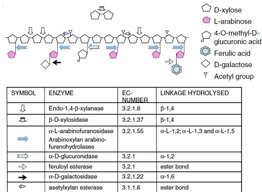
Figure 34 : Exemple de synergie dans la dégradation des arabinoxylanes (Aro et al., 2005).
