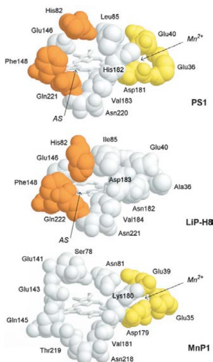
Figure 47 : Comparaison structurale de la LiP de P.chrysosporium (LiP-H8), de la MnP de P.chrysosporium (MnP1) et de la VP de Pleurotus eryngii (PS1). Les résidus impliqués dans la fixation du Mn^{2+} sont colorés en jaune et les résidus impliqués dans la reconnaissance de l'alcool vératryl et des substrats aromatiques (AS) sont colorés en orange (Camarero et al., 1999).
