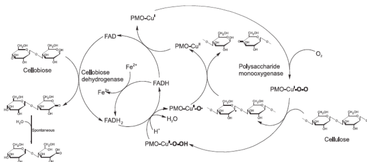
Figure 33 : Schéma représentant les réactions catalysées par les PMO et leur coopération avec les CDH (Žifčáková et Baldrian, 2012).
