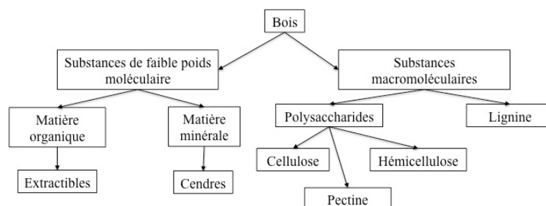
Figure 5 : Schéma général des constituants chimiques du bois (d'après Pereira et al., 2003).
