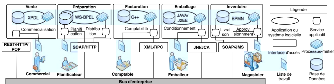
Figure 1.3 – Architecture applicative : une vue de l'infrastructure logicielle du détaillant.
