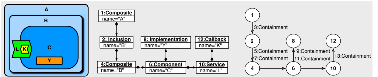
Figure 5.9 – Exemple d'un modèle SCA assimilable à un graphe.
