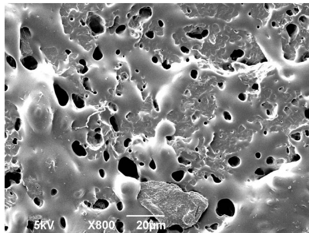
Figure 15 MEB image du mélange PBA/PLA (20/80) quand le tensioactif composite -[0.5gBrij700 avec 2g PEGMEM] a été utilisée dans la préparation de latex PBA. dn=1.57 \mu\text{m} , dv=5.05 \mu\text{m} .
