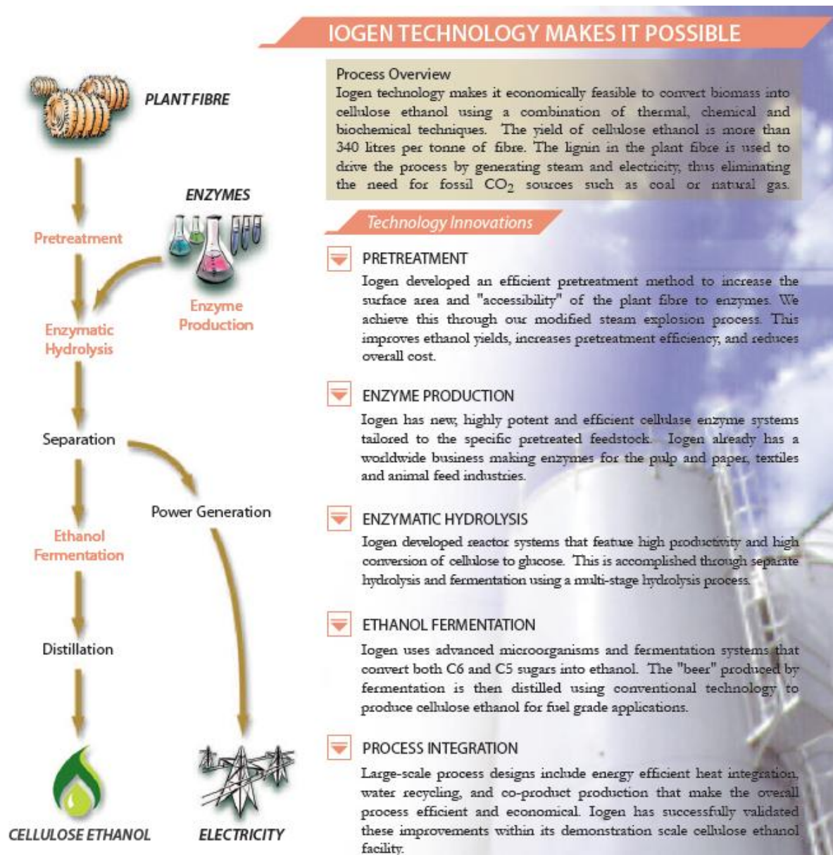
Figure11 : L'utilisation d'enzymes afin de dégrader la ligno-cellulose permet d'augmenter la production d'éthanol (Source IOGEN : www.iogen.ca ).
