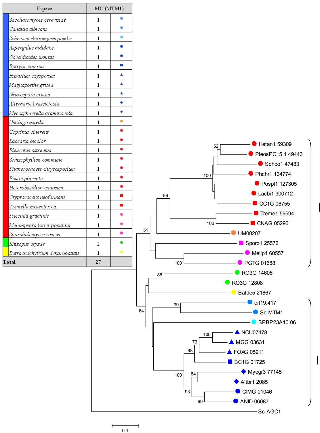
Figure 87 : Arbre phylogénétique présentant les orthologues de MTM1 de S. cerevisiae . Le tableau présent dans la figure reprend le nombre de transporteurs présent pour chaque organisme. Les séquences ont été alignées avec le logiciel MEGA afin de générer un arbre selon la méthode du neighbour-joining. Les bootstraps ont été calculés à l'aide de 1000 répétitions. AGC1, un transporteur de la superfamille des MC a été utilisé comme outgroup.
