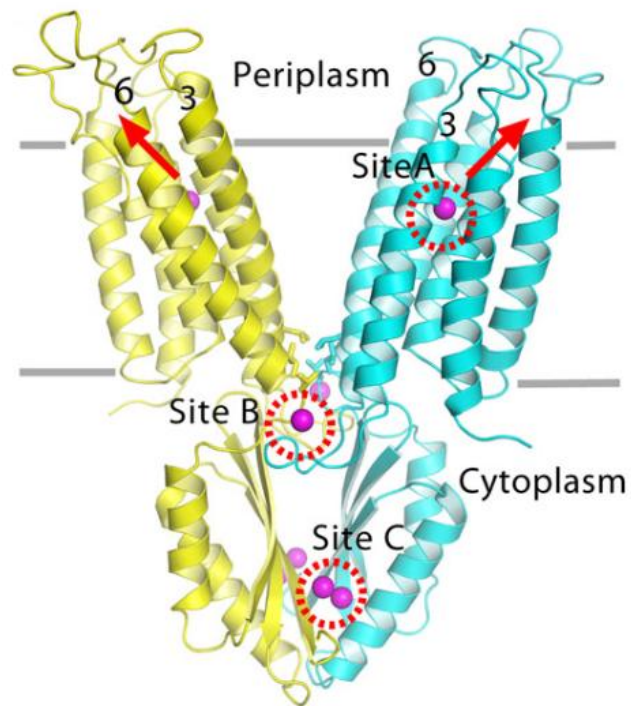
Figure 125 : Structure de YjiP : Représentation de l'homodimère (un protomère en jaune et un en cyan). Les sphères en magenta représentent les ions de zinc associés aux sites marqués par des cercles rouges. Les lignes grises indiquent les limites de la membrane et les flèches rouges indiquent les directions de sortie du Zn des deux sites actifs (Lu et al, 2009).
