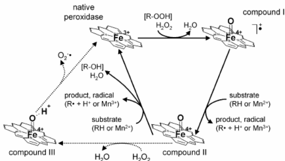
Figure 17 : Mécanisme catalytique des peroxydases impliquées dans la dégradation de la lignine (Cullen & Kersten, 2004).
