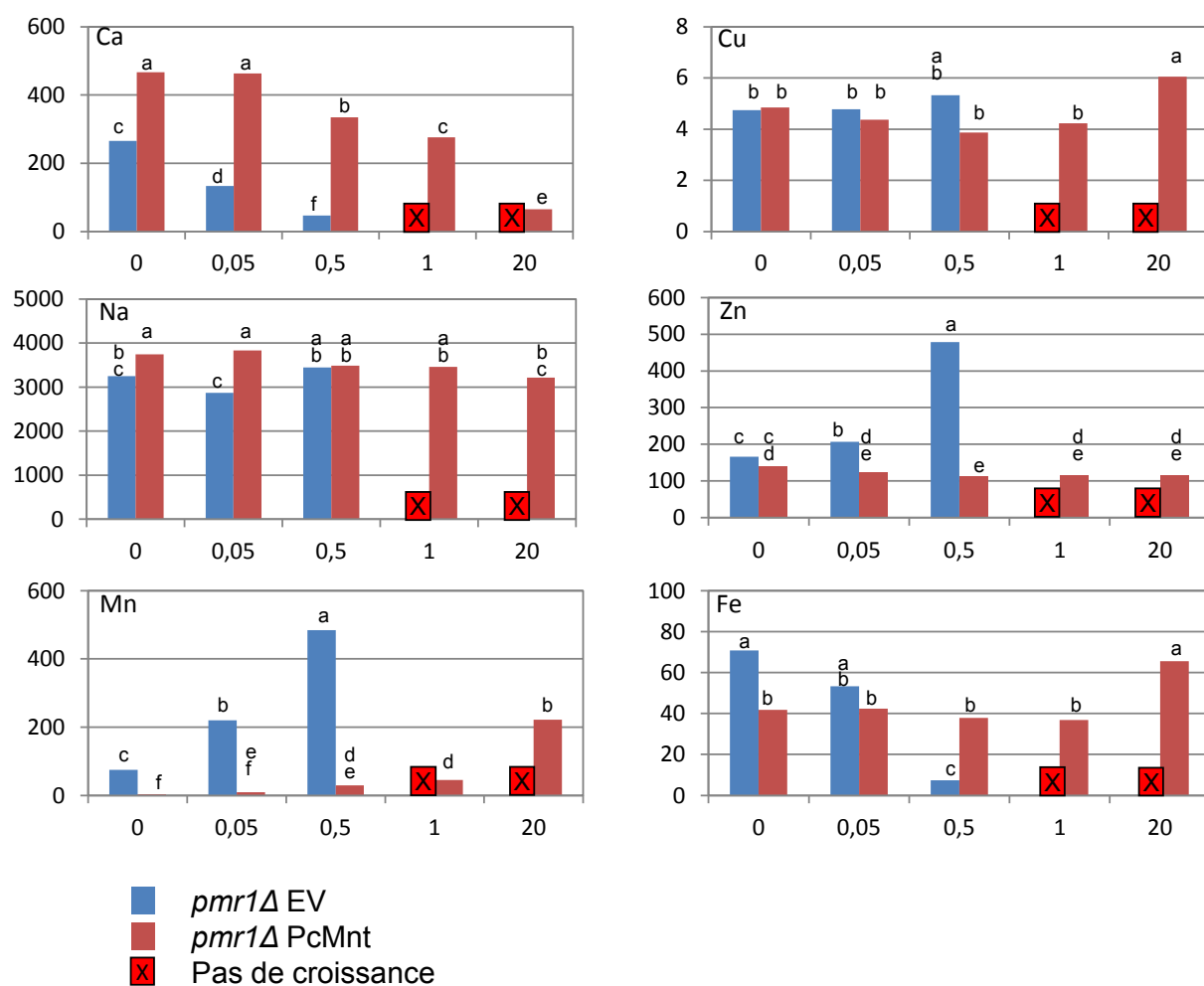
Figure 112 : Concentration intracellulaire de différents éléments (en \mu\text{g/g MS} ) pour la souche pmr1\Delta transformée avec le vecteur vide ou avec le vecteur contenant PcMnT en fonction de la concentration de \text{Mn}^{2+} (en mM) dans le milieu de culture. Une lettre différente indique une différence significative de valeur avec une P value \leq 0,05 .
