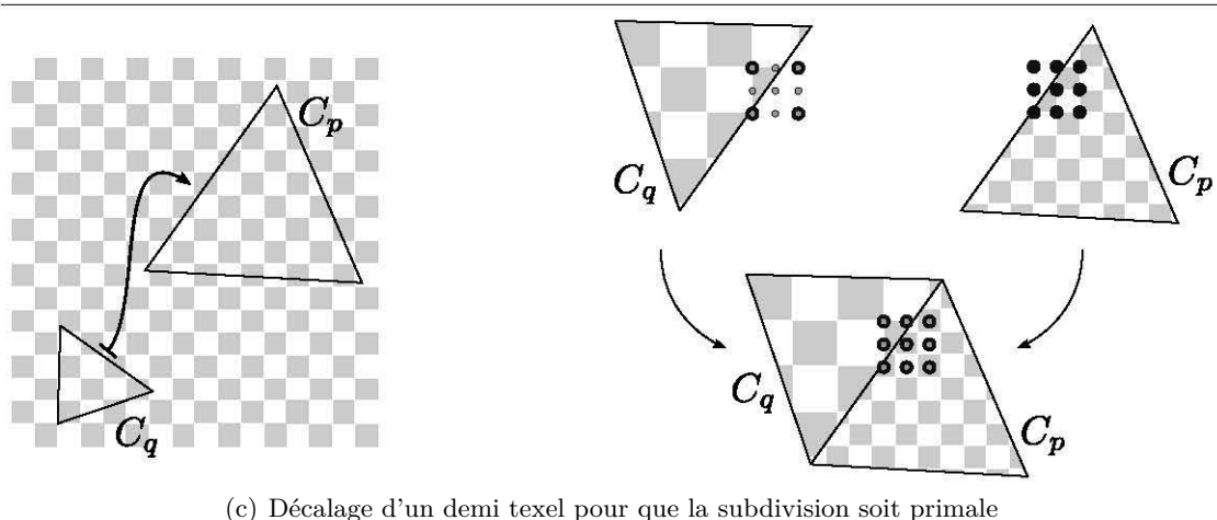
FIGURE 2.27 – Relation entre subdivision du mipmapping et subdivision du mode de filtrage. L'atlas initial (a) est généré pour assurer un placage sans couture apparente au niveau de mipmap le plus grossier supporté. Ici, deux triangles C_p et C_q adjacents sont de résolution différentes, et en subdivisant les texels de C_q , nous pouvons les aligner avec ceux de C_p en collant bord à bord les triangles. Au niveau de mipmap de résolution immédiatement supérieur (b), les texels sont subdivisés de manière duale et les texels des triangles C_p et C_q ne peuvent plus être alignés. En décalant les coordonnées paramétriques d'un demi texel (c), il est de nouveau possible d'aligner les texels de C_p et C_q .
