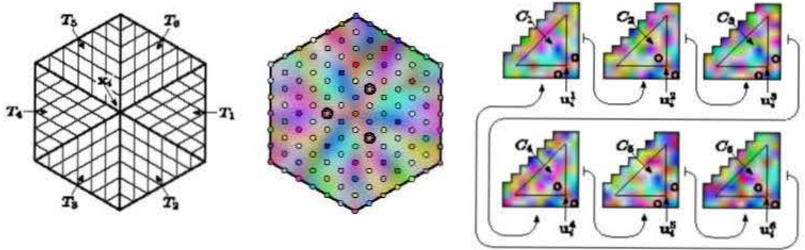
FIGURE 2.14 – Classes d'équivalence au voisinage d'une singularité d'indice -\frac{1}{2} , dans le cadre du filtrage bicubique. À gauche, les cellules de filtres de six triangles \{T_k\}_{k=1}^6 s'agencent pour former une singularité d'indice -\frac{1}{2} au sommet \mathbf{x}_i . Au centre une texture aléatoire est plaquée sans couture visible, avec un filtrage bicubique. Les points de la surface dont les coordonnées correspondent aux positions de texels sont marqués avec la couleur des texels correspondants. Nous voyons apparaître des points de la surface distincts correspondant à des texels contraints à avoir la même valeur. À droite, les versions paramétriques \{C_k\}_{k=1}^6 des triangles, avec les texels utiles de chaque carte. Les flèches indiquent comment les cartes se recollent. La classe correspondant aux trois positions marquées sur la surface au centre contient deux texels par carte, centrés sur les coordonnées paramétriques \mathbf{u}_i^k de la singularité. Sur trois des cartes, l'un de ces texels est à l'intérieur du triangle paramétrique, ces trois texels correspondent à ceux marqués sur la surface au centre.
