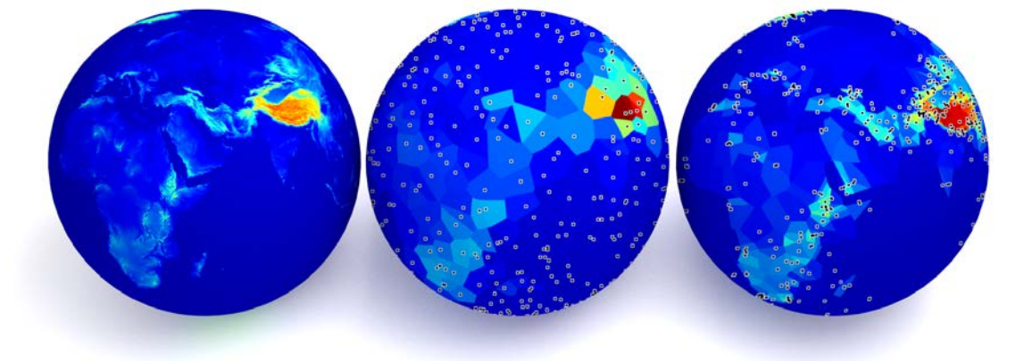
FIGURE 3 – Approximation de la fonction « altitude » sur la surface de la terre. À gauche, la fonction originale, au centre une approximation utilisant un échantillonnage de 1000 points tirés uniformément au hasard, à droite un échantillonnage de 1000 points optimisés.
