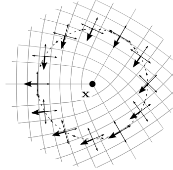
FIGURE 1.14 – Un exemple de champ de directions continu de symétrie 4 à partir duquel il n’est pas possible de produire un champ de vecteurs continu. En suivant une boucle autour du point central \mathbf{x} comme pour la Figure 1.13, le champ de directions effectue une rotation d’angle \frac{\pi}{2} . Le point \mathbf{x} est donc une singularité d’indice \frac{1}{4}
