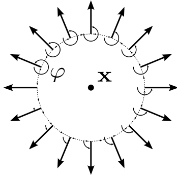
FIGURE 1.13 – Le champ de vecteurs défini dans le plan par \mathbf{w}(x, y) = (x, y)^t , a une singularité en \mathbf{x} = (0, 0) . Après avoir réalisé un tour le long d’une boucle autour de la singularité, le champ de vecteurs aura parcouru un angle \varphi = 2\pi par rapport à sa position initiale. L’indice de cette singularité vaudra donc 1.
