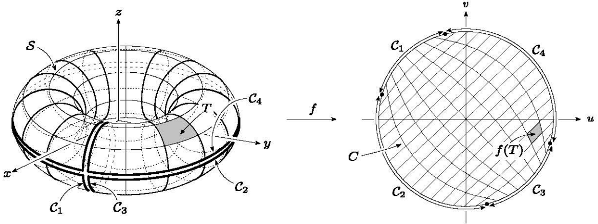
FIGURE 1.10 – Paramétrisation de Tutte pour le cas d’un tore. Sur le schéma, la surface \mathcal{S} a été découpée le long des transitions, pour former quatre courbes circulaires \mathcal{C}_1, \dots, \mathcal{C}_4 . Les sommets du bord de l’unique carte \mathcal{C} ont été placés sur un cercle pour assurer la convexité. Le résultat est bien une paramétrisation sans recouvrements. Cette méthode fonctionne avec des faces non triangulaires, et nous l’avons ici appliquée à un maillage quadrangulaire.
