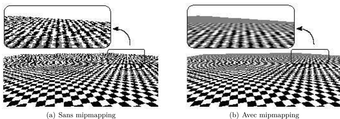
FIGURE 2.7 – Effet du mipmapping pour diminuer l'effet de crênelage lorsque la texture a une résolution plus forte que l'affichage.
