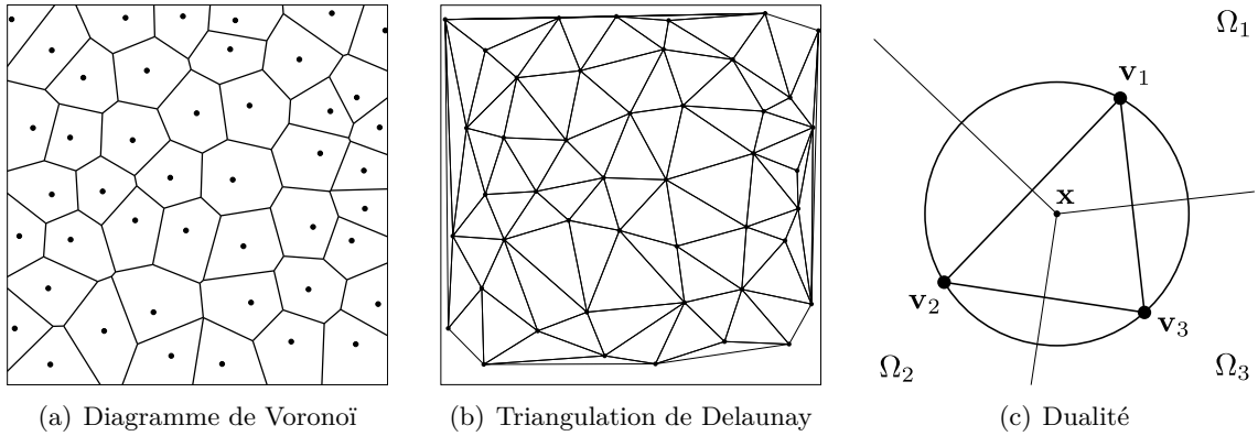
FIGURE 3.4 – Un diagramme de Voronoï et la triangulation de Delaunay associée. La triangulation de Delaunay est duale au diagramme de Voronoï : à la région \Omega_1 correspond le sommet v_1 , à l'arête entre \Omega_1 et \Omega_2 correspond le segment [v_1, v_2] , et au sommet x commun à \Omega_1, \Omega_2 et \Omega_3 correspond le triangle (v_1, v_2, v_3) .
