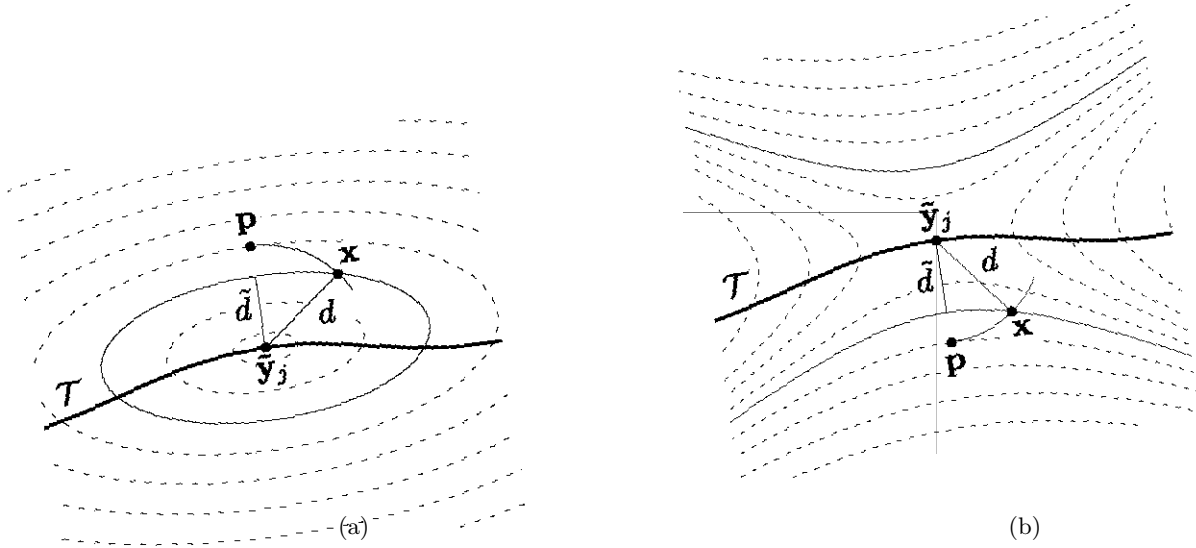
FIGURE 5.3 – En pointillés, les isovalues de l'approximation au second ordre de la distance au carré à \mathcal{T} en \tilde{\mathbf{y}}_j . Le développement limité au second ordre est pris au point \mathbf{p} , à la même distance d de \tilde{\mathbf{y}}_j que \tilde{\mathbf{x}}_i dans la direction de la normale en \tilde{\mathbf{y}}_j . C'est au point \mathbf{p} que l'approximation a un contact d'ordre 2 avec la distance au carré à \mathcal{T} . Deux cas sont possibles selon que \mathbf{x} se trouve du côté opposé au cercle osculateur en \tilde{\mathbf{y}}_j (a) ou du côté opposé (b). L'isovaleur correspondant au point \tilde{\mathbf{x}}_i est celle qui n'est pas en pointillés. \tilde{d} est la distance mise au carré pour approximer la distance entre \tilde{\mathbf{x}}_i et \mathcal{T} . Dans le cas (b) où \tilde{\mathbf{x}}_i est du même côté de \mathcal{T} que le cercle osculateur en \tilde{\mathbf{y}}_j , l'approximation de la distance au carré n'est plus une fonction positive. Pottmann et Hofer [86] proposent une modification de l'approximation pour corriger ce problème.
