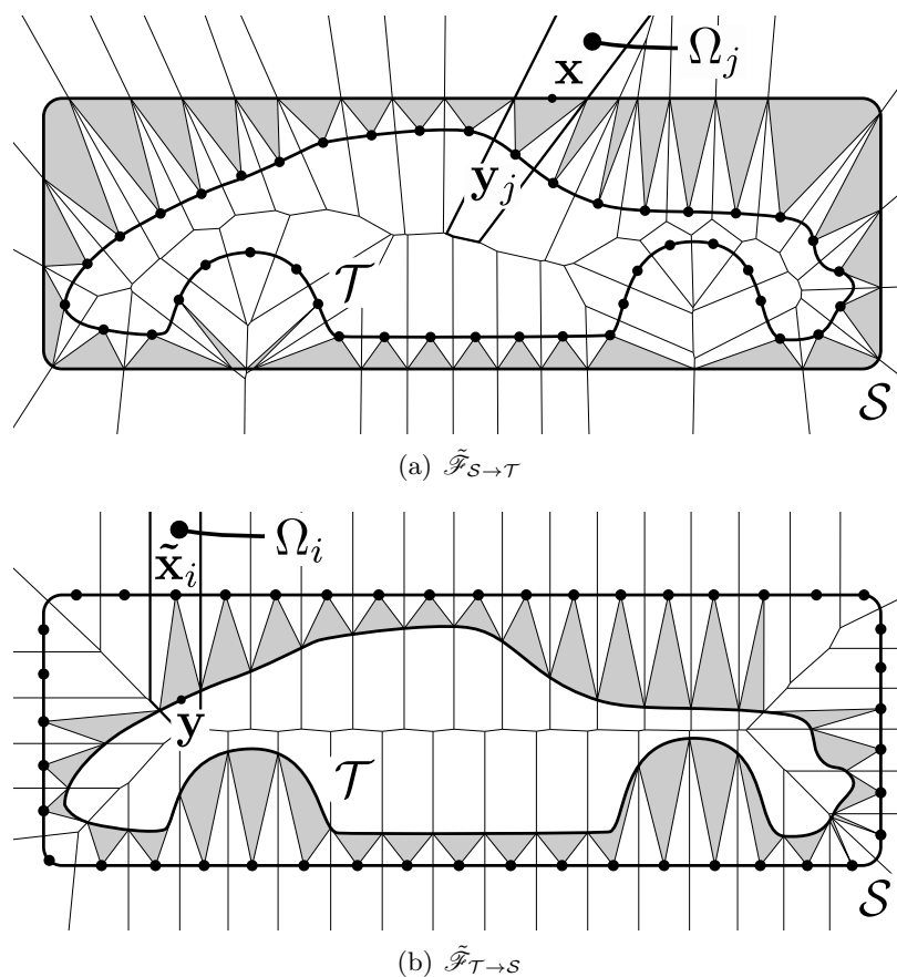
FIGURE 5.5 – Distance au carré de Voronoï. Les régions grisées représentent, pour chaque échantillon \tilde{\mathbf{x}}_i (resp. \tilde{\mathbf{y}}_j ) la portion de \mathcal{T} (resp. \mathcal{S} ) pour laquelle \tilde{\mathbf{x}}_i sera le plus proche.
