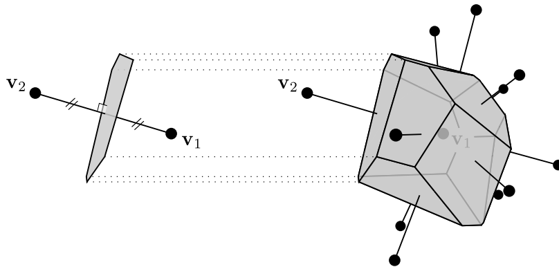
FIGURE 3.6 – Cellule de Voronoï dans \mathbb{R}^3 . Dans ce cas, les cellules sont des polyèdres dont chaque face est le plan bissecteur d'une paire de sites. Étant donnés deux sites v_1 et v_2 , leur plan bissecteur est le plan perpendiculaire au segment [v_1, v_2] , passant par son milieu.
