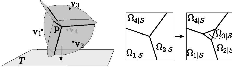
FIGURE 4.7 – Changement de combinatoire lorsqu'un sommet de Voronoï \mathbf{p} traverse une face T de \mathcal{S} . Lorsque \mathbf{p} est au dessus de T , seules les cellules de Voronoï des sites \mathbf{v}_1 , \mathbf{v}_2 et \mathbf{v}_4 intersectent T . Lorsque \mathbf{p} passe en dessous de \mathcal{S} , la cellule de Voronoï de \mathbf{v}_3 intersecte également T , ce qui modifie la combinatoire du diagramme de Voronoï restreint à l'intérieur de T .
