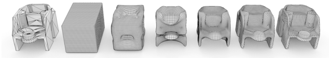
FIGURE 4 – Ajustement de deux surfaces. La surface cible est la pièce mécanique de gauche, et la surface ajustée est le pavé. De gauche à droite, le pavé est déformé pour s'ajuster au maillage cible.
