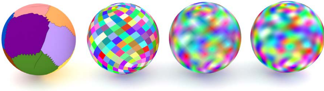
FIGURE 2.16 – Placage sans couture visible pour différents modes de filtrages. De gauche à droite, les différentes cartes et les filtrages au plus proche bilinéaire et bicubique. Ici, la paramétrisation contient quatre singularités d'indice \frac{2}{2} visibles en haut et en bas de la sphère, en particulier sur le filtrage au plus proche. Aucune couture n'est apparente, même autour des singularités.
