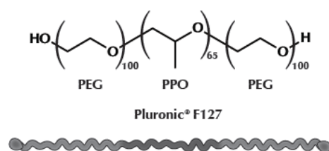
Figure 25 : Structure moléculaire du Pluronic® F127
