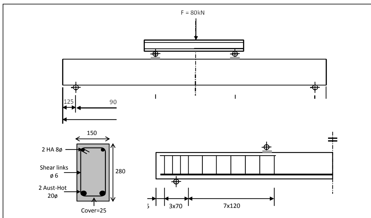
Fig. RE5 Dimension en mm des poutres en béton armé
