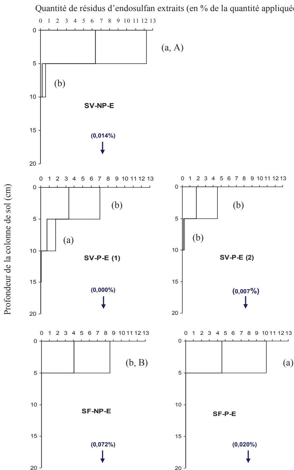
Figure 5-7 : Répartition des quantités totales d'endosulfan \beta (□) et d'endosulfan sulfate (▨) dans les profils de sols verticale (SV) et ferrugineux (SF) non planté (NP) et planté au vétiver (P) 6 mois après le traitement. Les quantités d'endosulfan lessivées sont données (entre parenthèses). L'endosulfan \alpha n'est détecté dans aucun des sols ( < 0,03 \text{ mg kg}^{-1} ). Pour chaque horizon, la différence entre les colonnes est évaluée par le test F de Fisher (intervalle de confiance de 95%). Les différences significatives sont indiquées par des lettres (a, b) pour le même sol (entre planté et non planté) et par des lettres en MAJUSCULES (A, B) pour les deux sols de nature différente (SV-NP et SF-NP).
