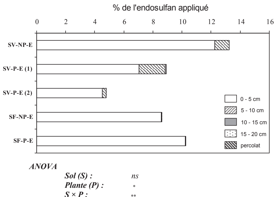
Figure 5-8: Bilan de masse des résidus d'endosulfan dans les colonnes de sols vertique (SV) et ferrugineux (SF), non plantés (NP) et plantés au vétiver (P), ayant reçu de l'endosulfan (E), et dans les percolats (en % de la quantité appliquée).
