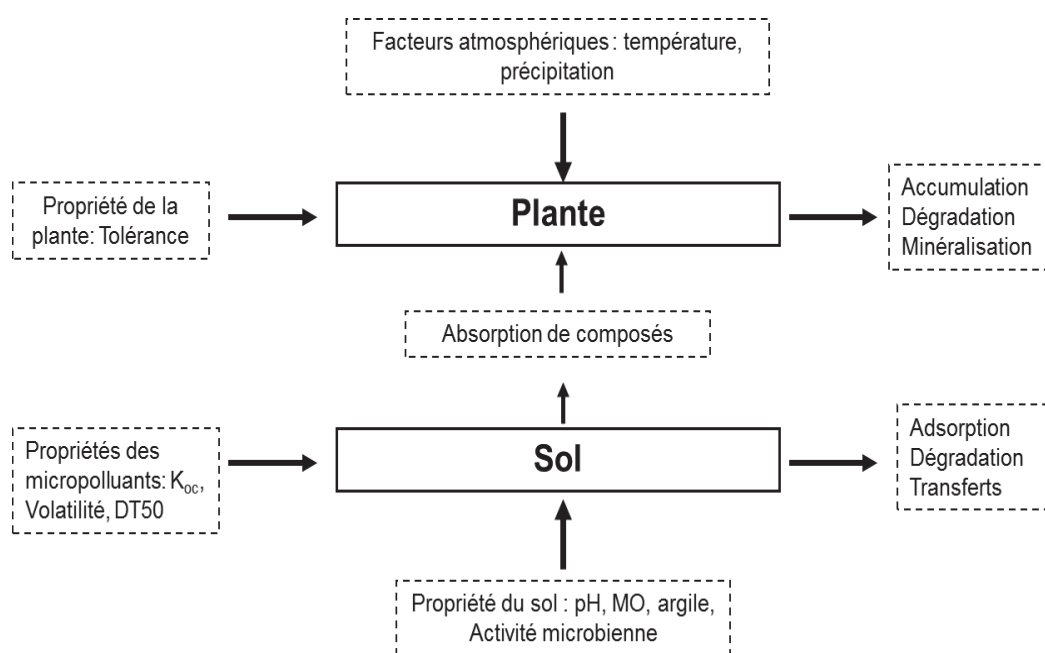
Figure 1- 5 : Dynamique des polluants organiques et métalliques dans le système sol-plante, influence des différents facteurs impliqués ; MO : matière organique.
