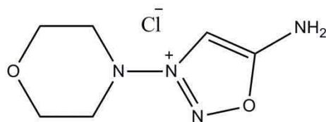
Linsidomine
