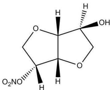
(5-) Mononitrate d'isosorbide
