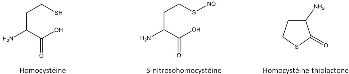
Figure 10 : Structures de l'homocystéine, de la S-nitrosohomocystéine et de l'homocystéine thiolactone
