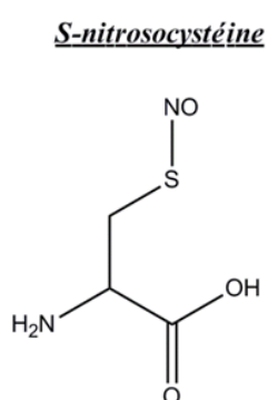
Figure 8 : Structures du S -nitrosoglutathion, de la S -nitrosocystéine et de la S -nitrosocystéinyglycine
