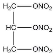
Trinitrine
