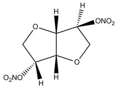
Dinitrate d'isosorbide
