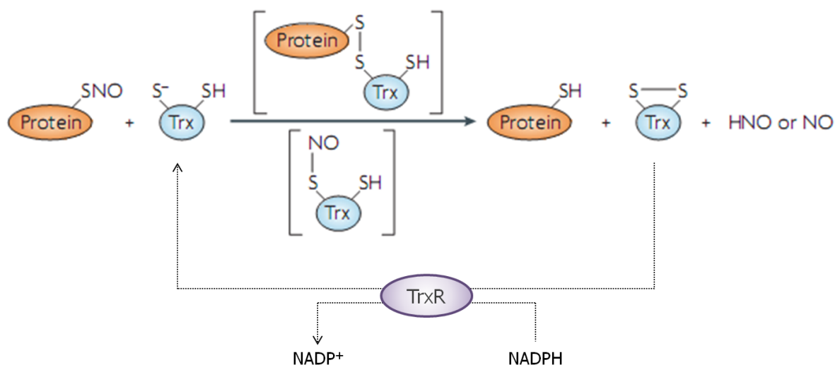
Figure 18 : Schéma de la réaction d'un S-nitrosothiol avec la thiorédoxine, exemple d'un S-nitrosothiol protéique. Modifié d'après [238].
