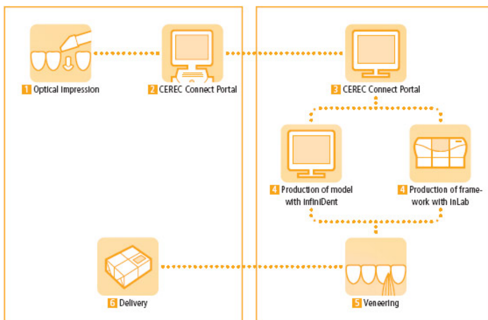
Figure 57 : Chaîne CEREC CFAO Semi direct ( www.sirona.fr )
