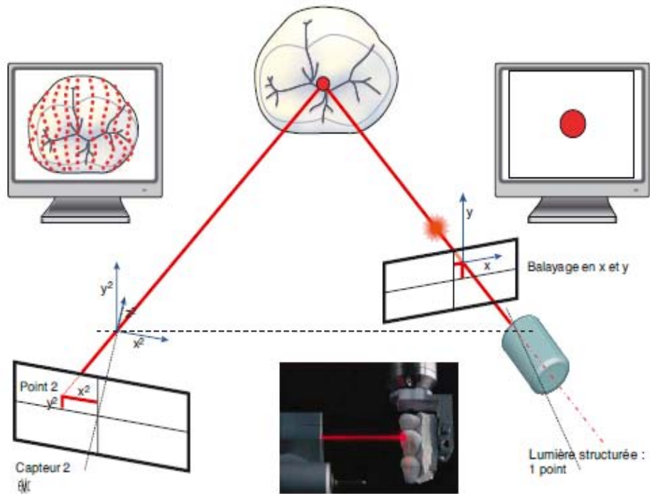
Figure 2 : Schéma de la méthode de mesure par projection d'un point en triangulation par lumière structurée.(3)
