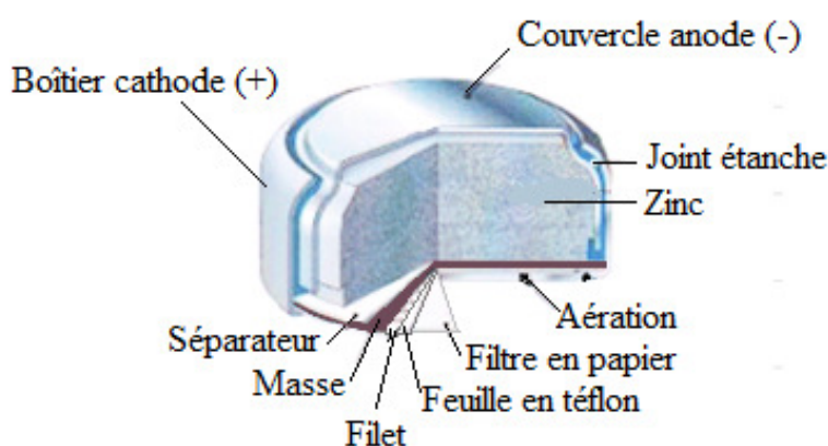
Figure 6 : Composants d'une pile zinc-air [11]
